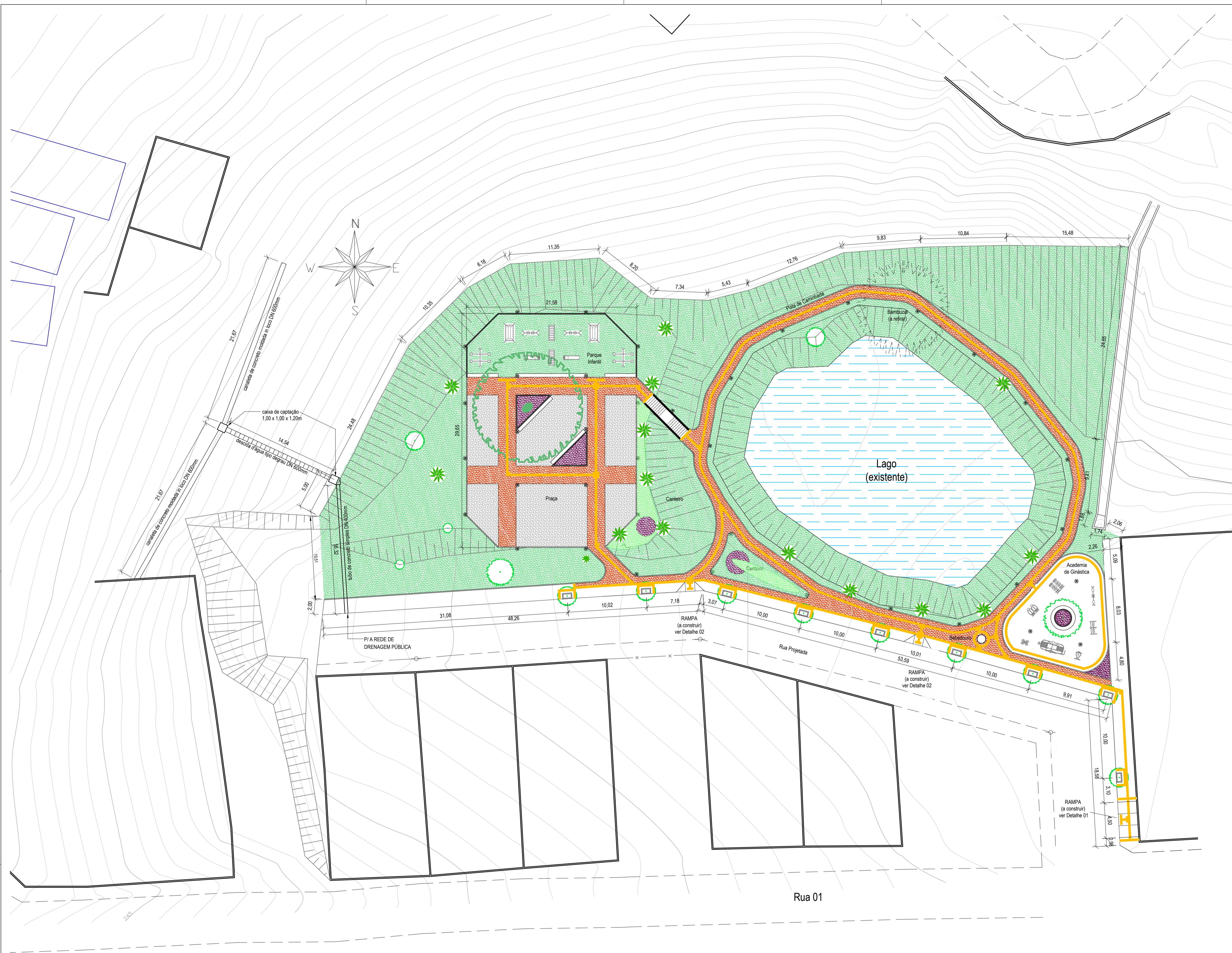
PLANTA DE SITUAÇÃO ESC: 1/250
