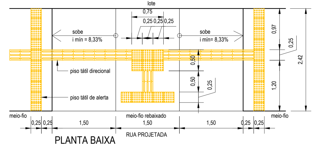
PLANTA BAIXA RUA PROJETADA VISTA meio-fio meio-fio rebaixado max 0.10
