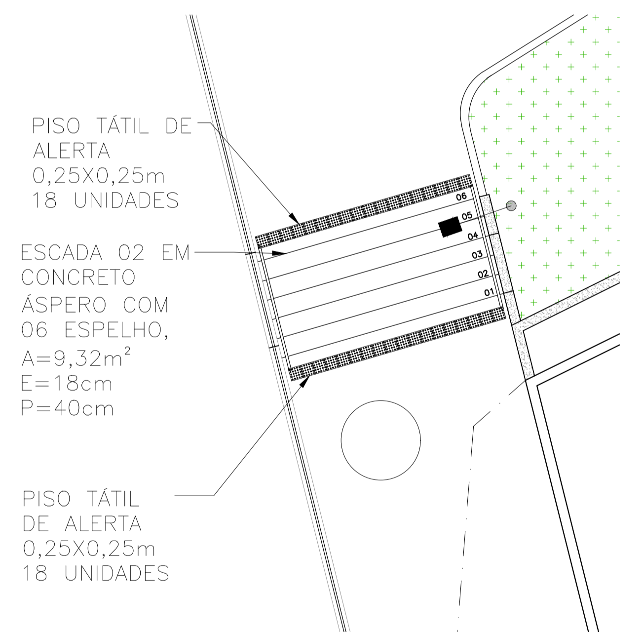
DETALHE 02 - ACESSIBILIDADE - ESCADA 02 ESC 1:75
