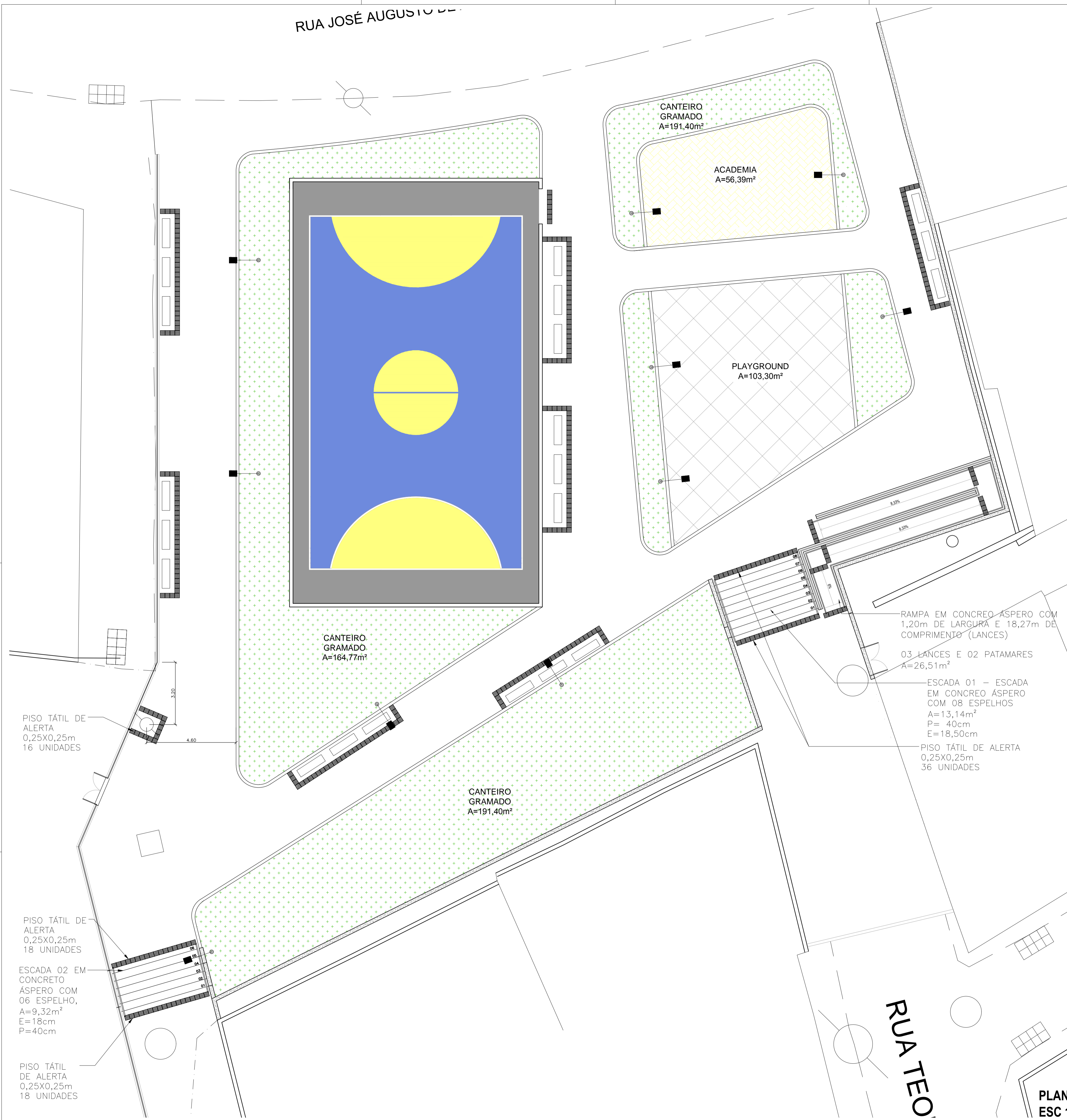
DETALHE 01 - ACESSIBILIDADE - ESCADA E RAMPA 01 ESC 1:75
