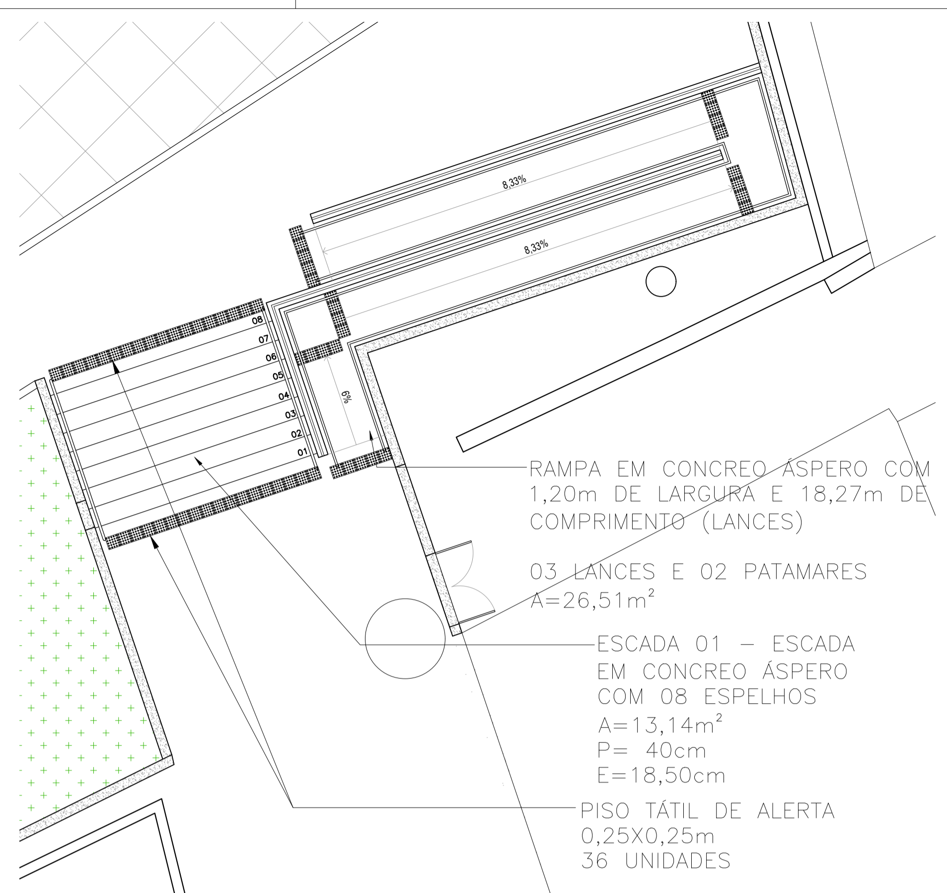
DETALHE 01 - ACESSIBILIDADE - ESCADA E RAMPA 01 ESC 1:75
