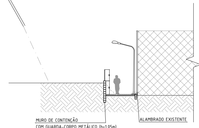
CORTE AA ESC 1:200
