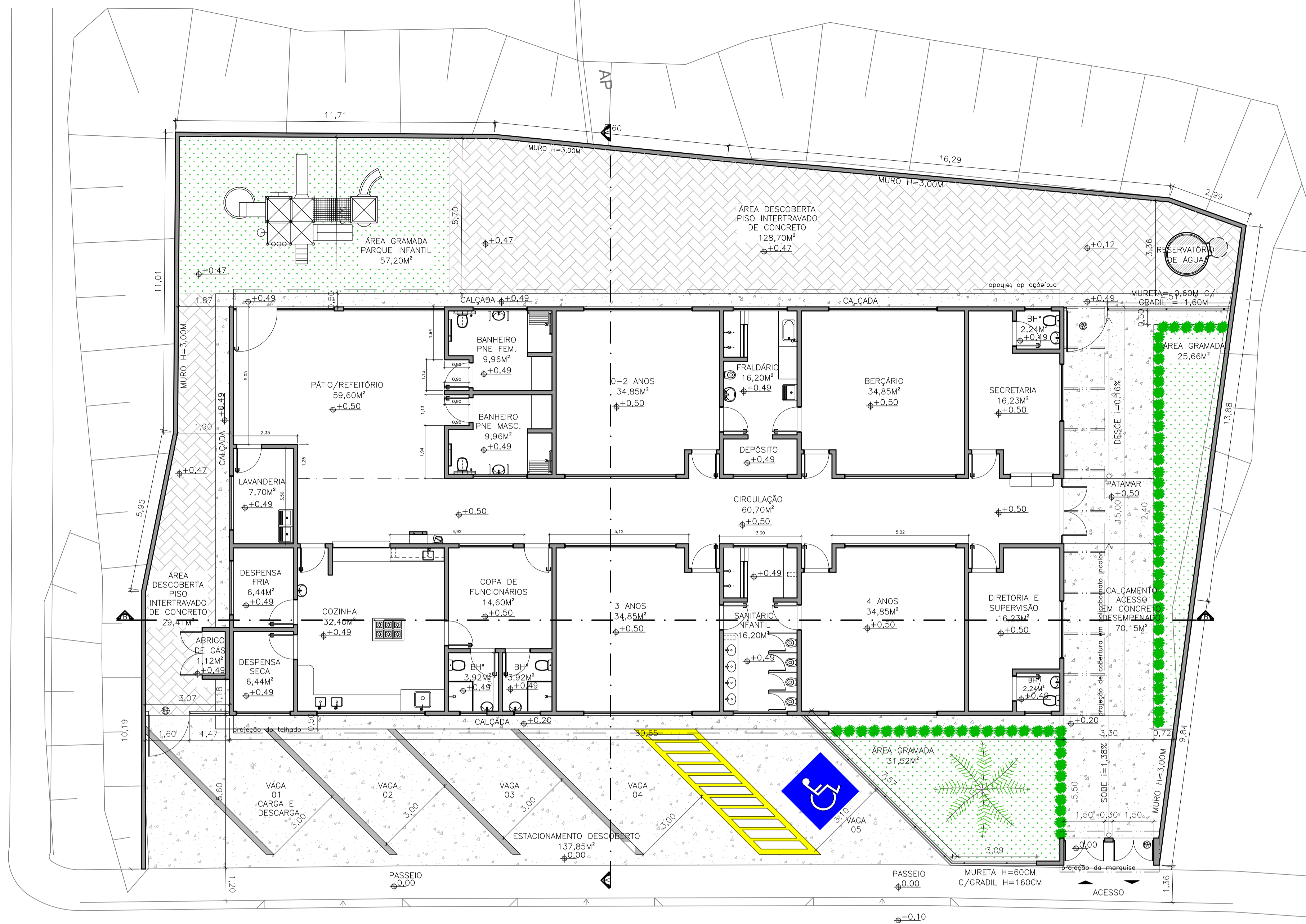
PLANTA DE IMPLANTAÇÃO ESC.: 1 / 100
