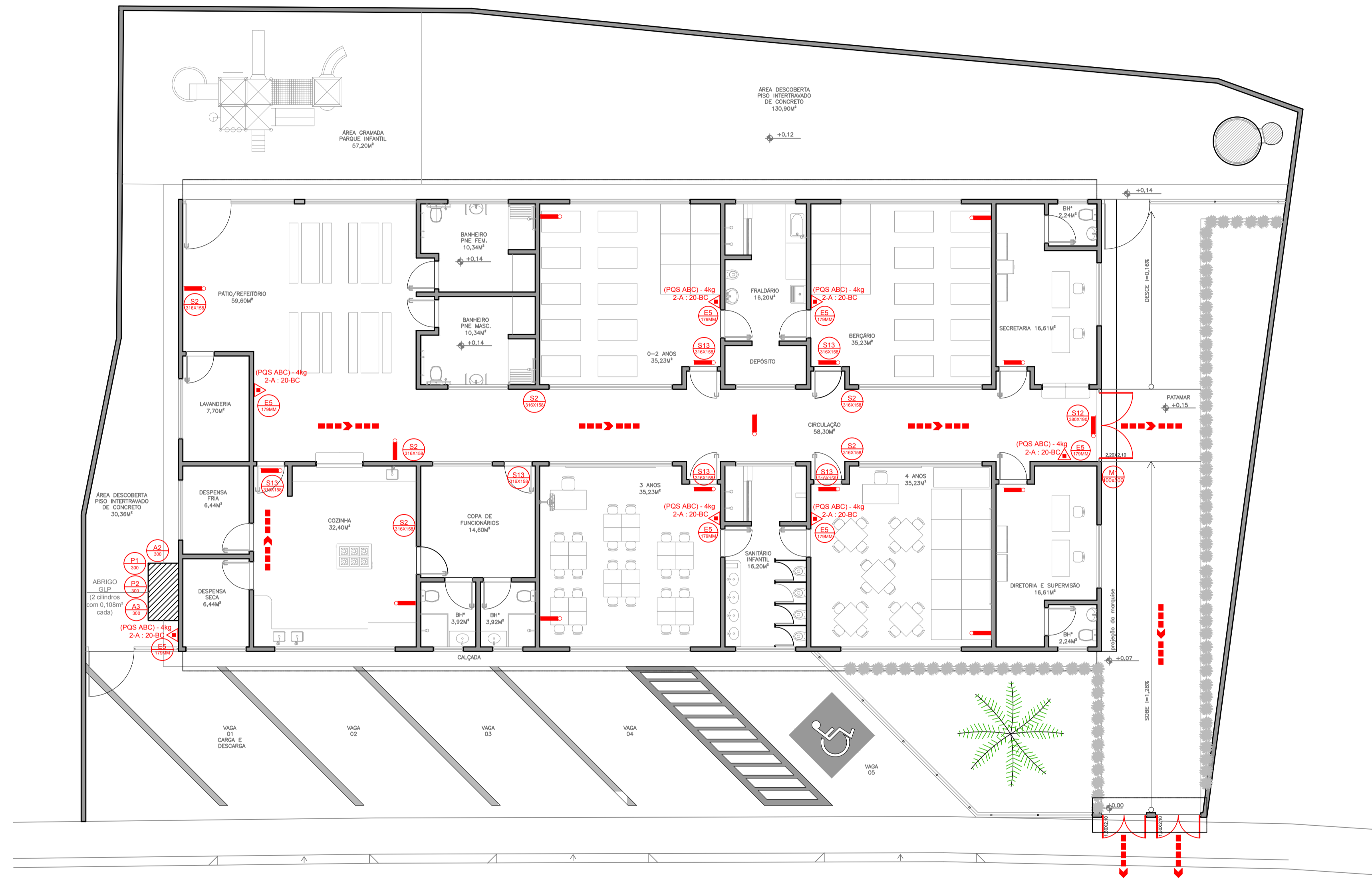
PLANTA BAIXA - INCÊNDIO ESCALA 1:100
