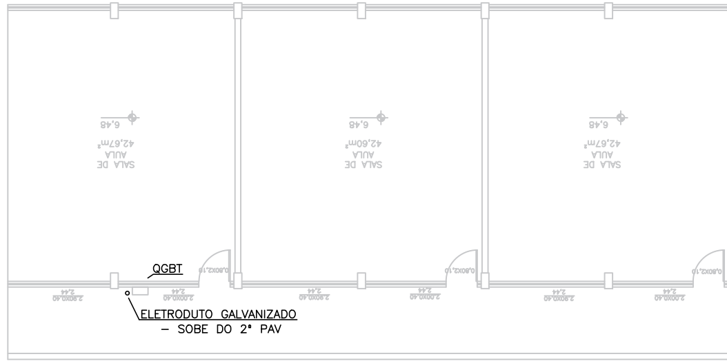
PLANTA BAIXA - 3º PAVIMENTO
