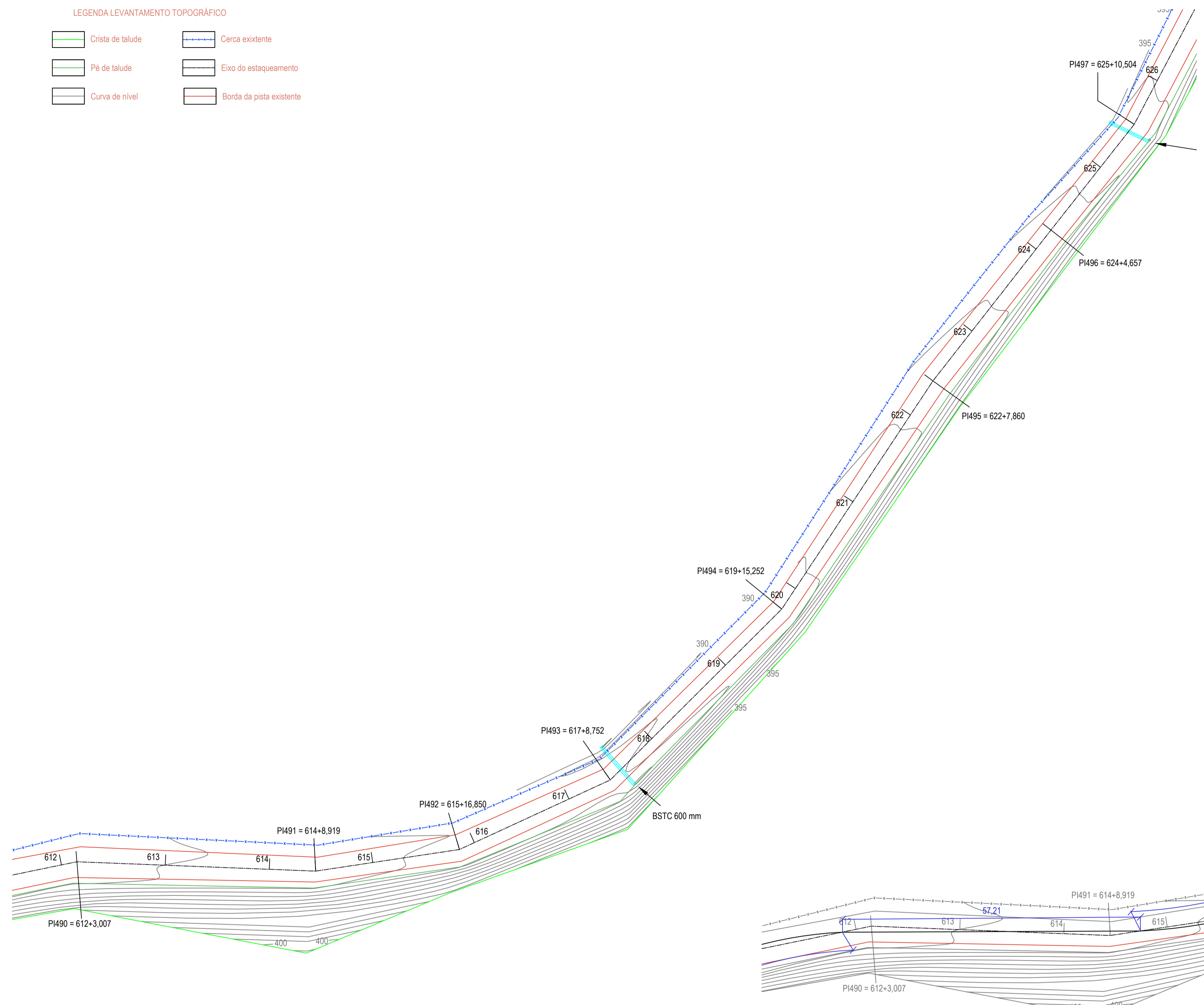
LEVANTAMENTO TOPOGRÁFICO PLANIATIMÉTRICO - TRECHO C-C ESC: 1/500
