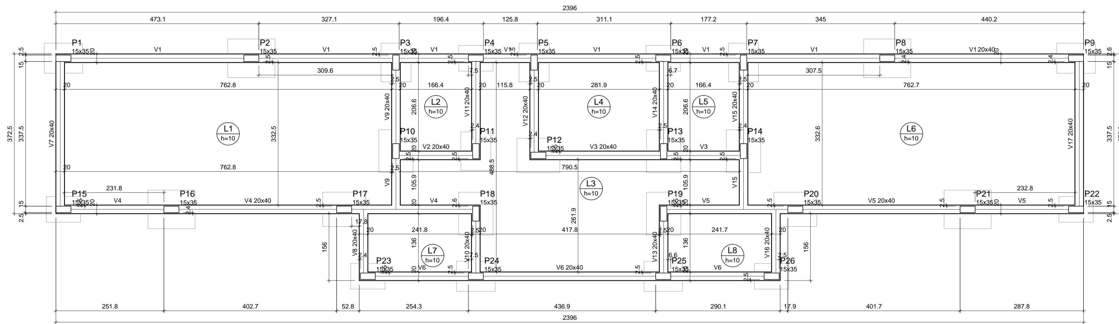
Forma do Pavimento Fundação (Nível 0) escala 1:50
