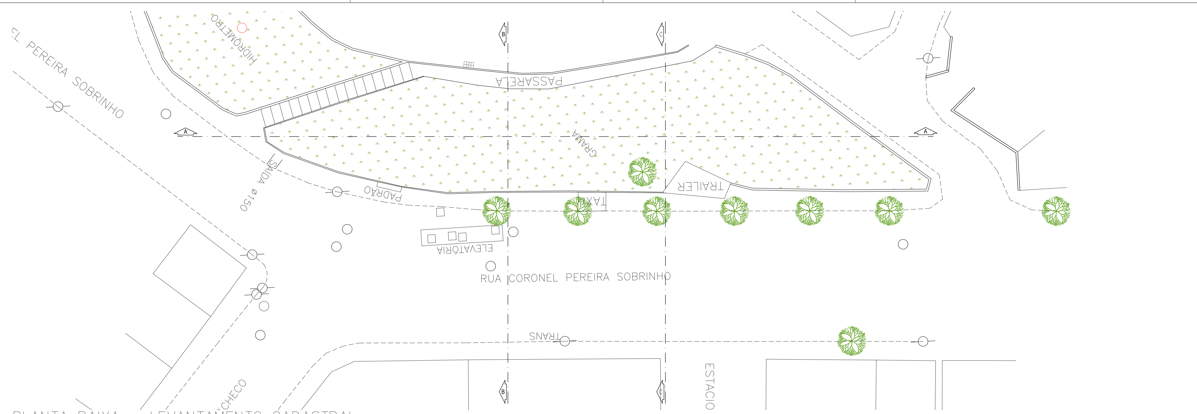
PLANTA BAIXA - LEVANTAMENTO CADASTRAL ESC: 1:100
