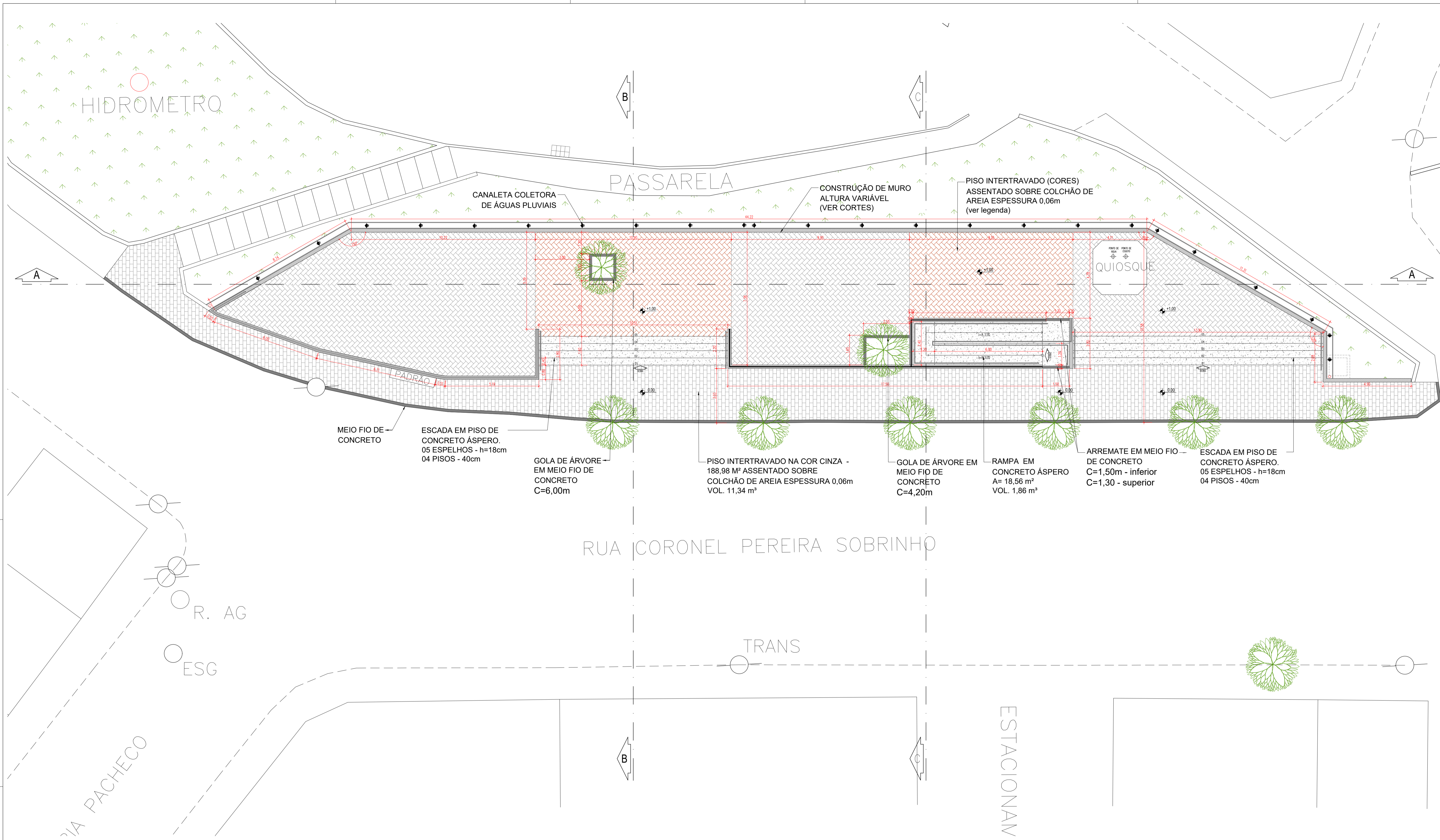
PLANTA BAIXA - CONSTRUÇÃO E PISOS ESC: 1:100
