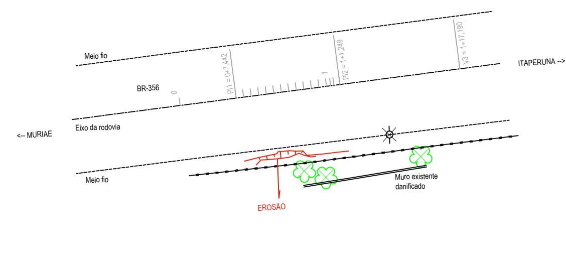
LEVANTAMENTO TOPOGRÁFICO PLANIATIMÉTRICO ESC: 1/500
