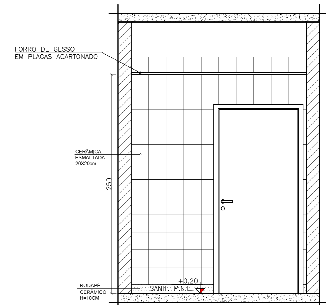
AMPLIAÇÃO 02 - BANHEIRO MASC. VISTA 03 ESCALA: 1/25
