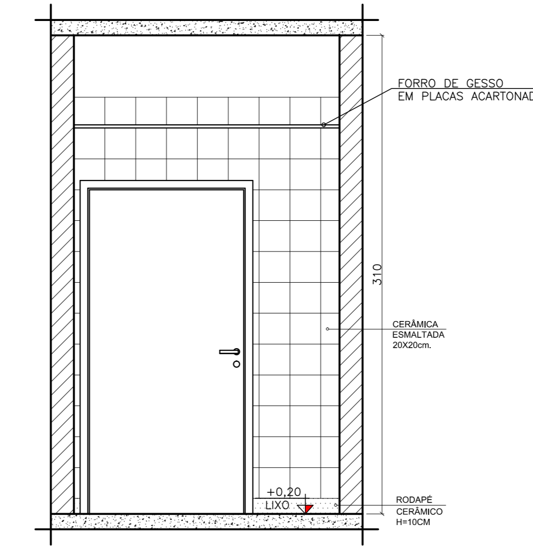
AMPLIAÇÃO 01 - LIXO VISTA 04 ESCALA: 1/25
