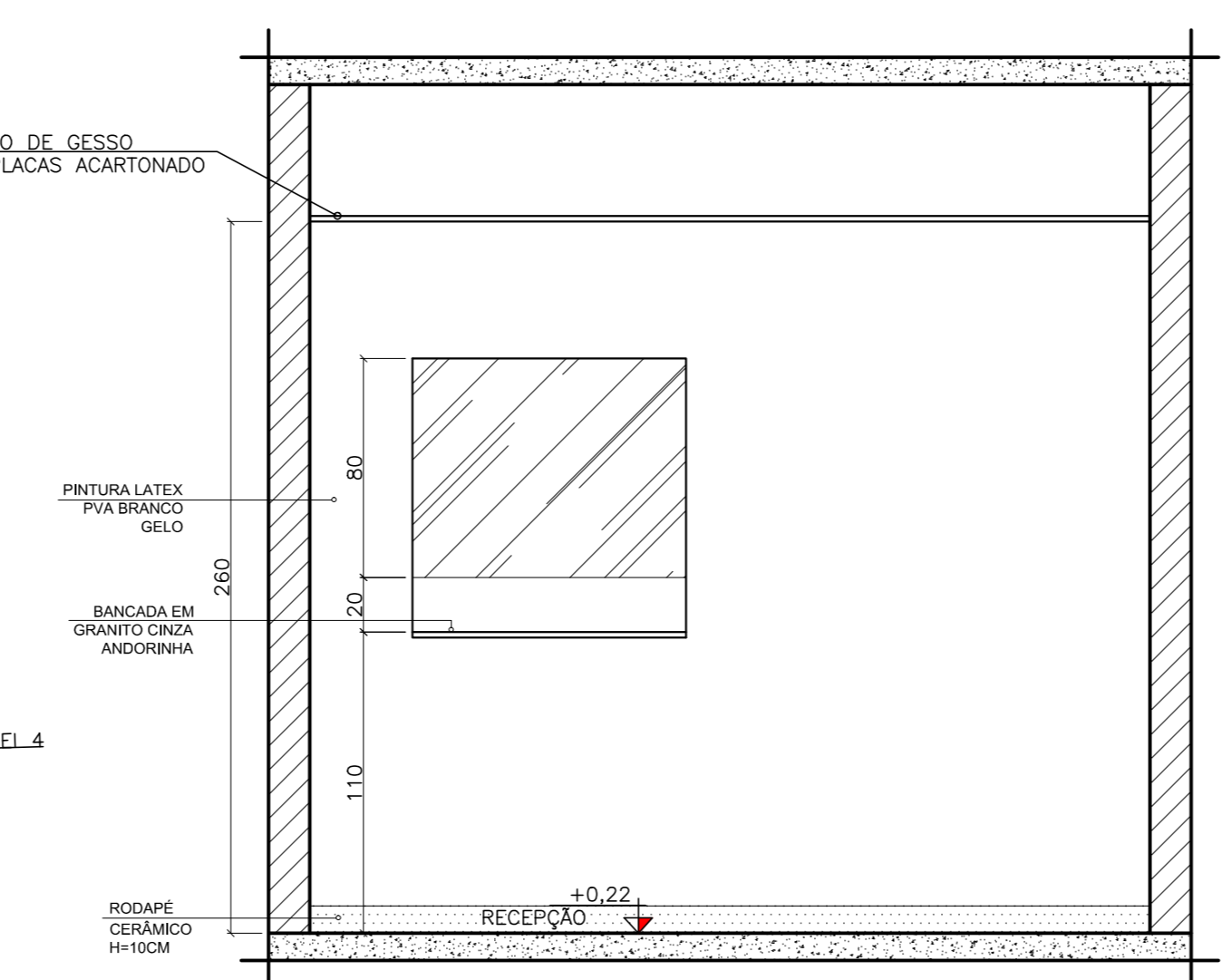
AMPLIAÇÃO 05 - RECEPÇÃO VISTA 01 ESCALA: 1/25
