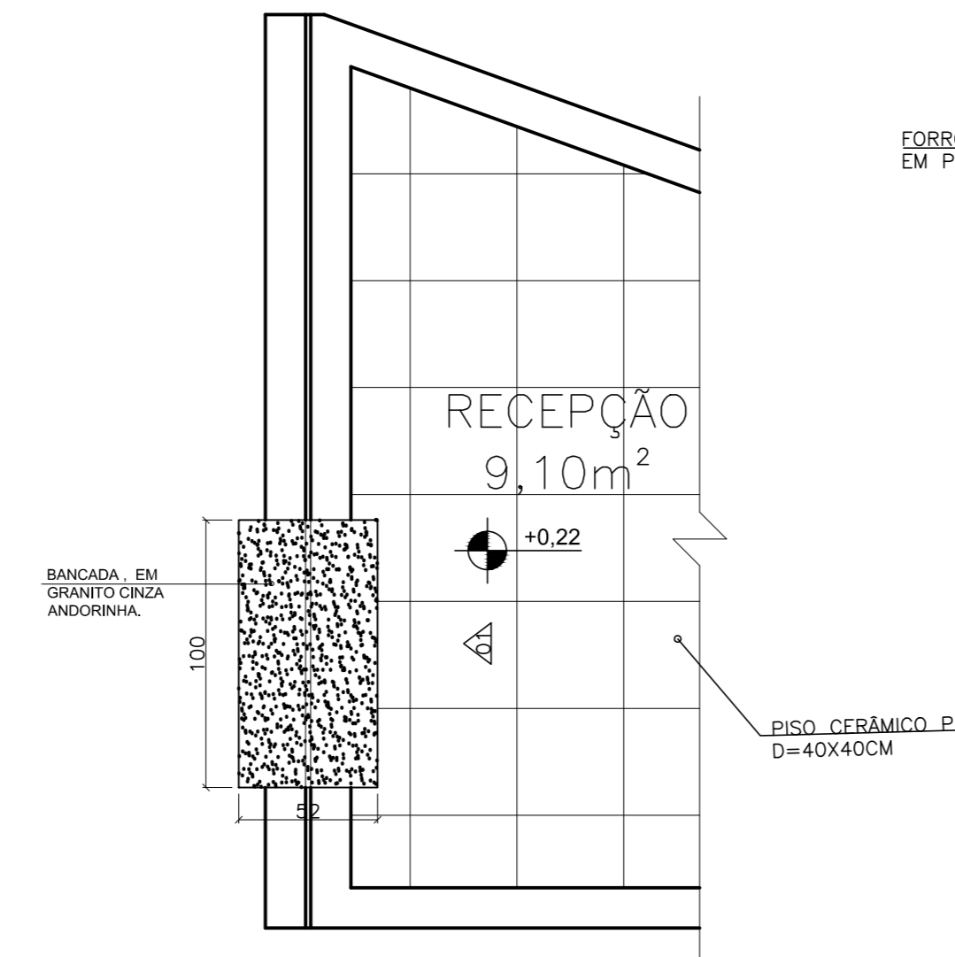
AMPLIAÇÃO 05 - RECEPÇÃO PLANTA ESCALA: 1/25
