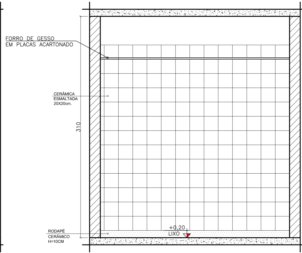
AMPLIAÇÃO 01 - LIXO VISTA 02 ESCALA: 1/25
