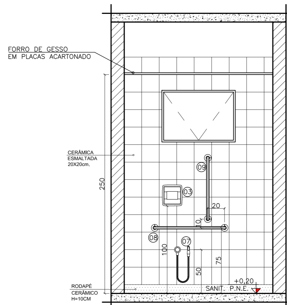
AMPLIAÇÃO 02 - BANHEIRO MASC. VISTA 02 ESCALA: 1/25
