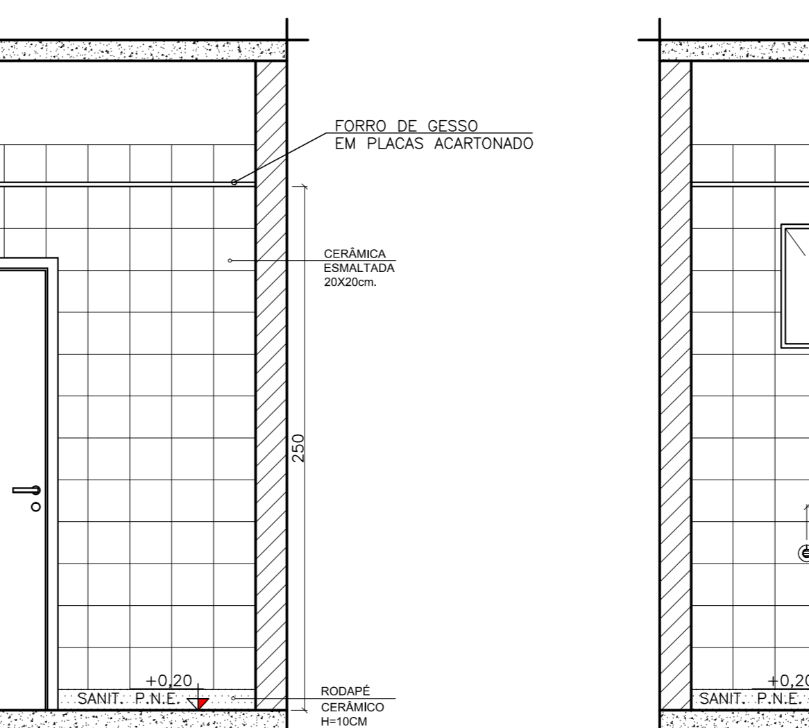
AMPLIAÇÃO 02 - BANHEIRO FEM. VISTA 04 ESCALA: 1/25
