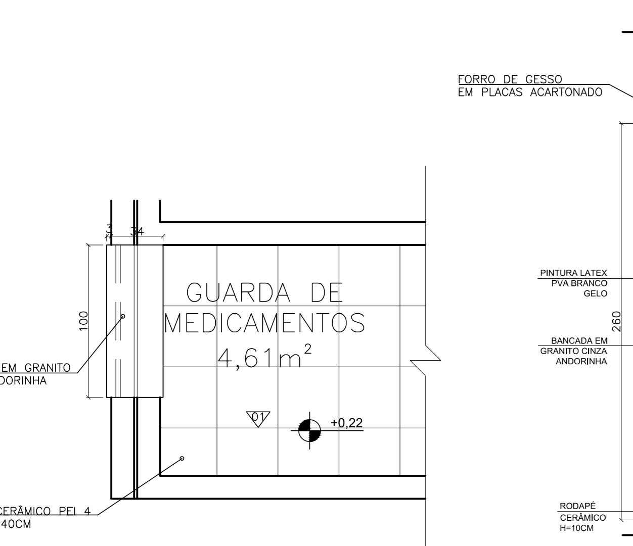
AMPLIAÇÃO 04 - GUARDA DE MEDICAMENTOS PLANTA ESCALA: 1/25
