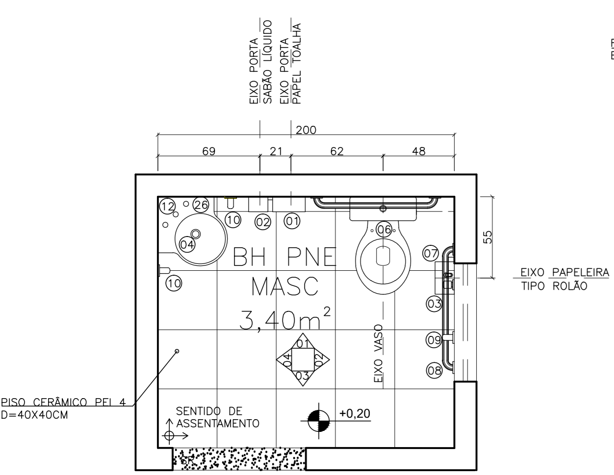
AMPLIAÇÃO 02 - BANHEIRO MASC. PLANTA ESCALA: 1/25
