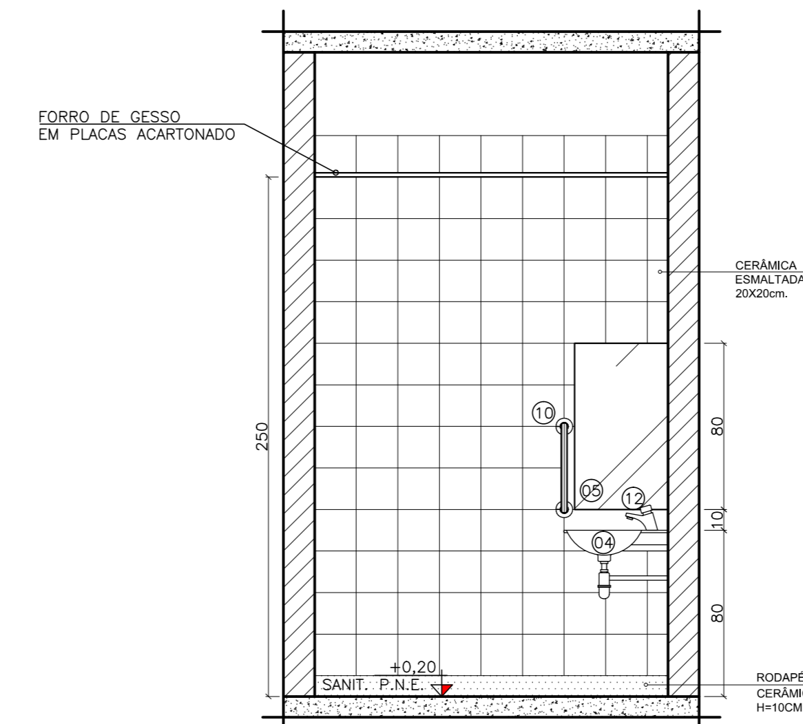
AMPLIAÇÃO 02 - BANHEIRO MASC. VISTA 04 ESCALA: 1/25
