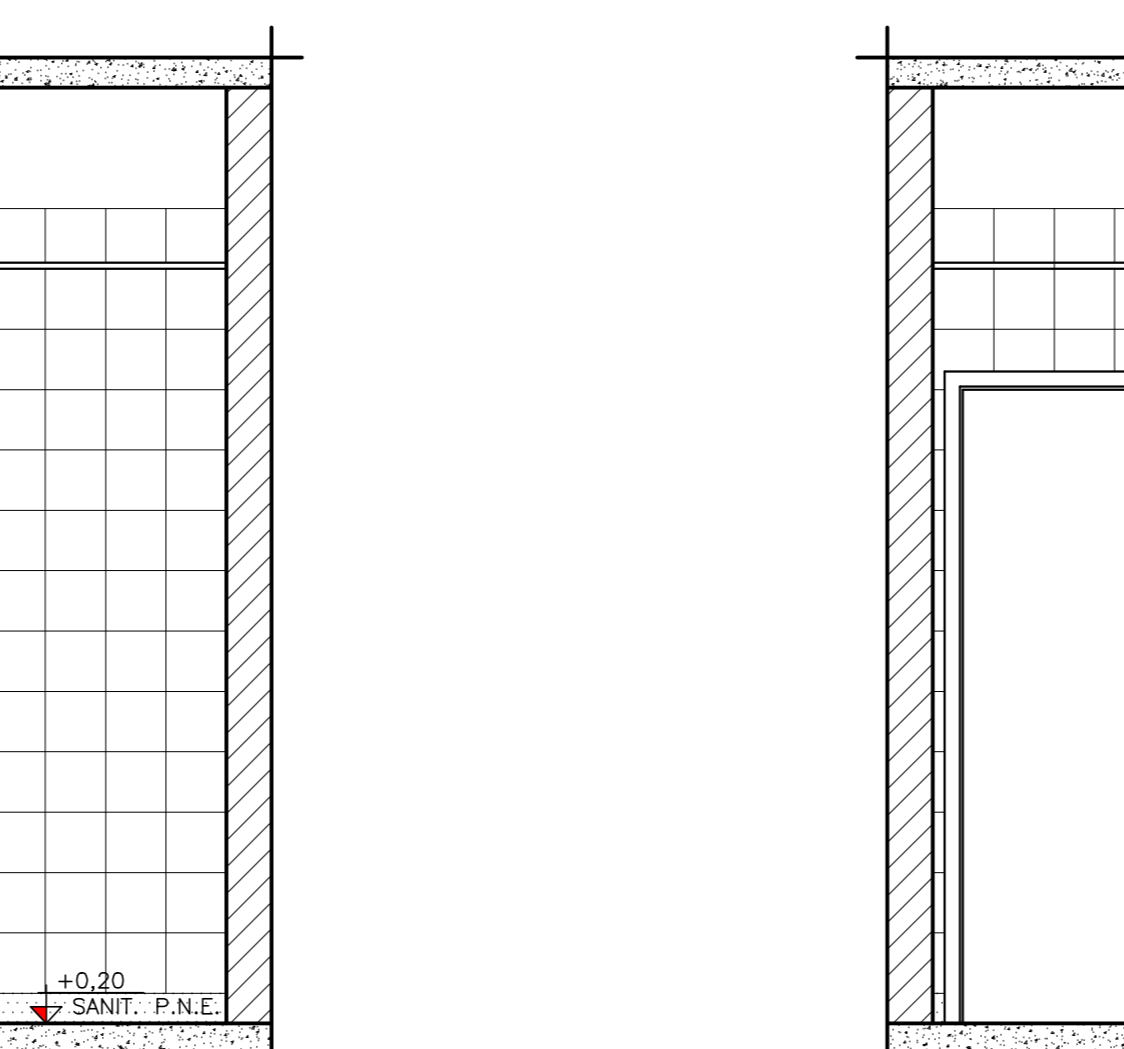
AMPLIAÇÃO 03 - BANHEIRO FEM. VISTA 03 ESCALA: 1/25
