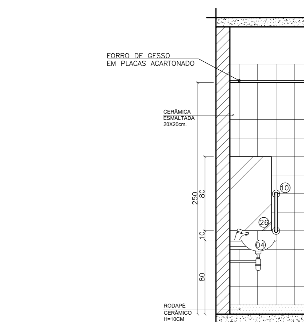
AMPLIAÇÃO 03 - BANHEIRO FEM. VISTA 02 ESCALA: 1/25
