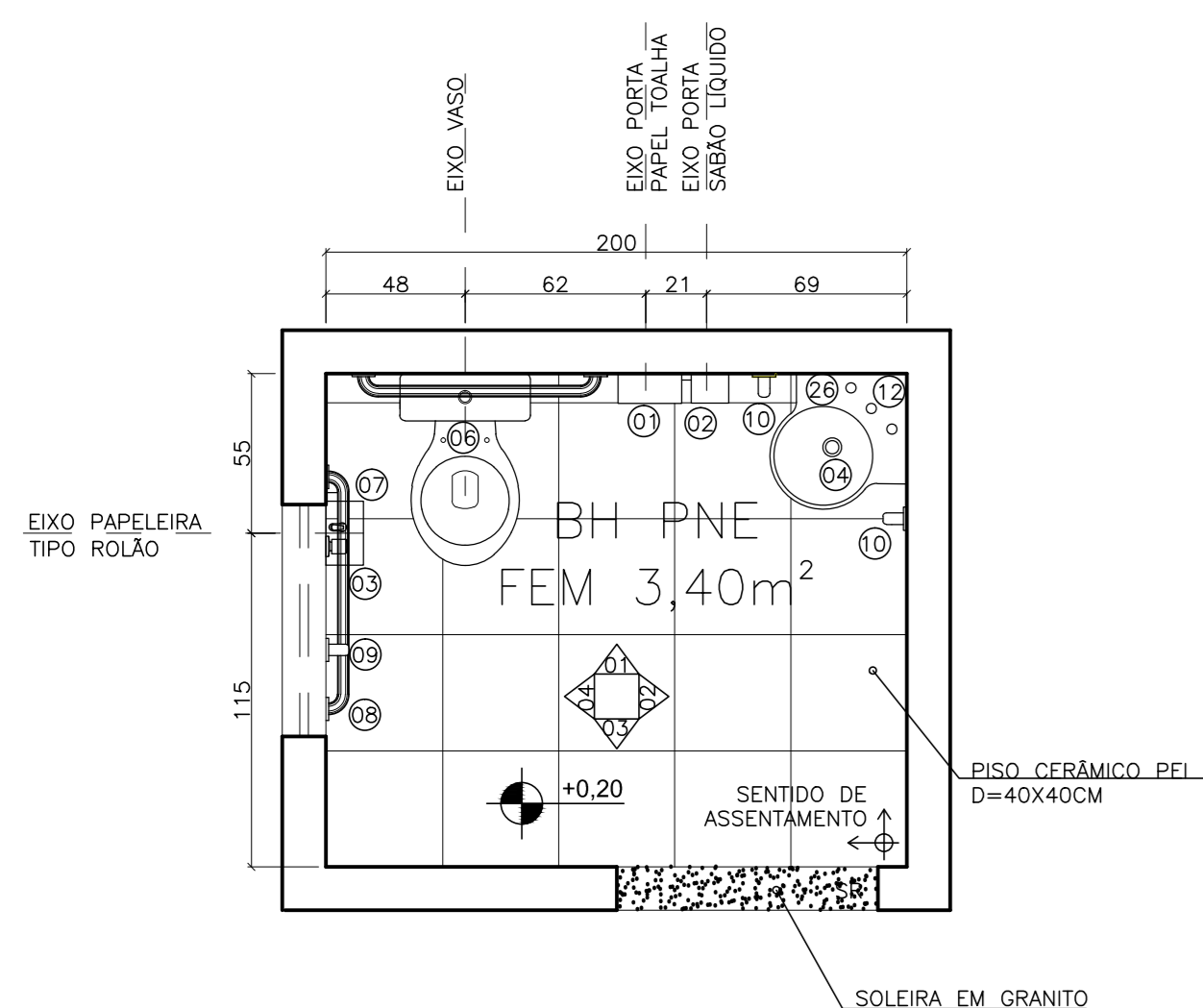
AMPLIAÇÃO 03 - BANHEIRO FEM. PLANTA ESCALA: 1/25
