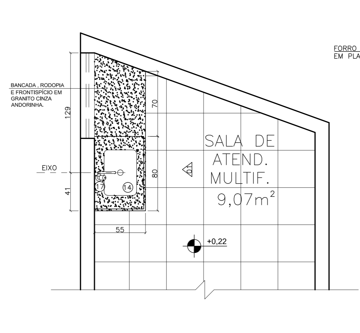
AMPLIAÇÃO 06 - ATEND. MULTIFUNCIONAL PLANTA ESCALA: 1/25
