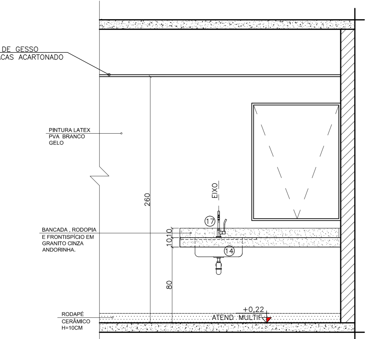
AMPLIAÇÃO 06 - ATEND. MULTIFUNCIONAL VISTA 01 ESCALA: 1/25
