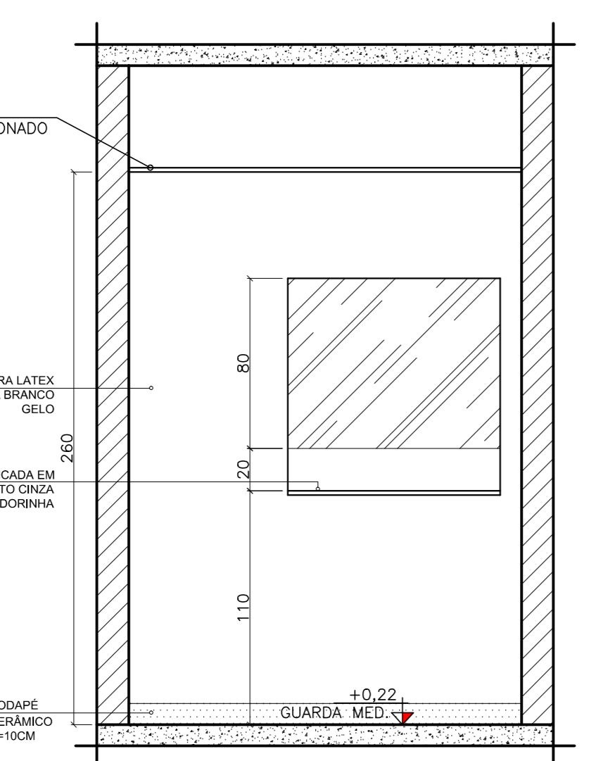
AMPLIAÇÃO 04 - GUARDA DE MEDICAMENTOS VISTA 01 ESCALA: 1/25
