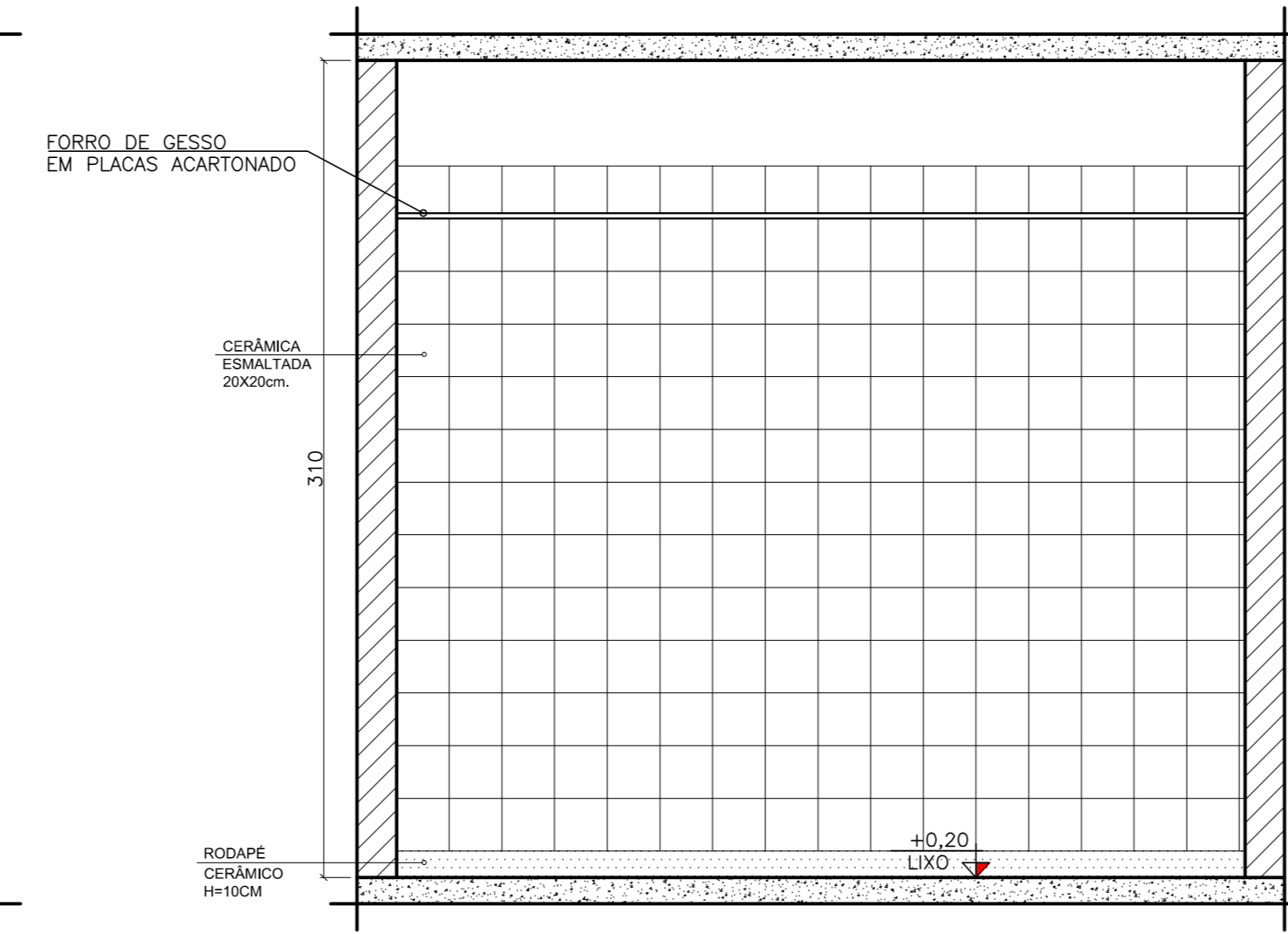
AMPLIAÇÃO 01 - LIXO VISTA 03 ESCALA: 1/25
