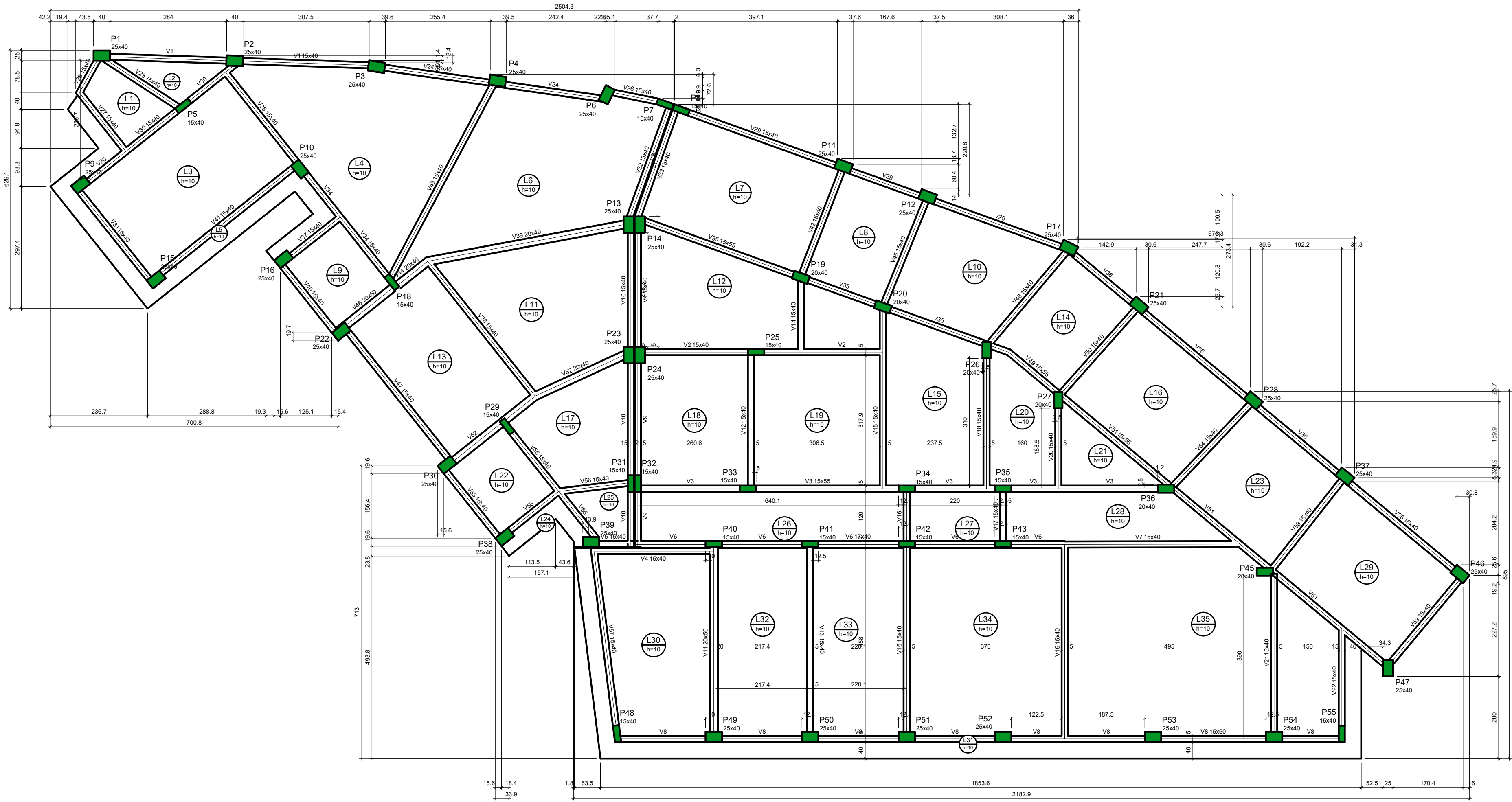
Forma do pavimento 1º Pavimento (Nível 664)
