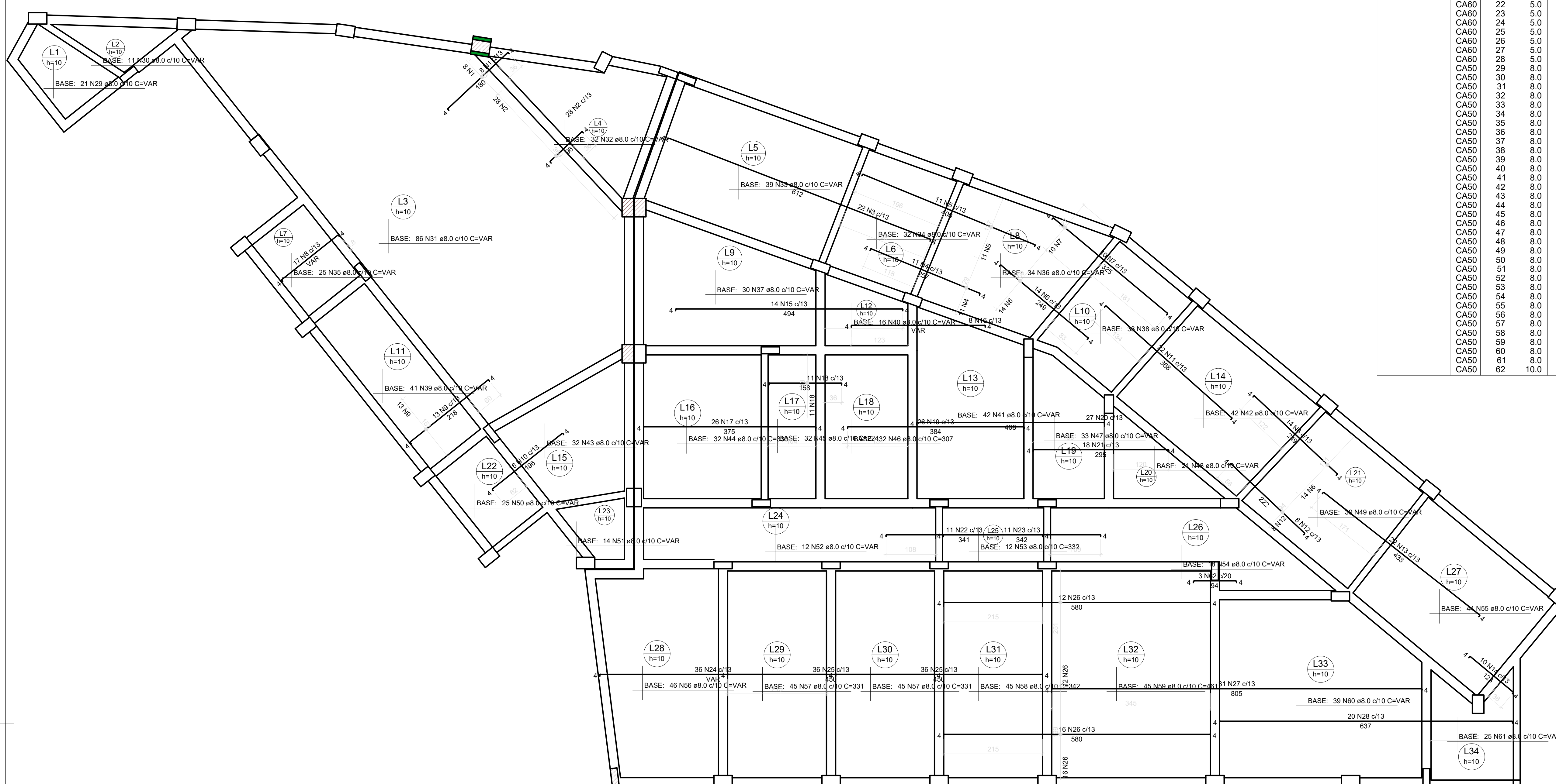
Armação Superior do Radier Pavimento Fundação (Eixo X) escala 1:50
