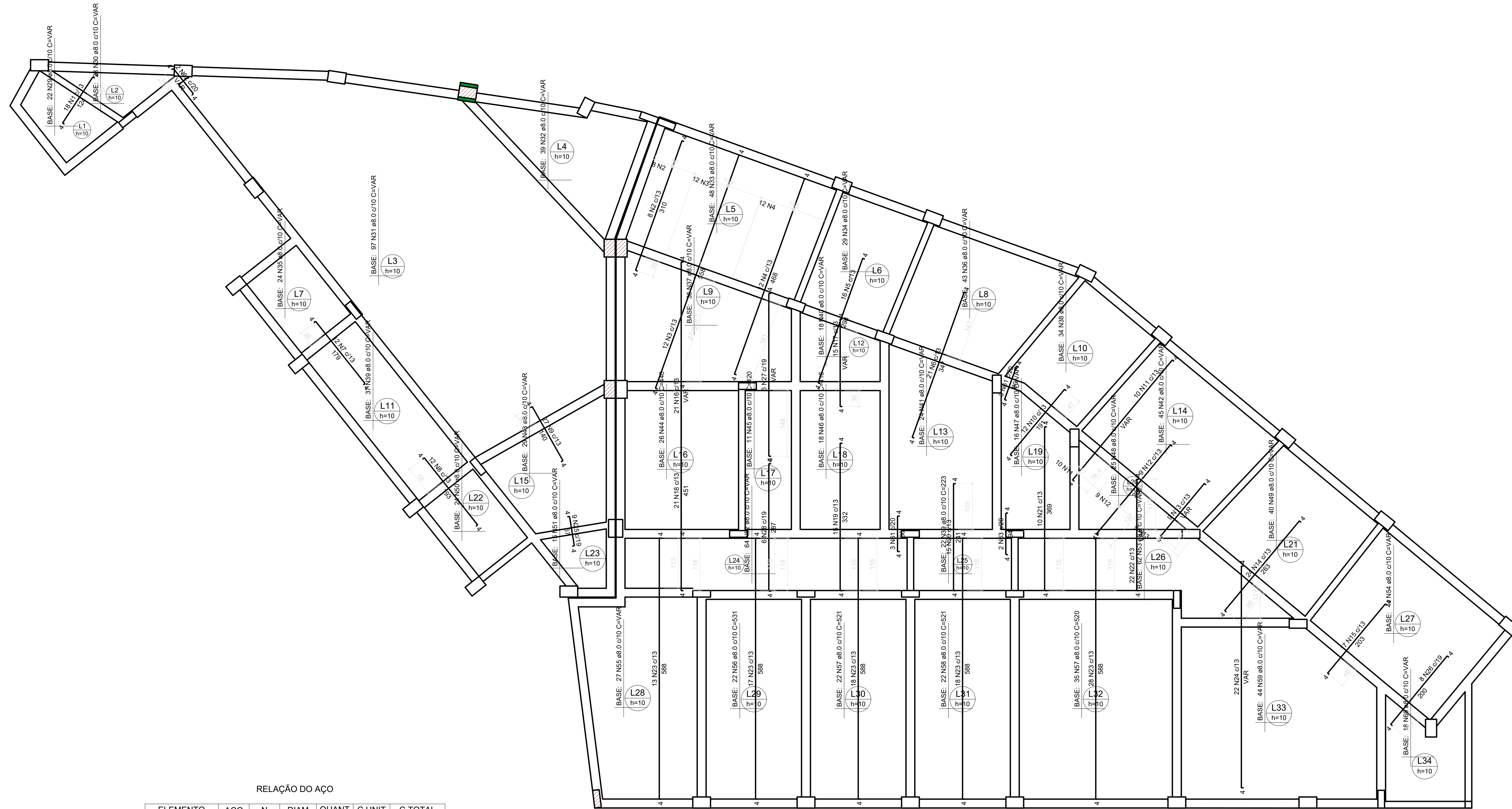
Armação Superior do Radier Pavimento Fundação (Eixo Y) escala 1:50
