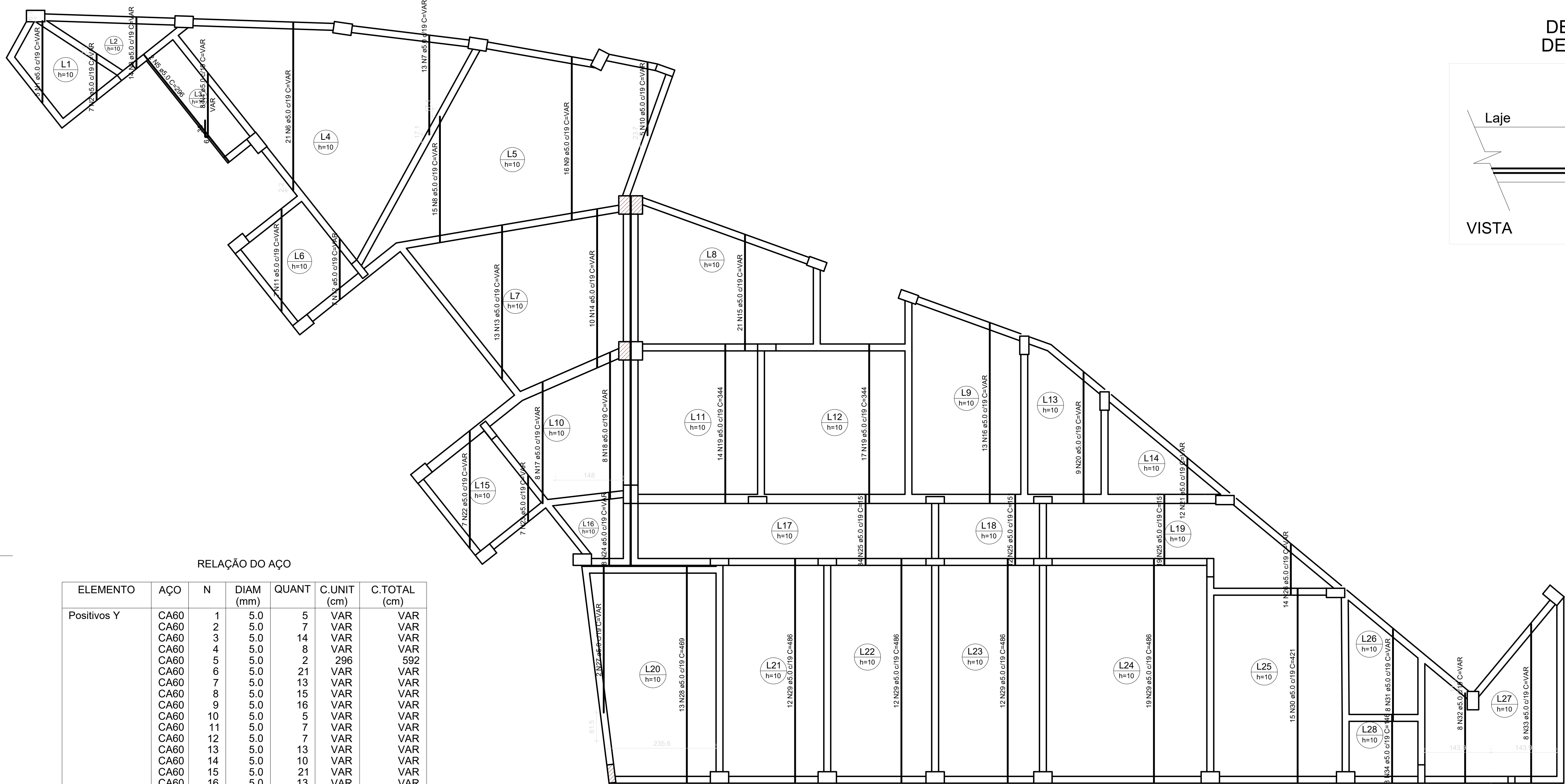
Armação Positiva das Lajes Pavimento Terreo (Eixo Y) escala 1:50
