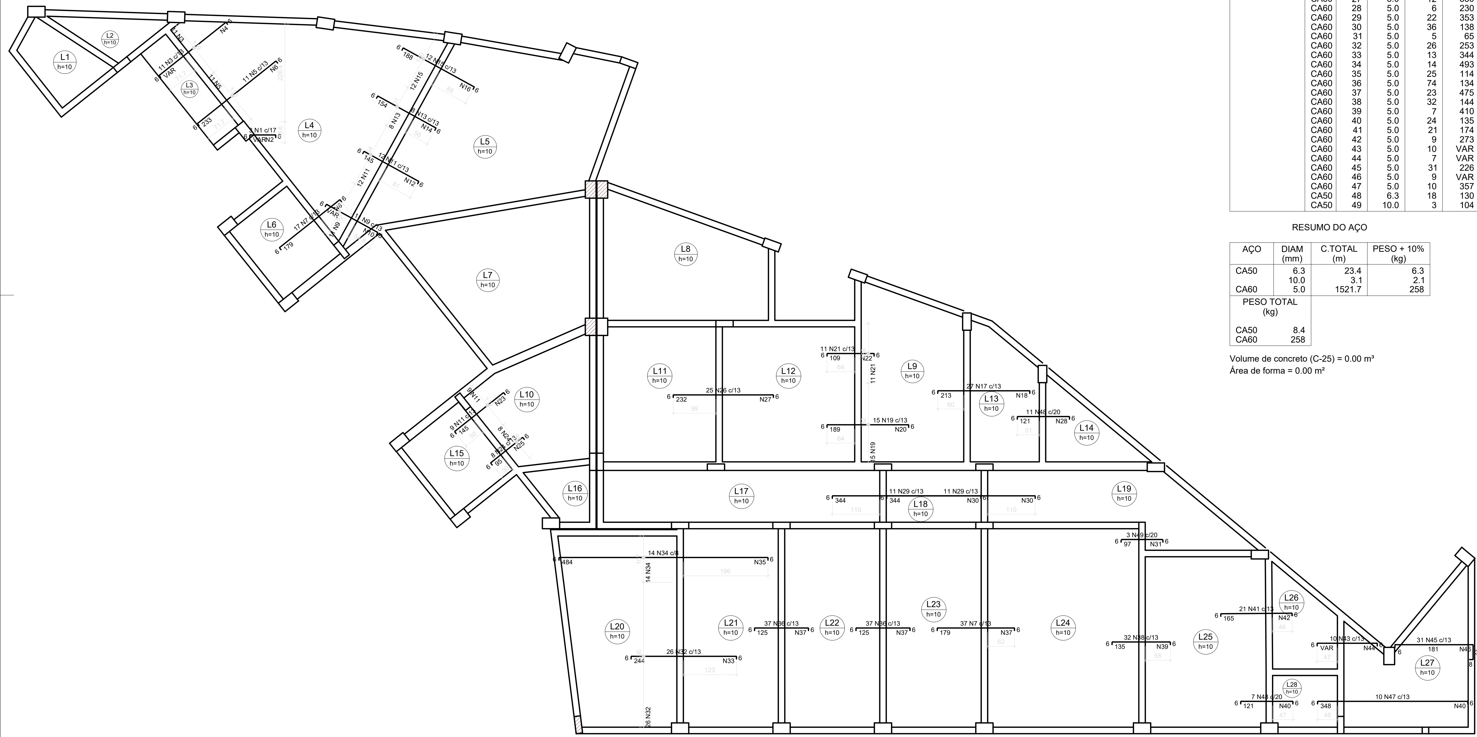
Armação Negativa da Laje Pavimento Terreo (Eixo X) escala 1:50
