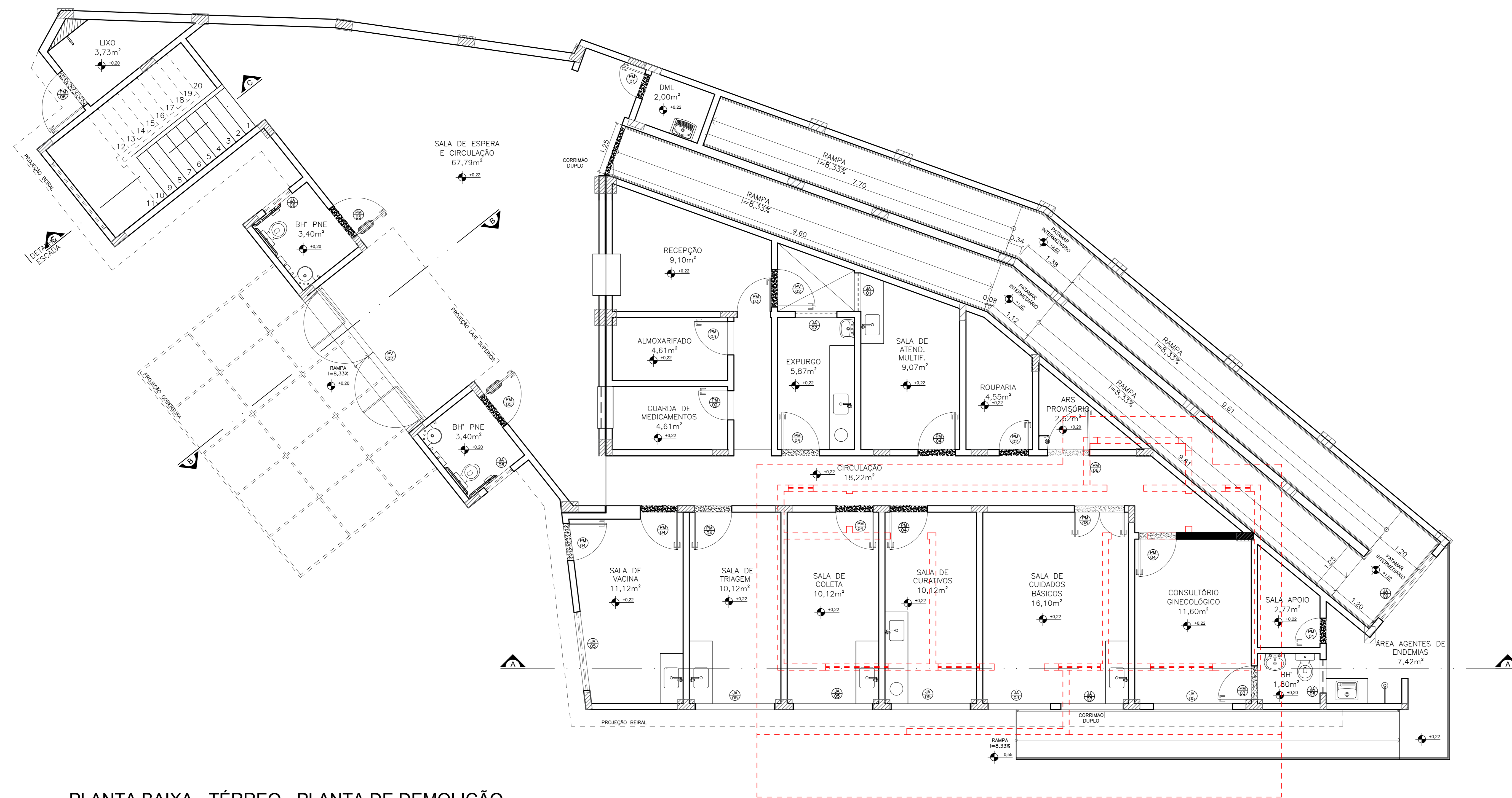
PLANTA BAIXA - TÉRREO - PLANTA DE DEMOLIÇÃO esc 1:50
