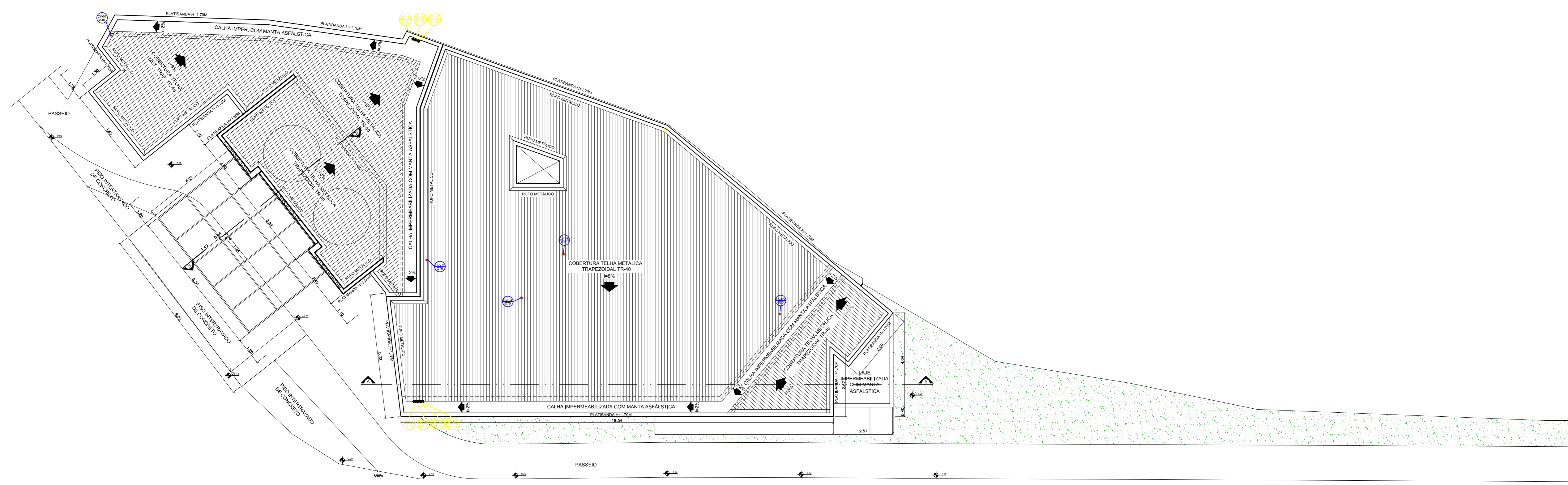
PLANTA DE IMPLANTAÇÃO E COBERTURA esc 1:100
