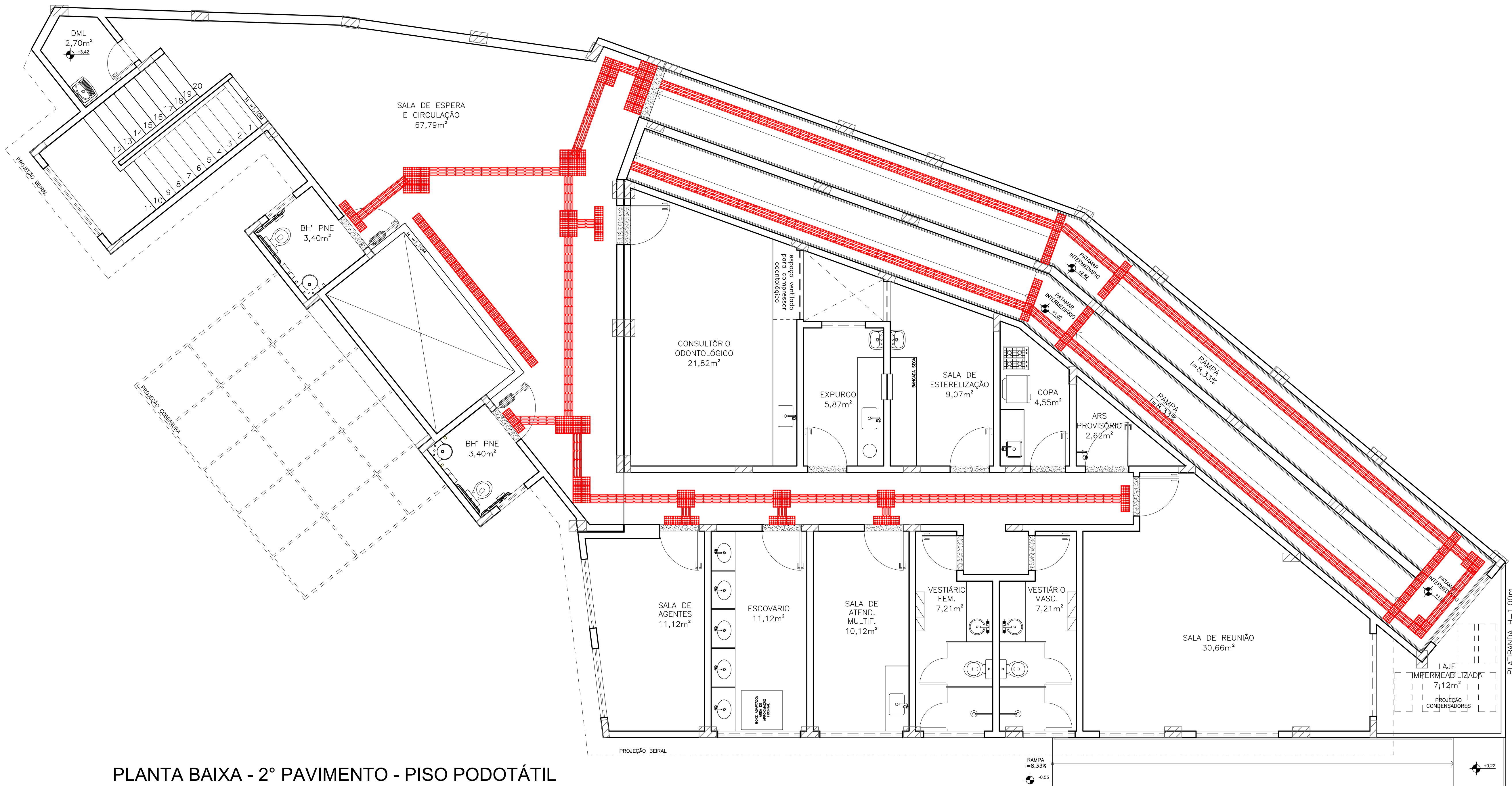
PLANTA BAIXA - 2º PAVIMENTO - PISO PODOTÁTIL esc 1:50
