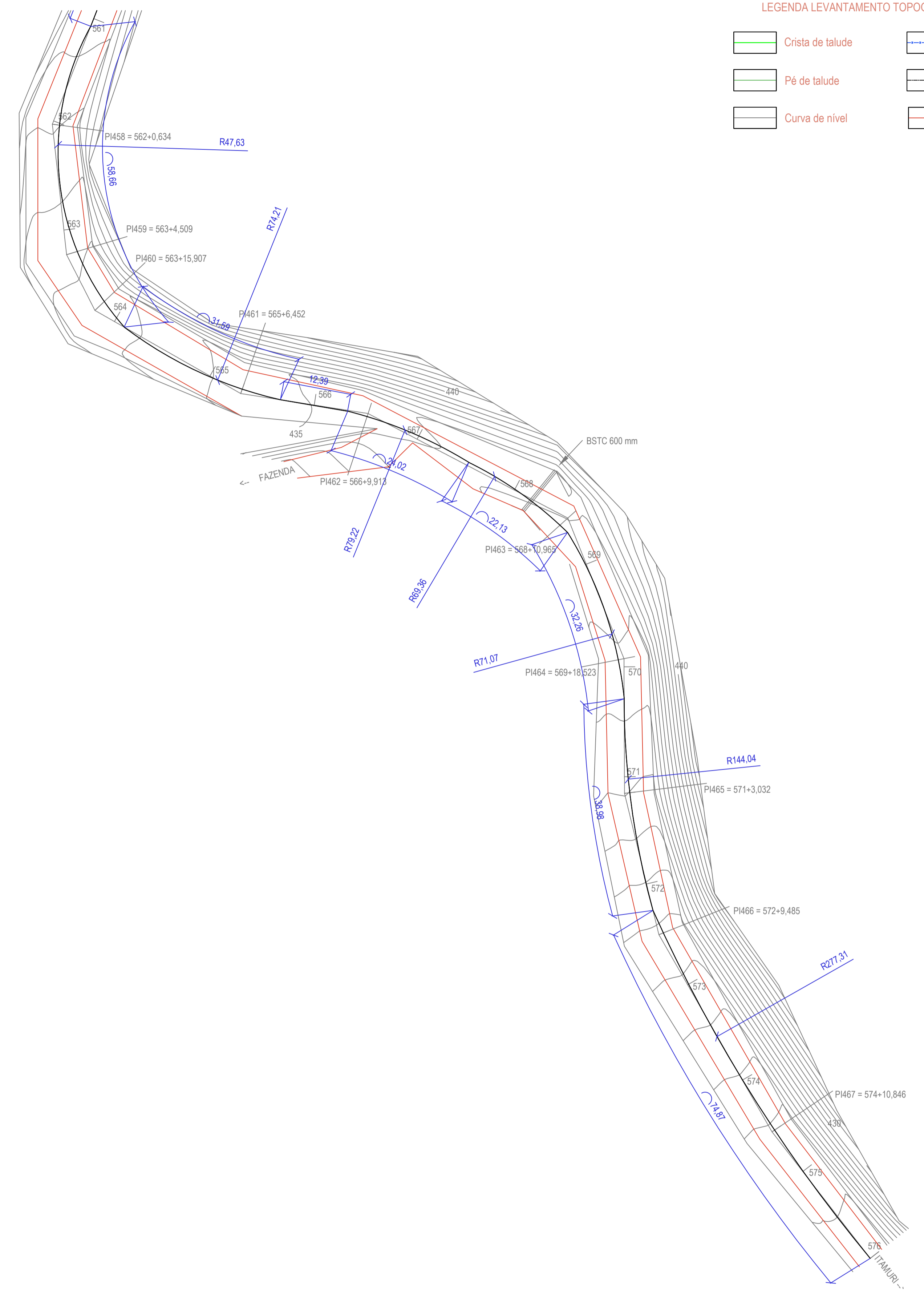
PROJETO GEOMÉTRICO - TRECHO A-A ESC: 1/500
