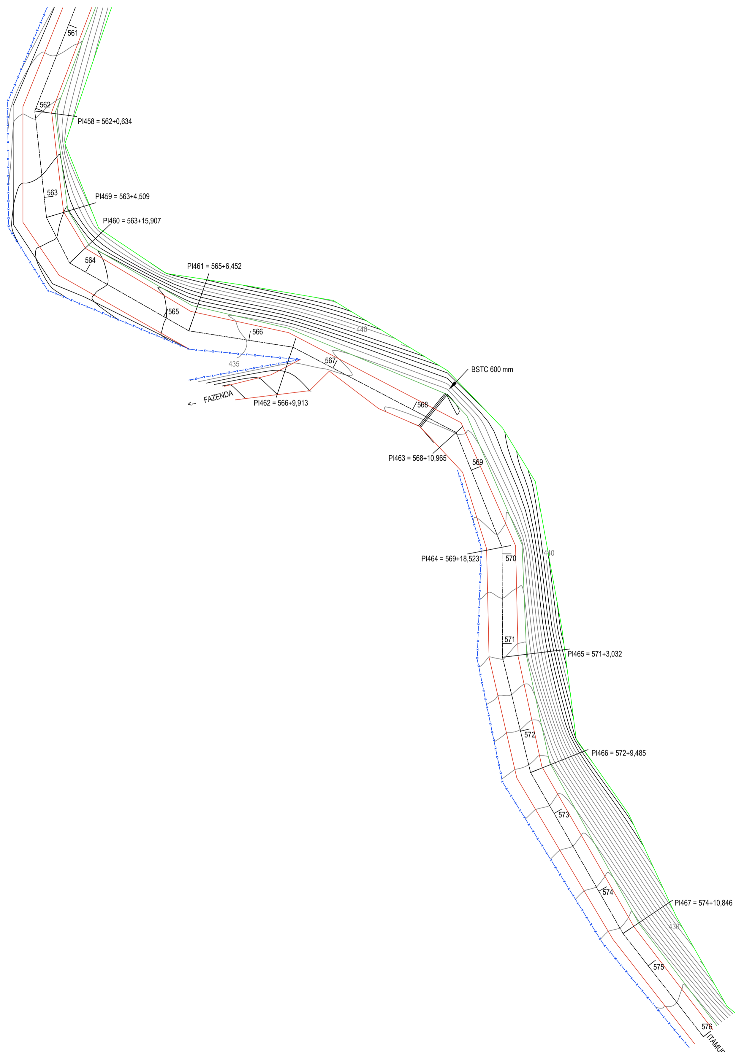
LEVANTAMENTO TOPOGRÁFICO PLANIATIMÉTRICO - TRECHO A-A ESC: 1/500
