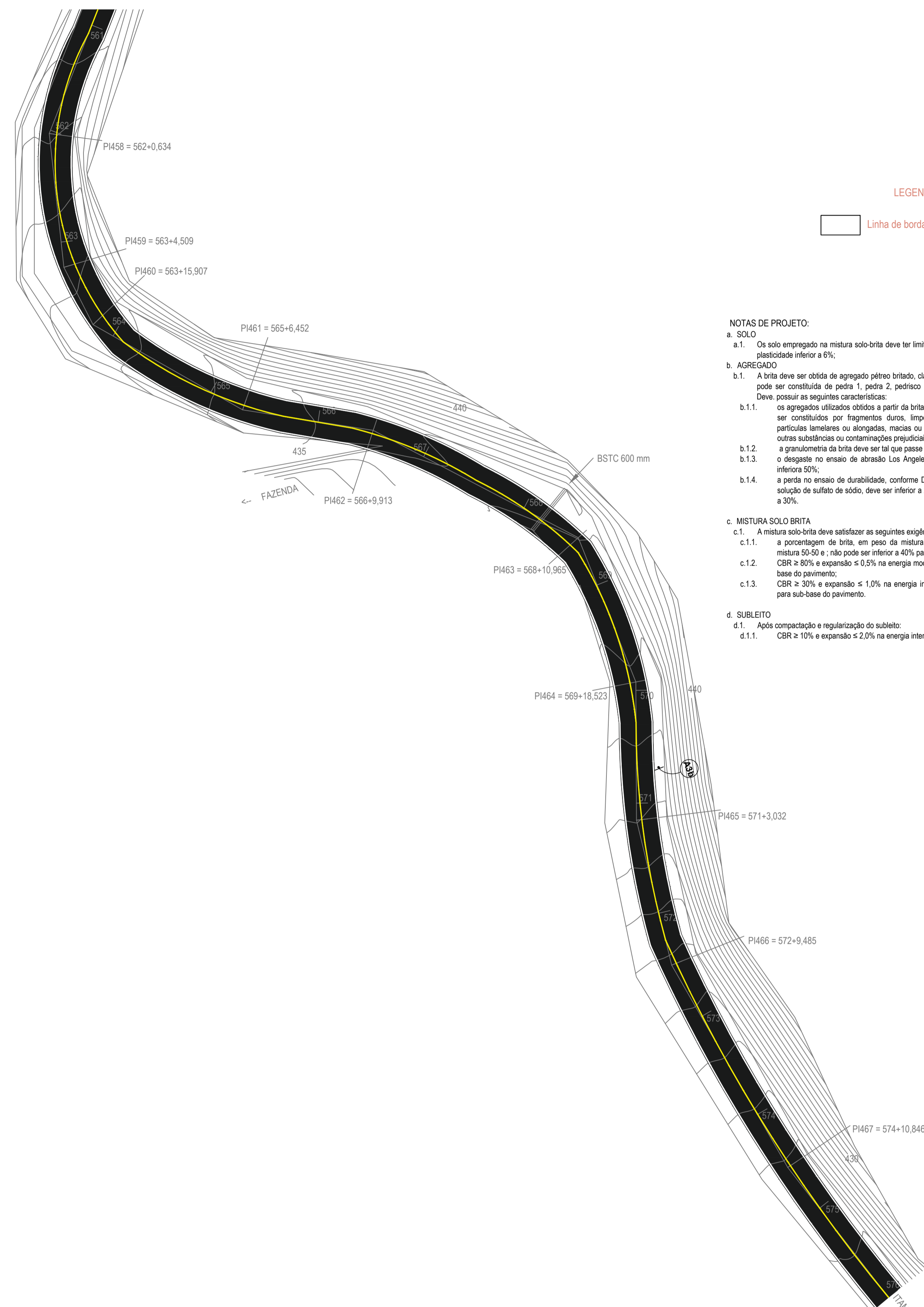
PROJETO DE SINALIZAÇÃO - TRECHO A-A ESC: 1/500
