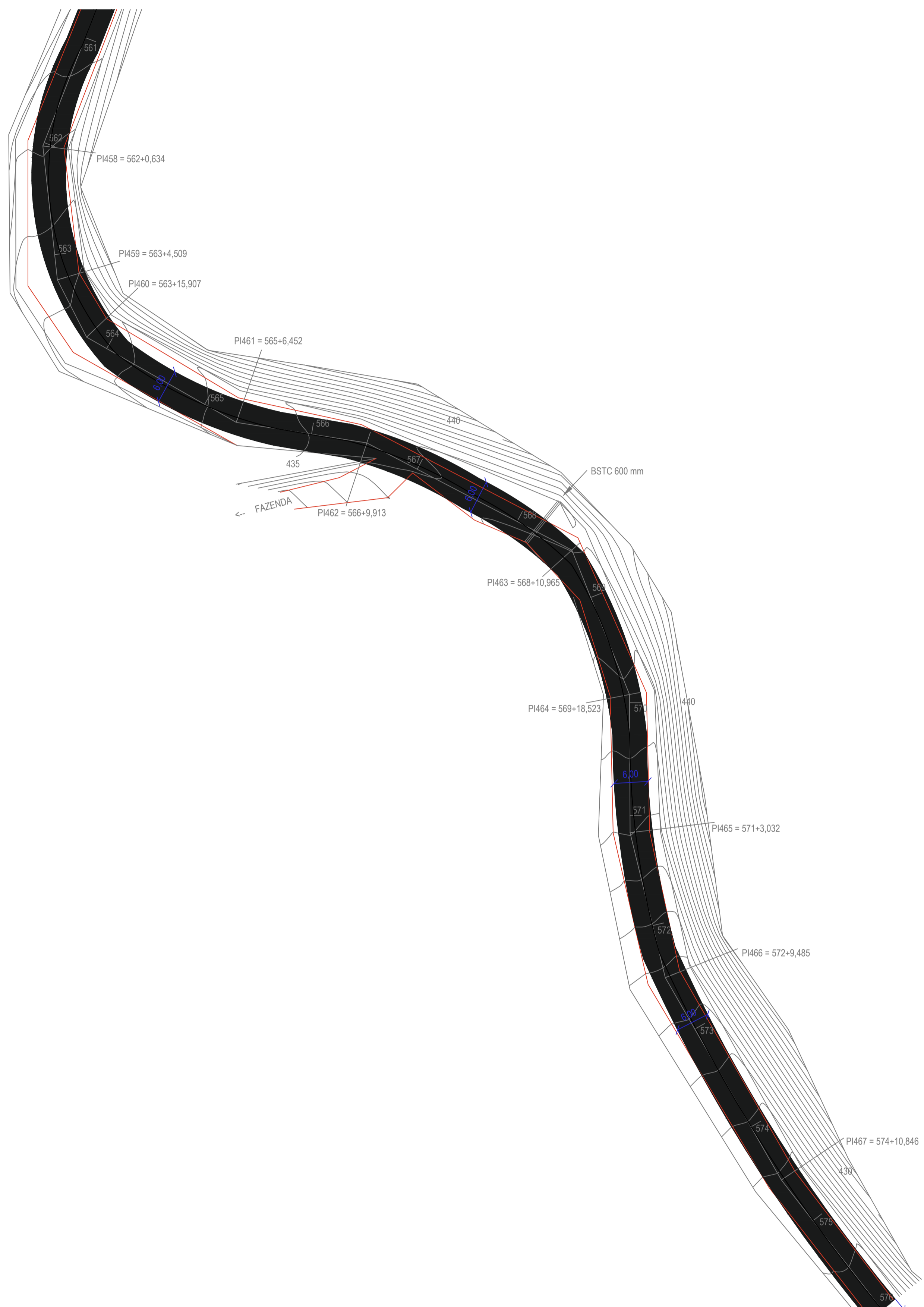
PROJETO DE PAVIMENTAÇÃO - TRECHO A-A ESC: 1/500
