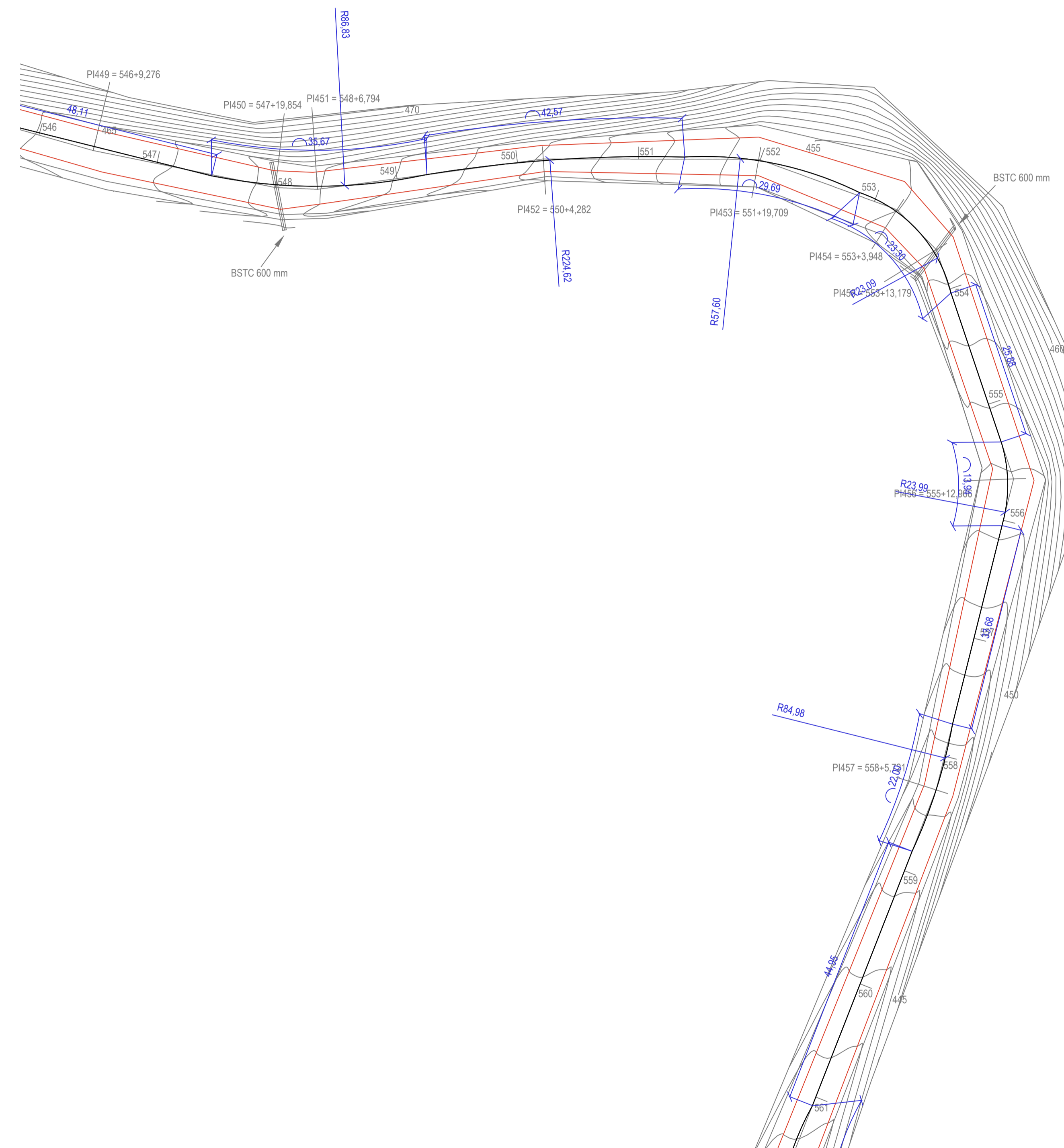
PROJETO GEOMÉTRICO - TRECHO B-B ESC: 1/500
