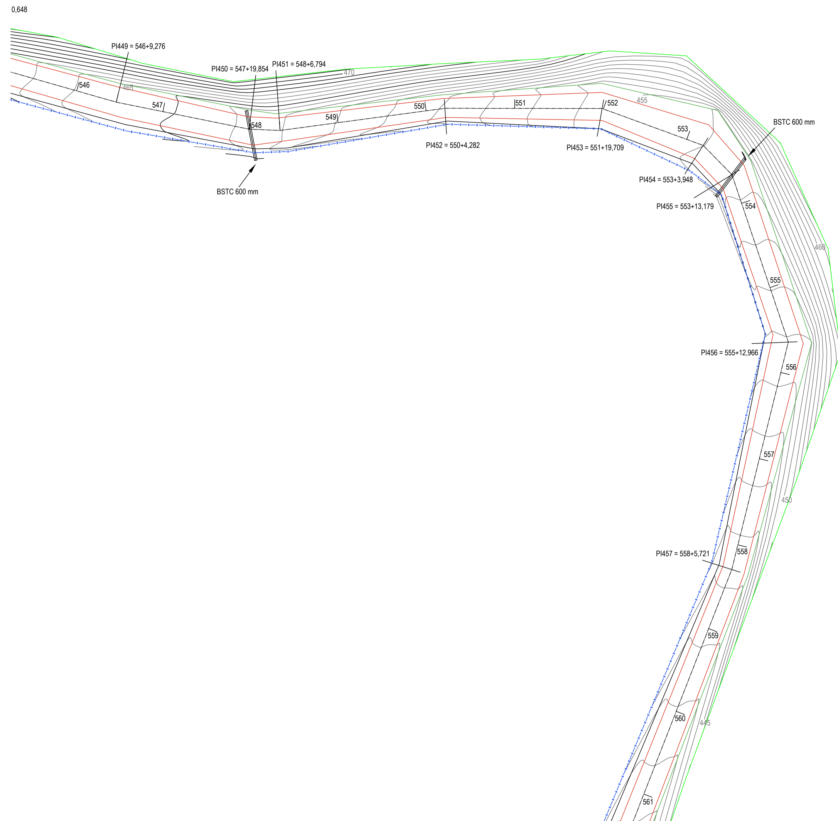
LEVANTAMENTO TOPOGRÁFICO PLANIATIMÉTRICO - TRECHO B-B ESC: 1/500
