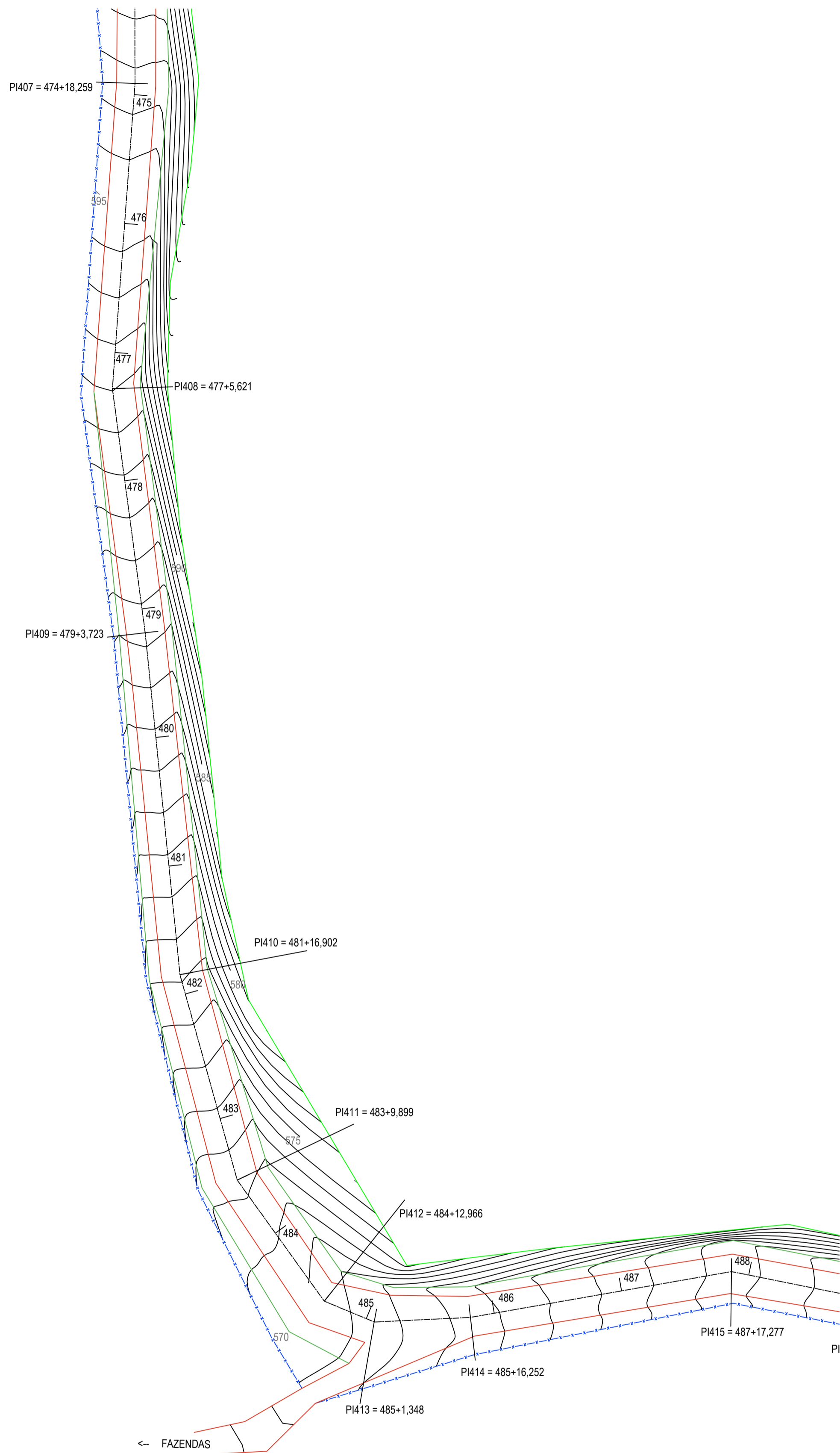
LEVANTAMENTO TOPOGRÁFICO PLANIATIMÉTRICO - TRECHO H-H ESC: 1/500
