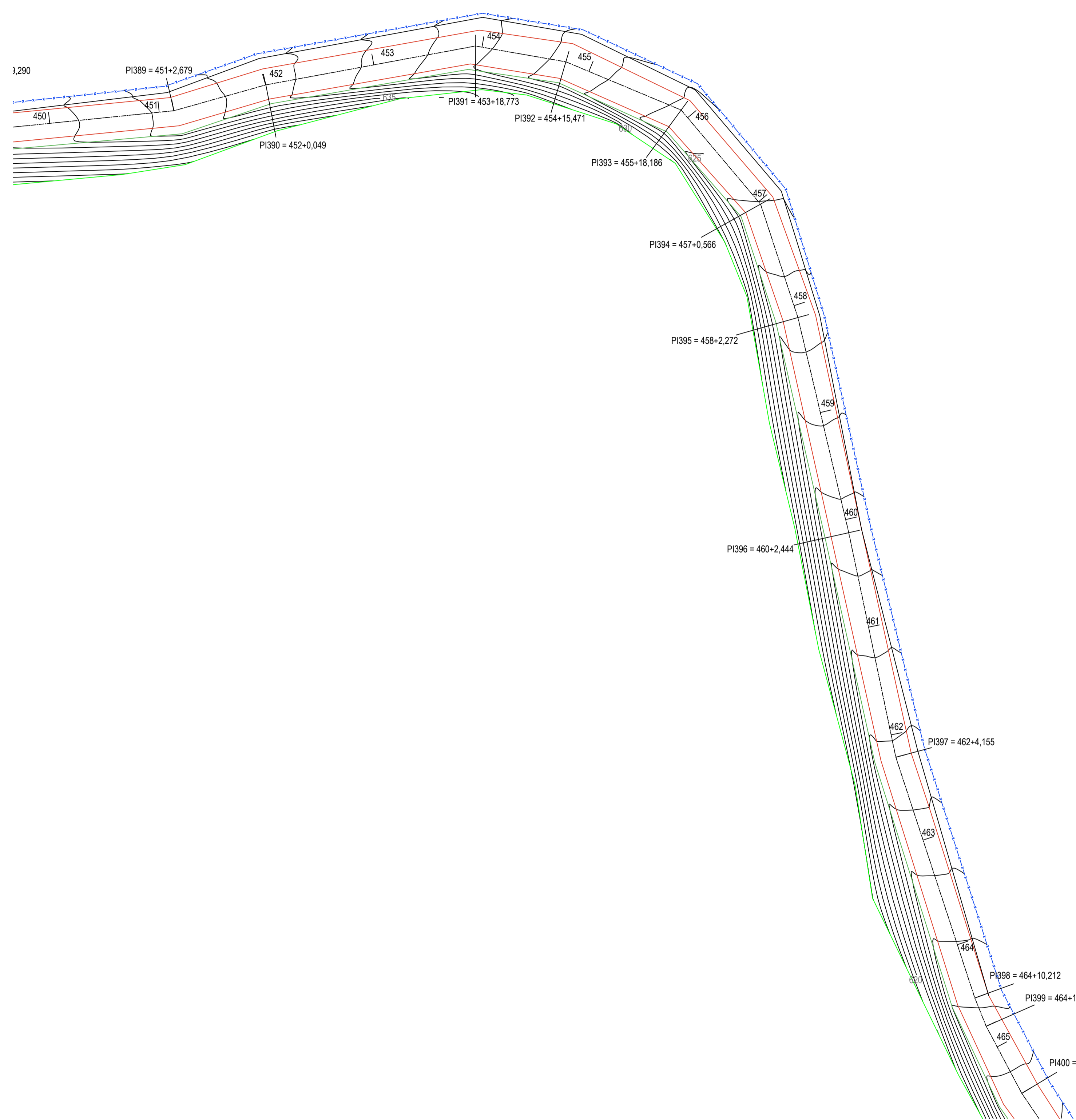
LEVANTAMENTO TOPOGRÁFICO PLANIATIMÉTRICO - TRECHO J-J ESC: 1/500
