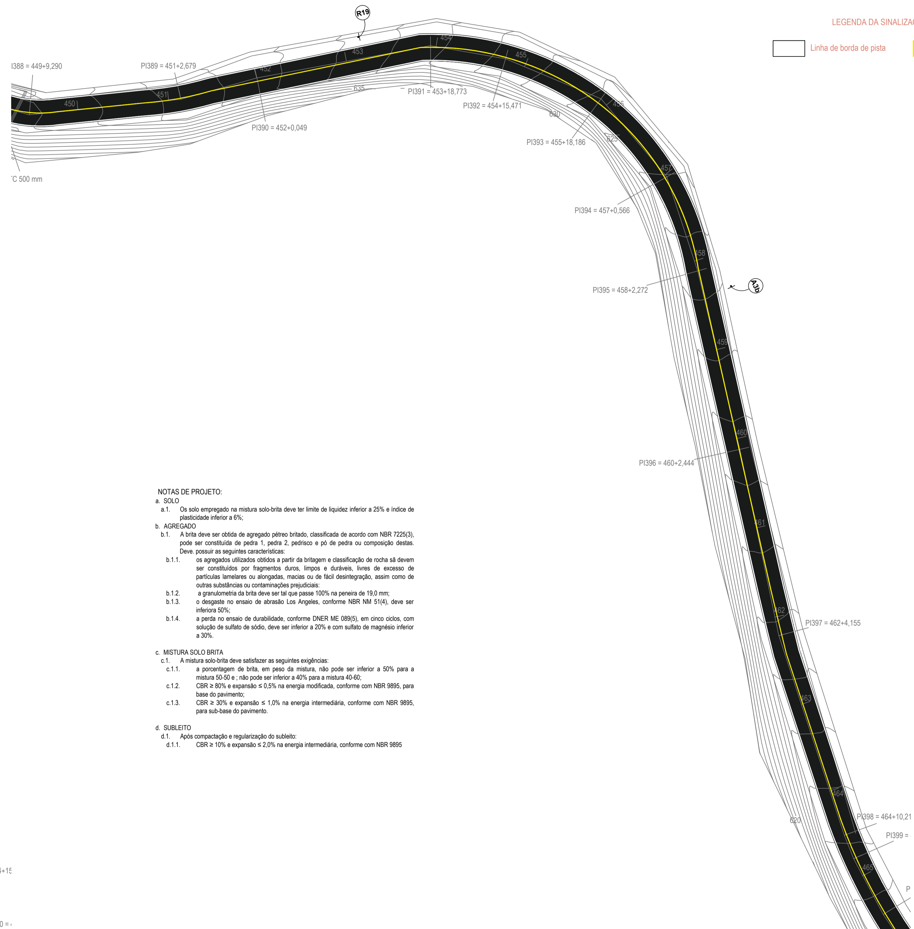
PROJETO DE SINALIZAÇÃO - TRECHO J-J ESC: 1/500
