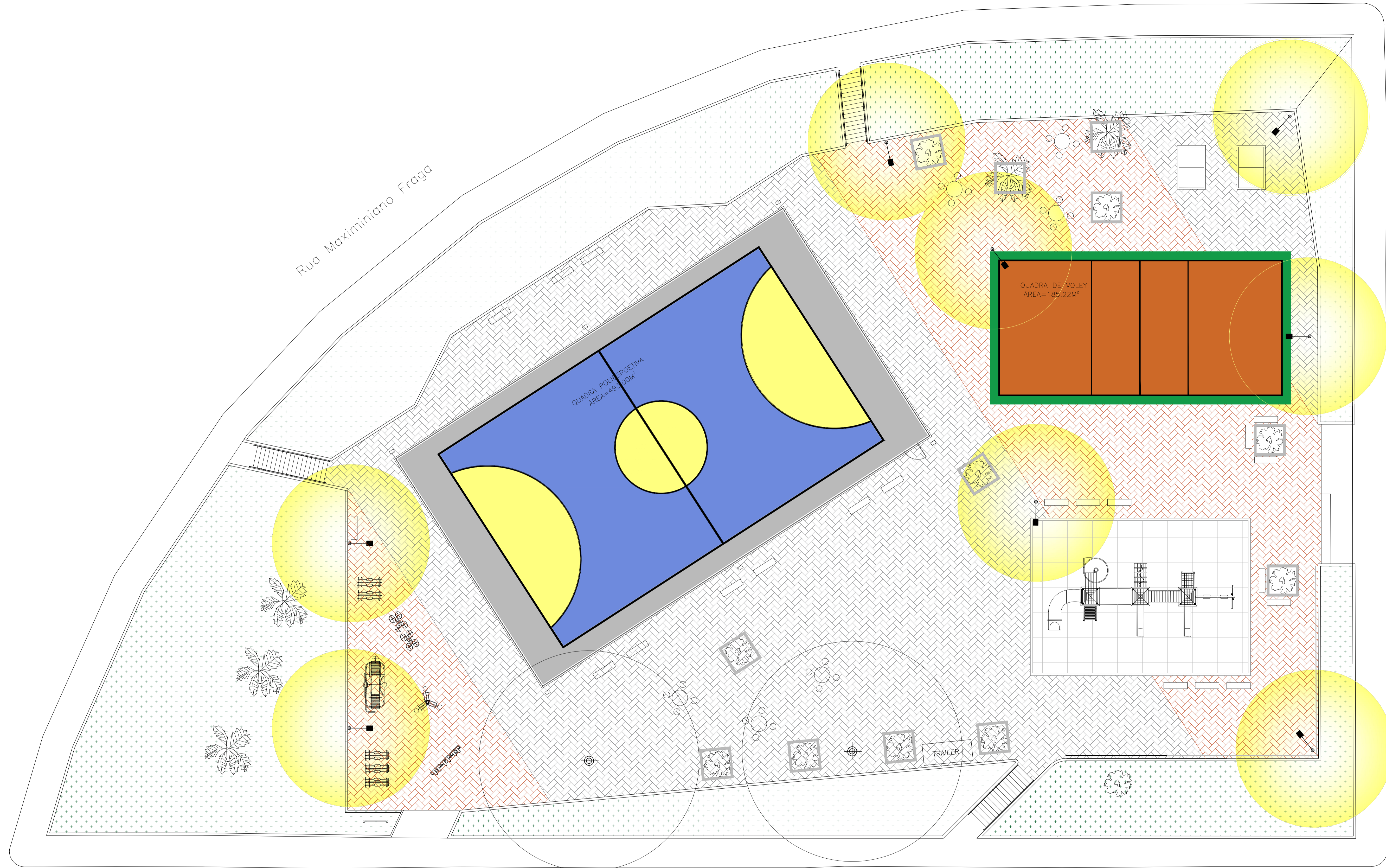
PLANTA BAIXA – PROJEÇÃO DE ILUMINAÇÃO ESC 1:125
