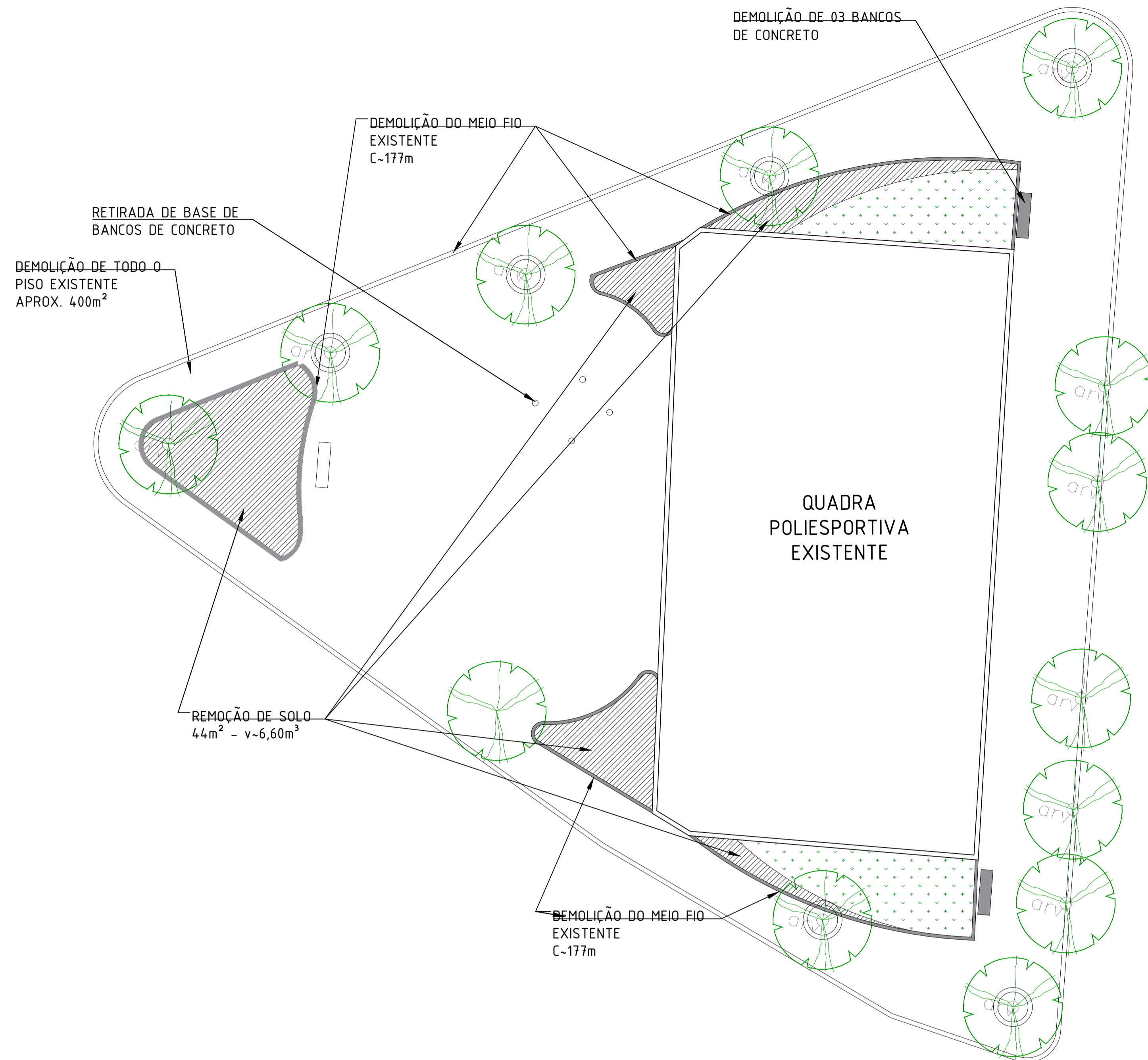
PLANTA BAIXA – DEMOLIÇÃO ESC 1:100
