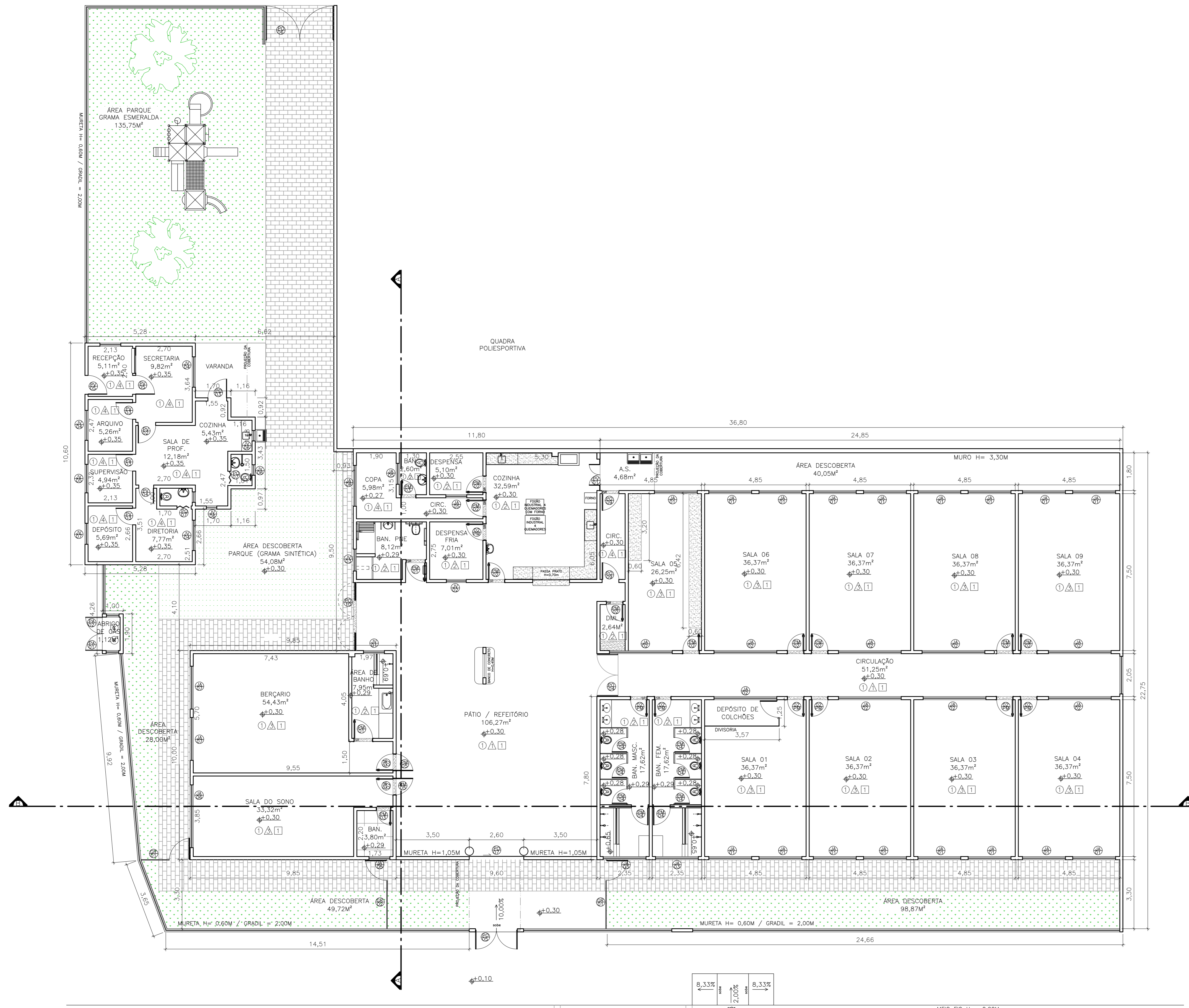
PLANTA BAIXA - SITUAÇÃO FINAL ESC.: 1/100
