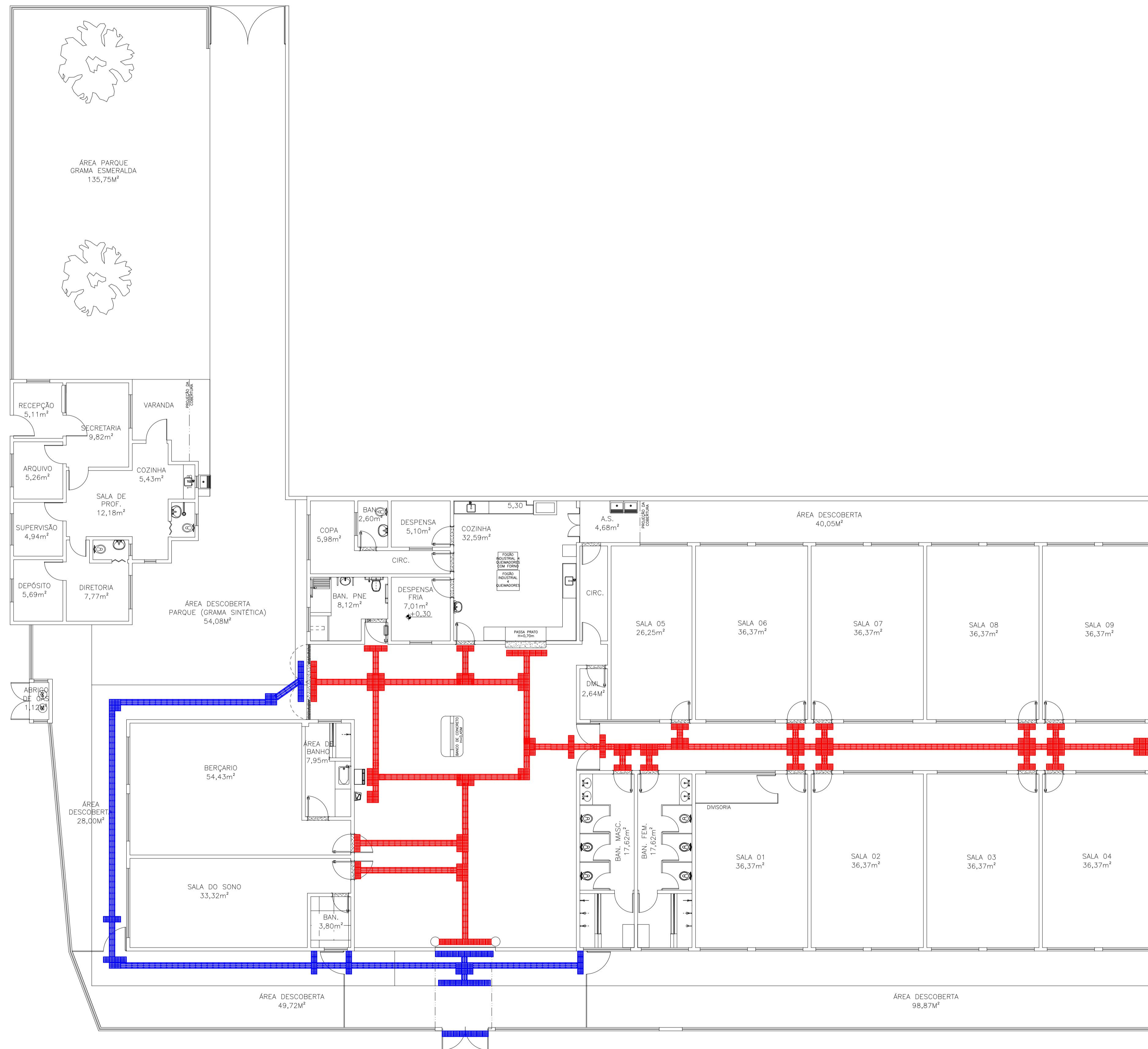
PLANTA BAIXA - PAGINAÇÃO DE PISO TÁTIL ESC.: 1/ 100
