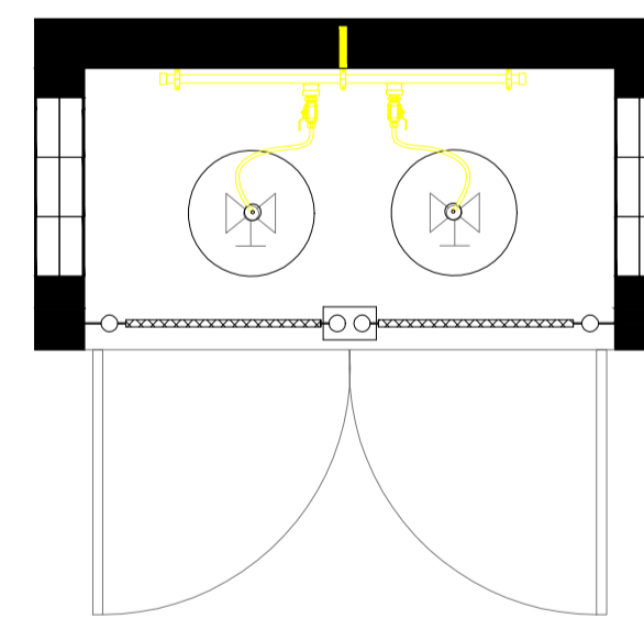
DETALHE ABRIGO DE GÁS ESCALA 1:50
