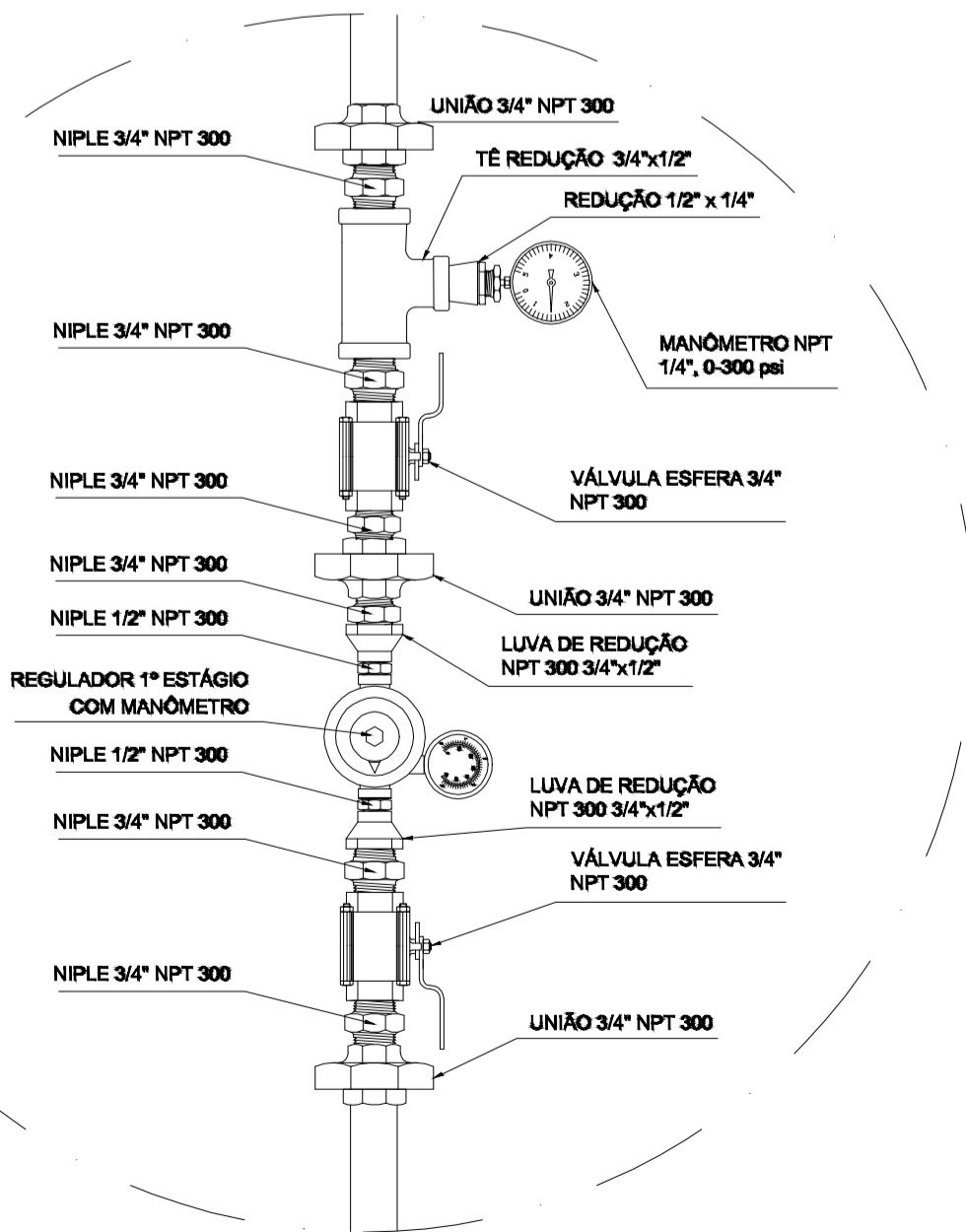
DETALHE DO REGULADOR DE 1º ESTÁGIO SEM ESCALA
