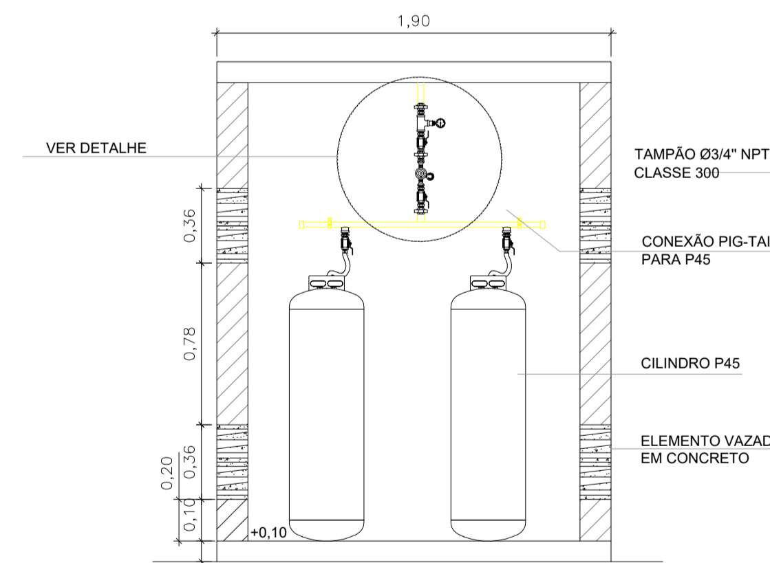
DETALHE ABRIGO DE GÁS ESCALA 1:50
