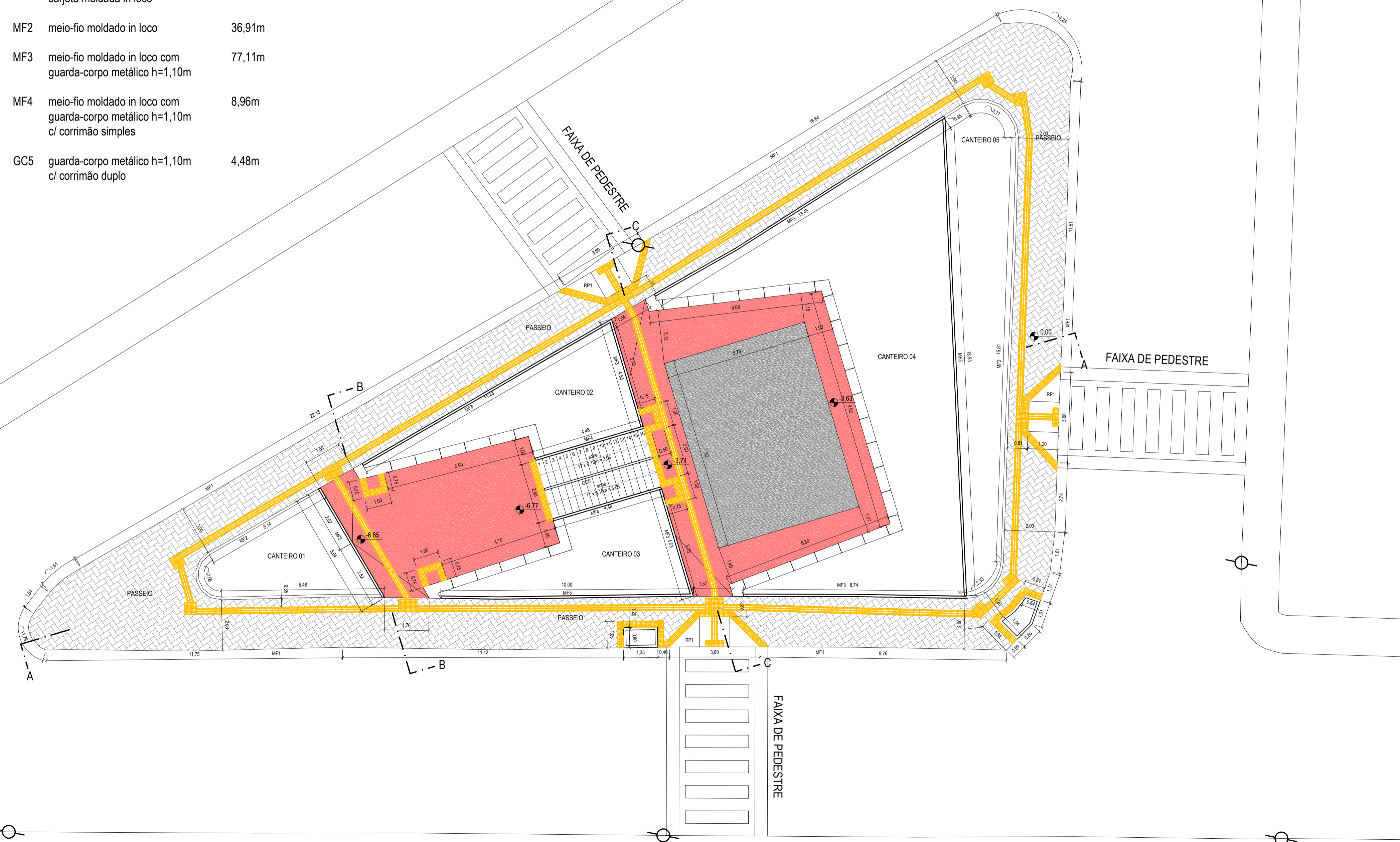
PLANTA BAIXA ESC: 1/100
