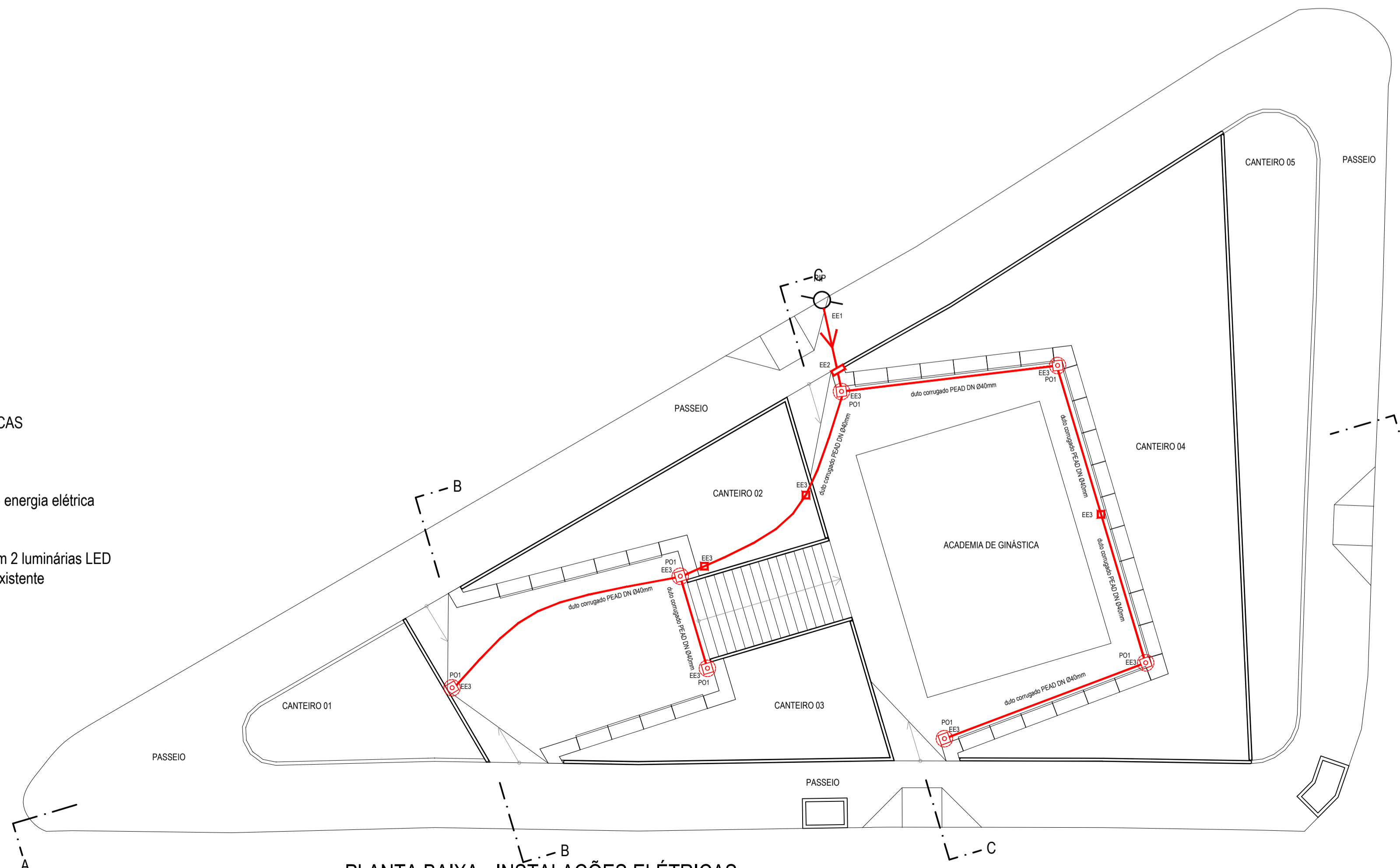
PLANTA BAIXA - INSTALAÇÕES ELÉTRICAS ESC: 1/100
