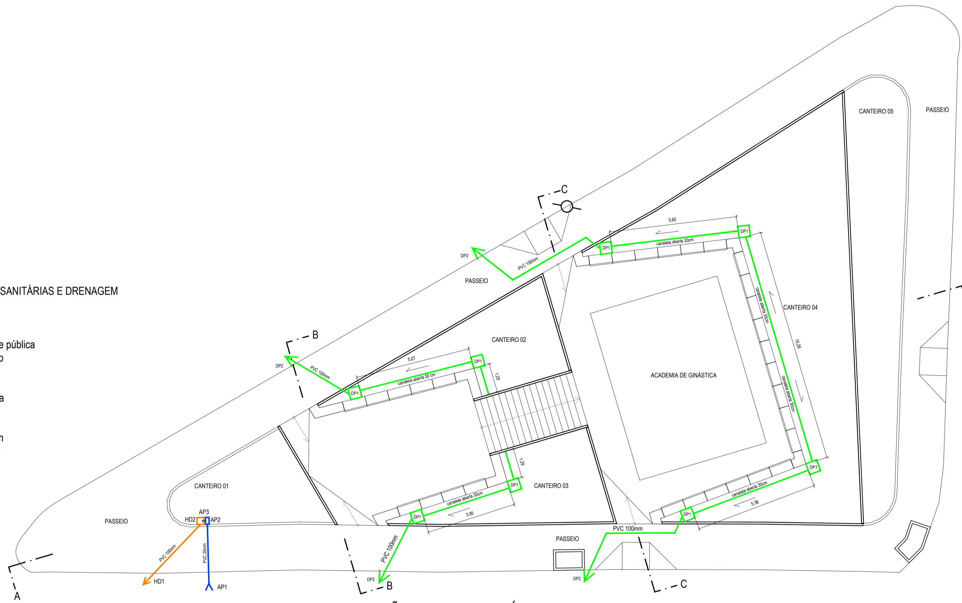
PLANTA BAIXA - INSTALAÇÕES HIDROSSANITÁRIAS E DRENAGEM ESC: 1/100
