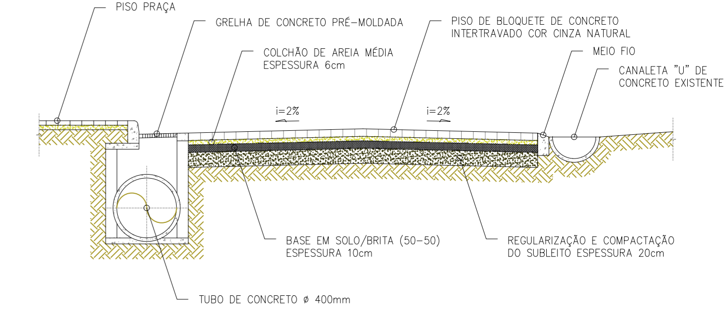
DETALHE TÍPICO DA PISTA DE ROLAMENTO
