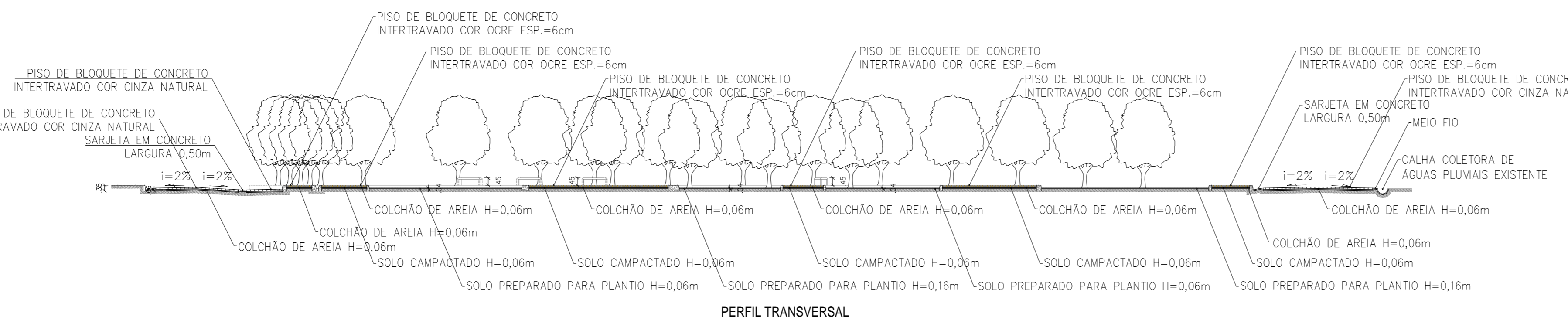
PERFIL TRANSVERSAL see 1:50
