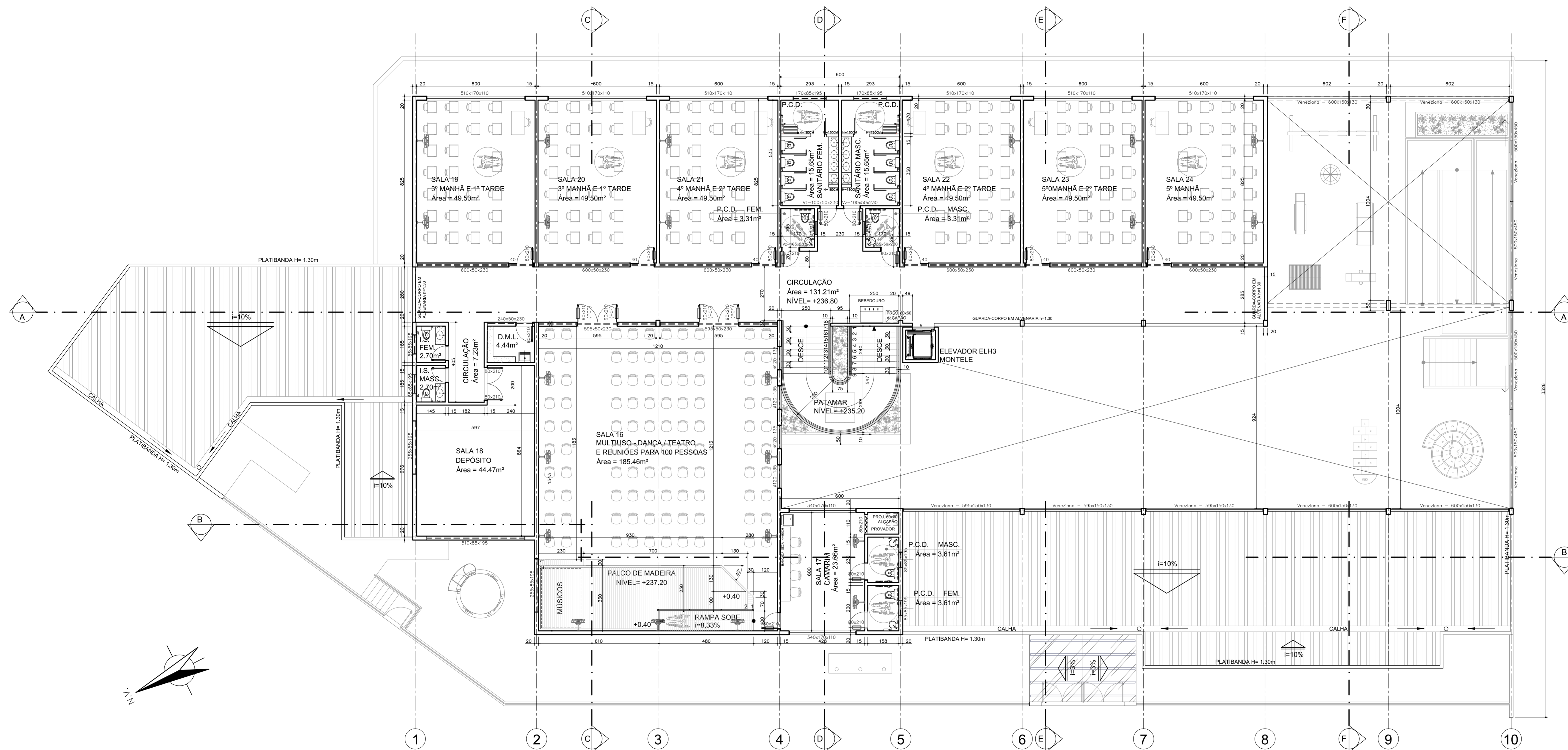
PLANTA BAIXA DO 2º PAVIMENTO ESCALA - 1/100
