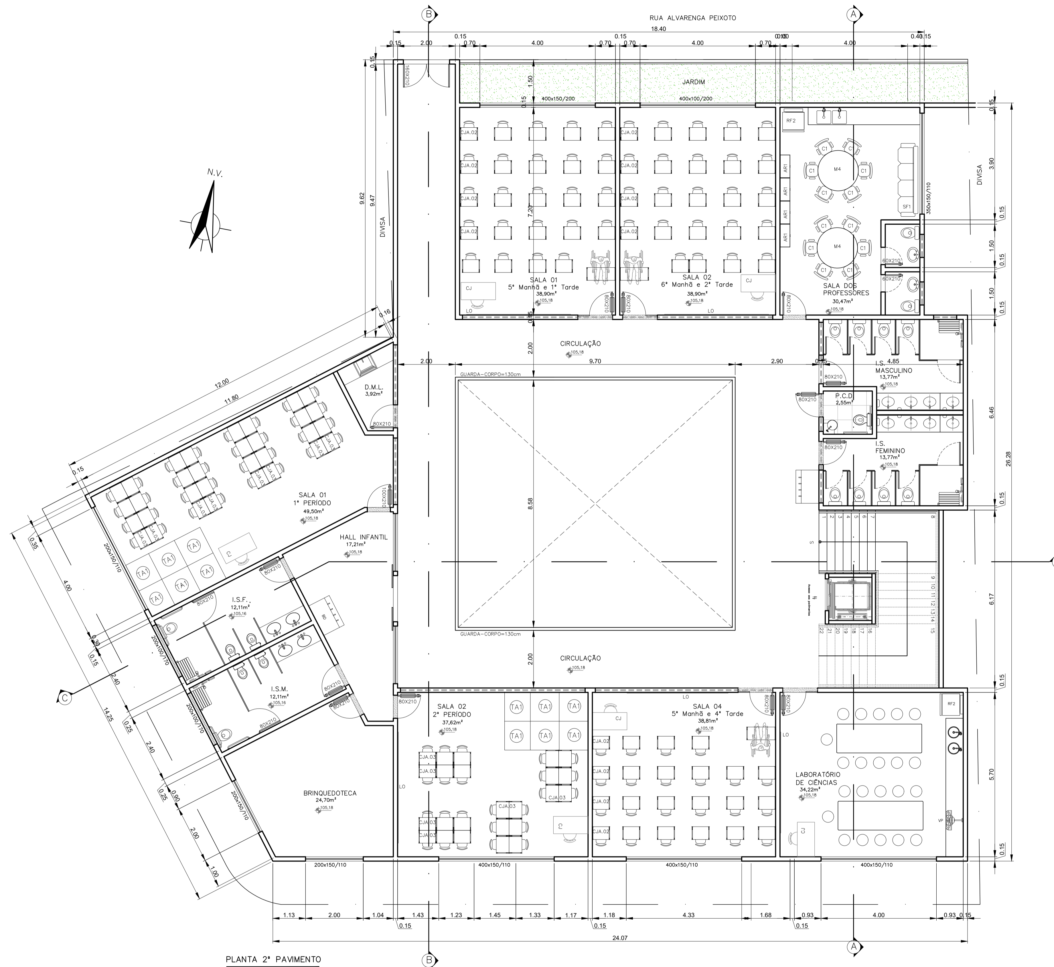
PLANTA 2º PAVIMENTO
