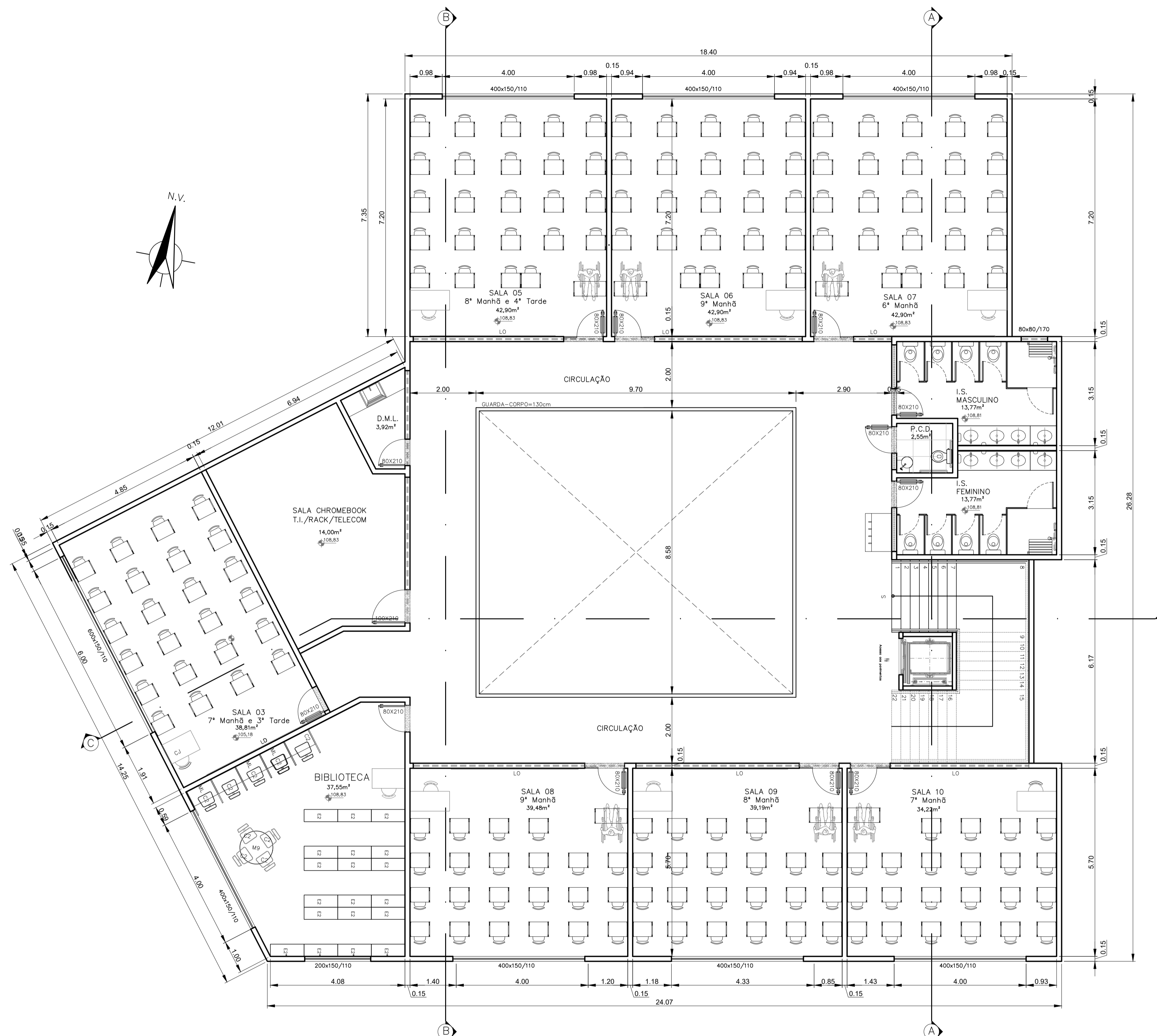
PLANTA 3º PAVIMENTO ESCALA 1:75
