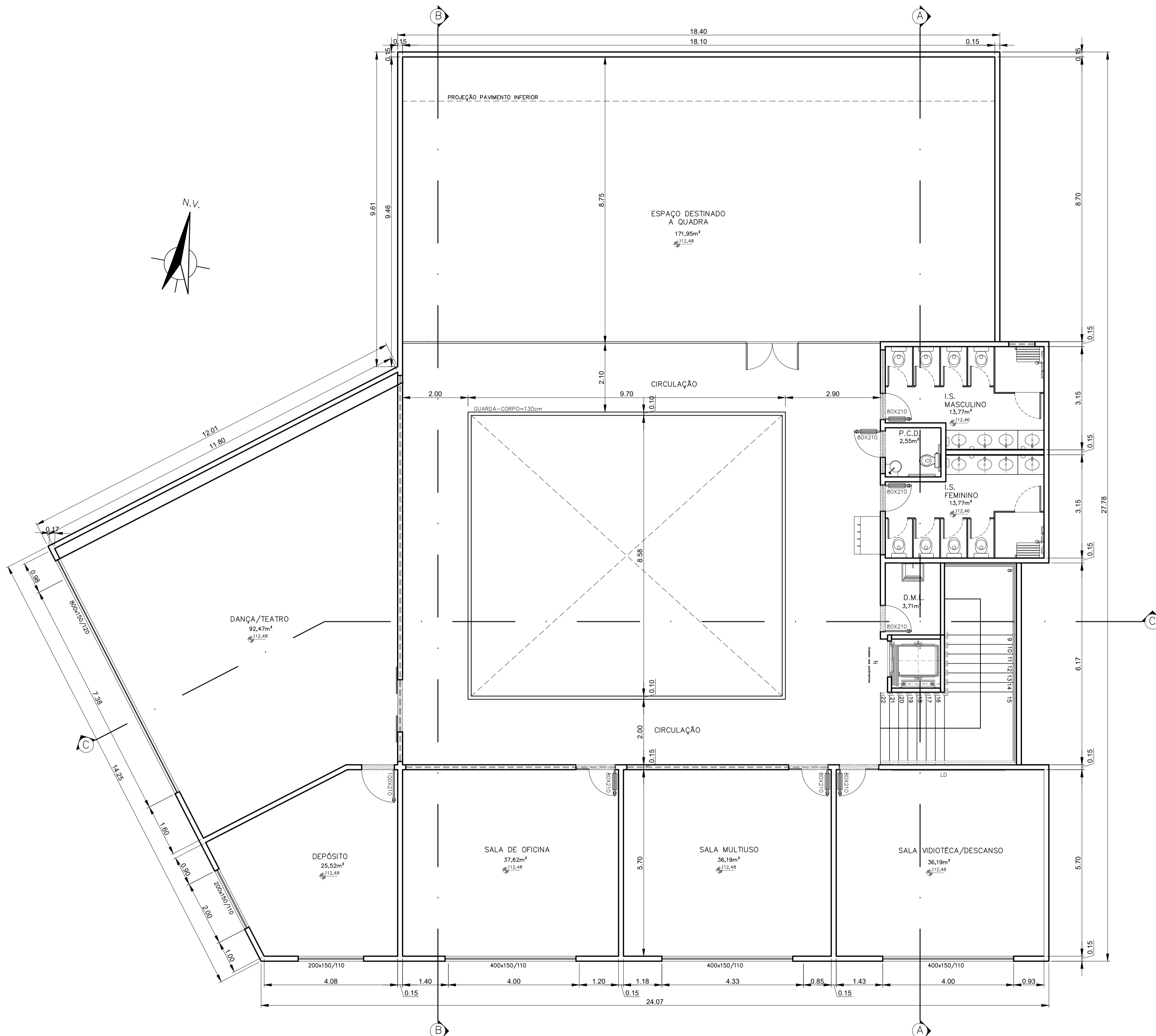
PLANTA 4º PAVIMENTO ESCALA: 1:75
