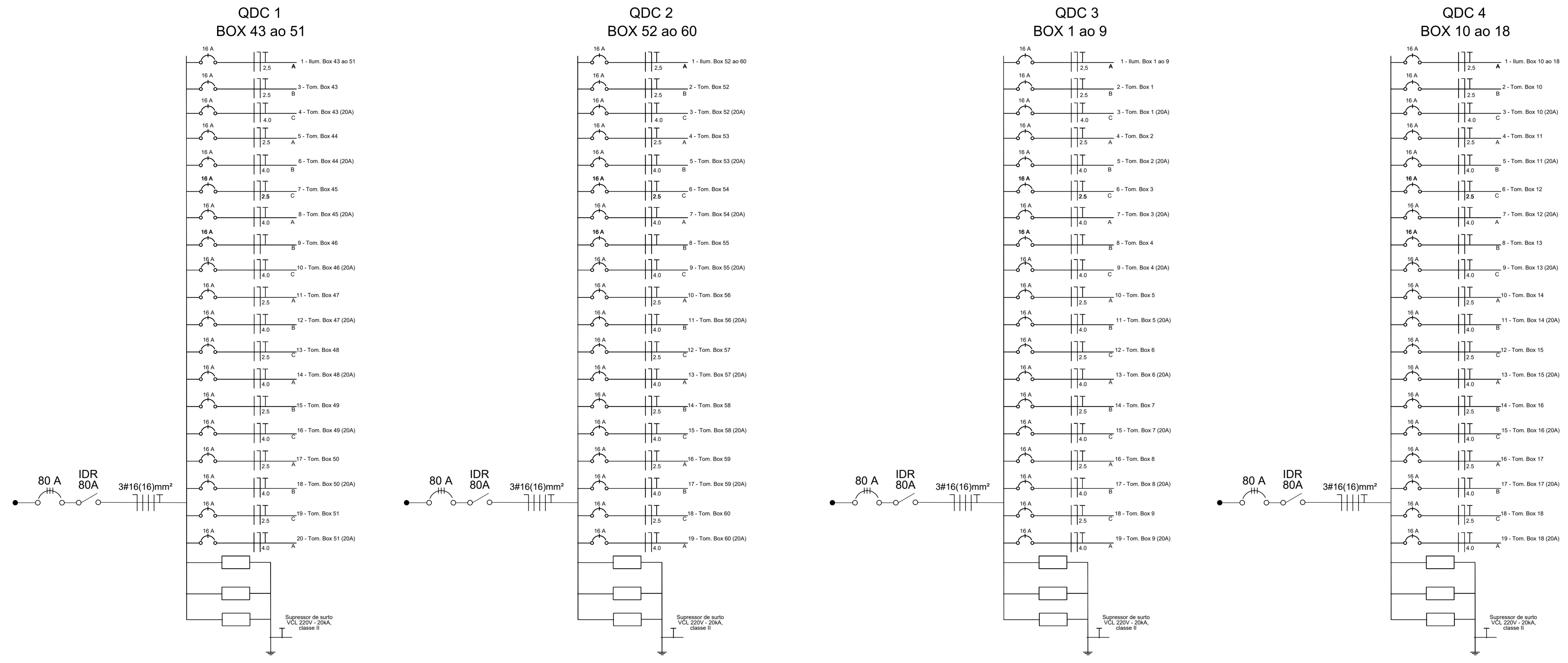
DIAGRAMA UNIFILAR – QDC BOX 01, 02, 03 E 04 ESC. 1:50
