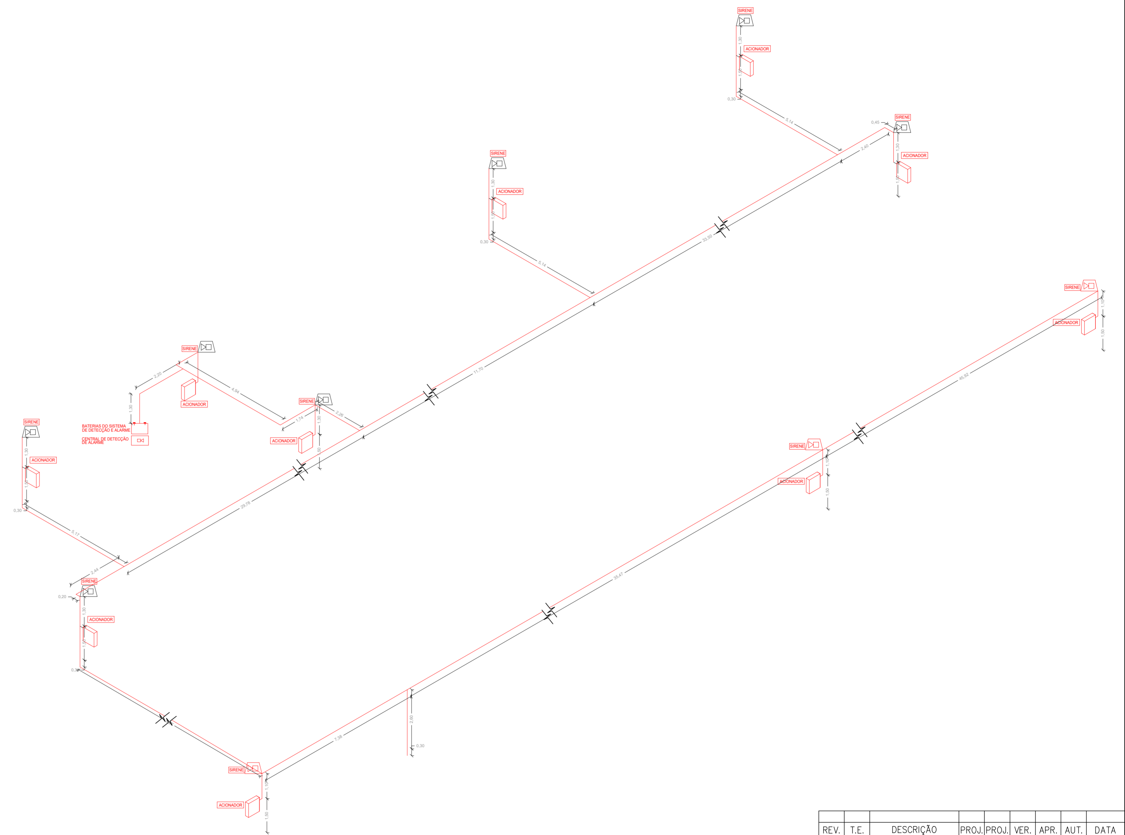
DIAGRAMA ISOMÉTRICO - SISTEMA DE ALARME DE INCÊNDIO SEM ESCALA
