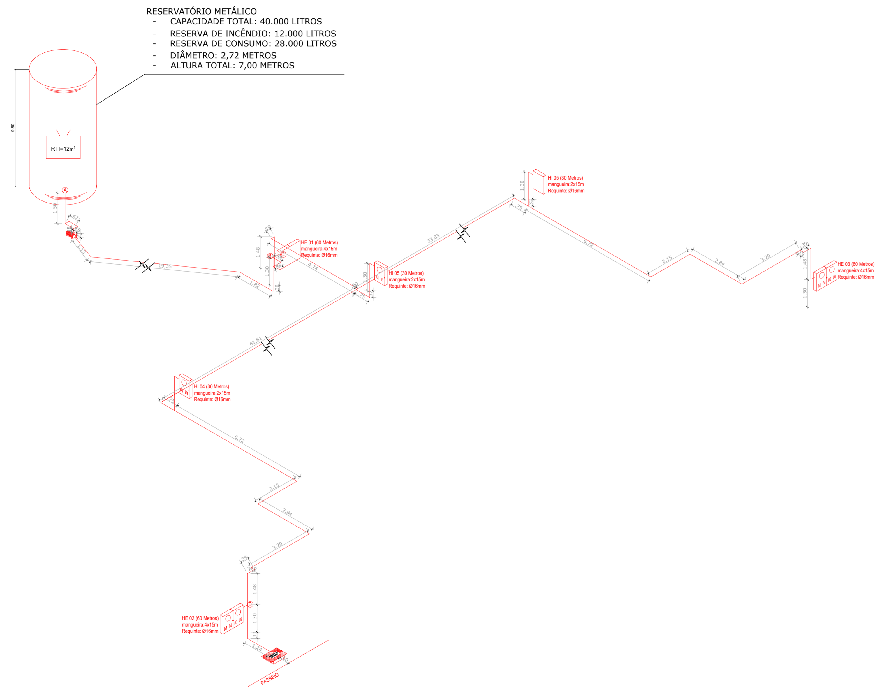
DIAGRAMA ISOMÉTRICO - SISTEMA DE HIDRANTES SEM ESCALA
