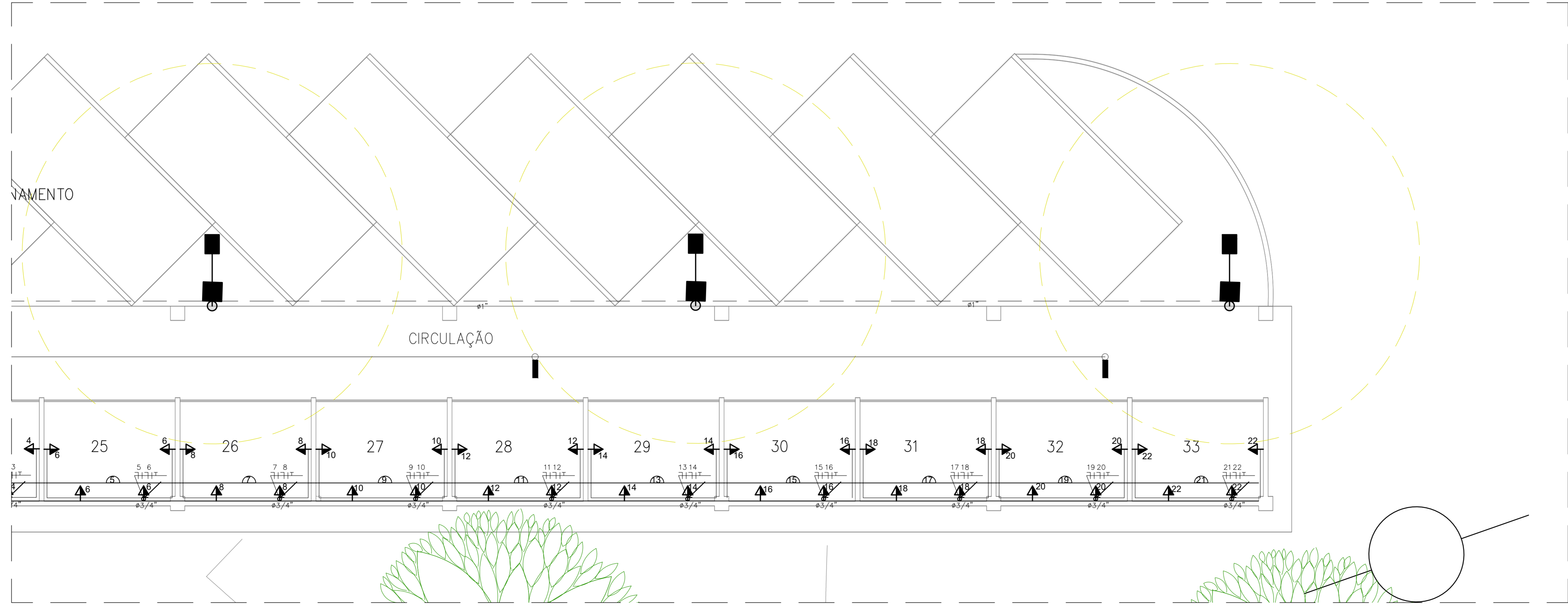
PLANTA DE LIGAÇÃO ELÉTRICA – CAMELÓDROMO PARTE 03 ESC. 1:50
