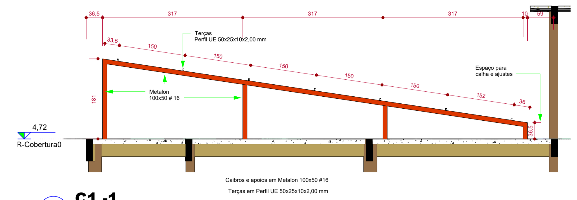
C1 - 1 ESCALA - 1 : 50
