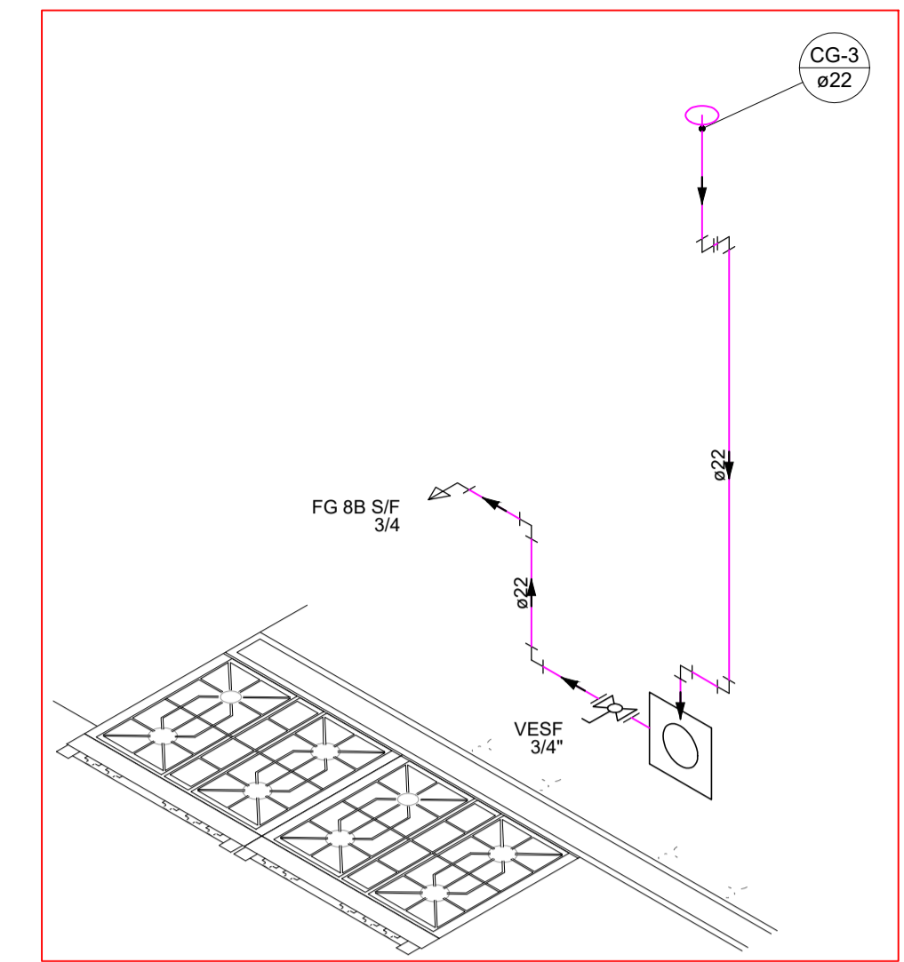
Detalhe GÁS-2 Escala 1:25
