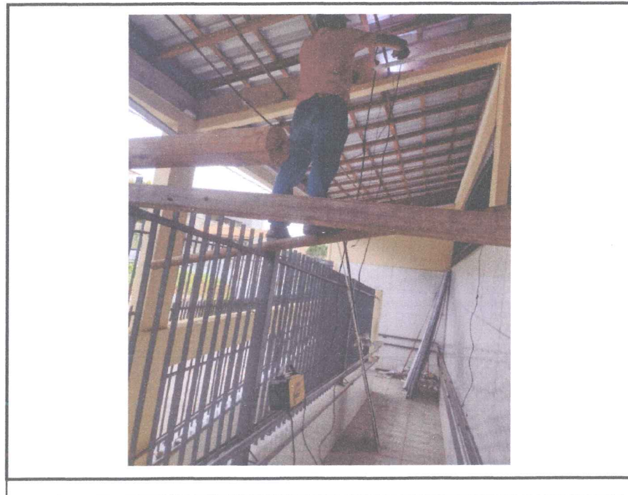
Foto 2: INSTALAÇÃO E APLICAÇÃO DE ZARCÃO NA ESTRUTURA DO FORRO.
