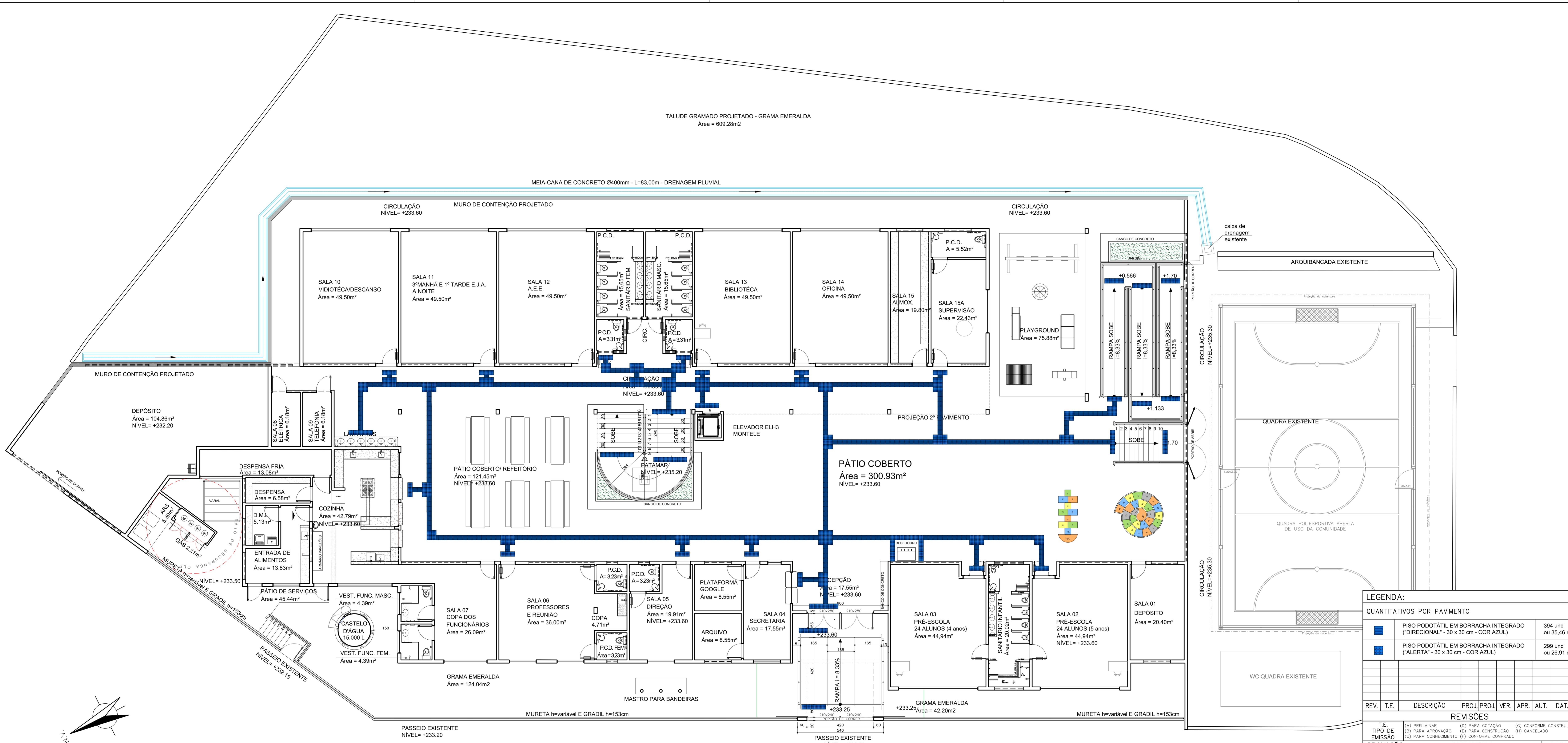
PLANTA PISO TÁTIL - 1º PAVIMENTO ESCALA - 1/100
