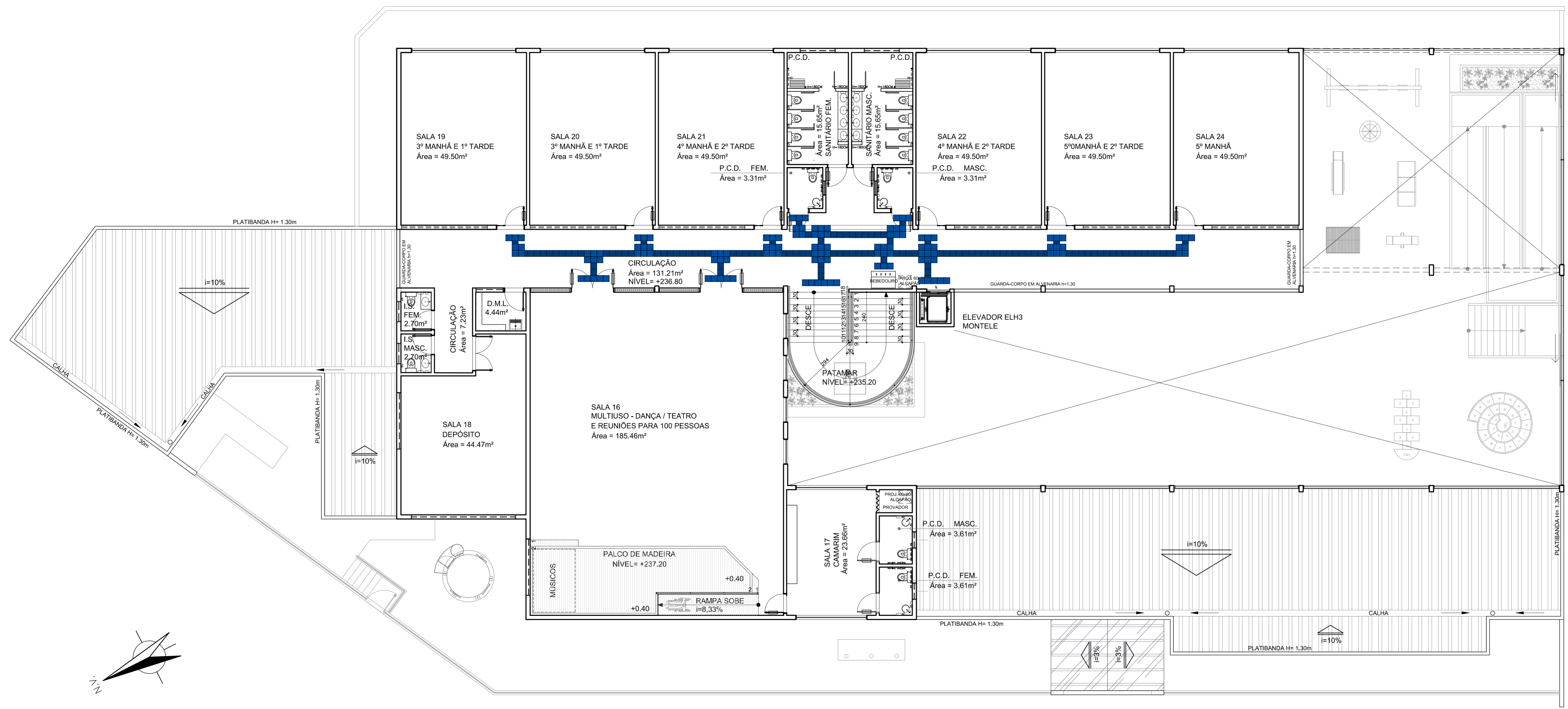
PLANTA PISO TÁTIL - 2º PAVIMENTO ESCALA - 1/100
