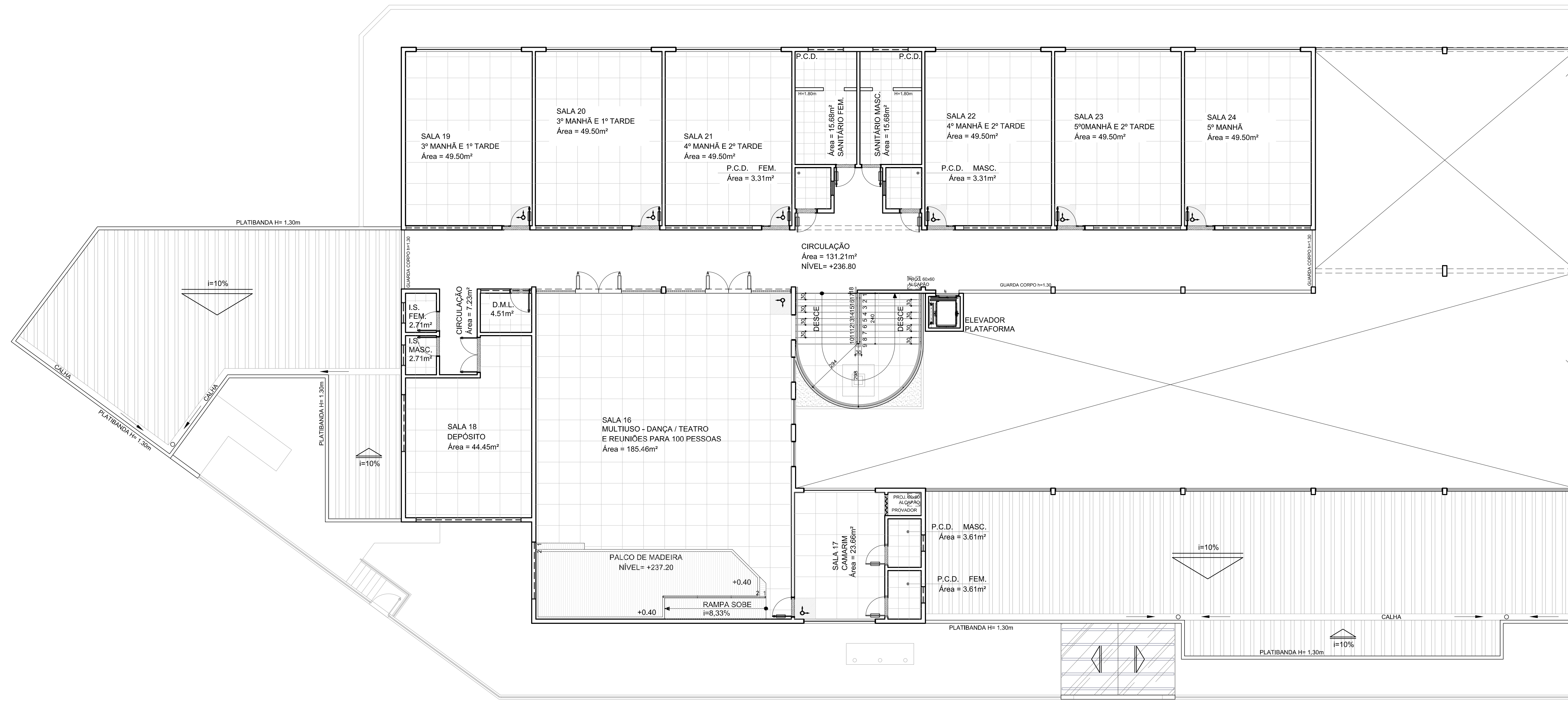
PAGINAÇÃO DE PISO 2º PAVIMENTO ESCALA - 1/100
