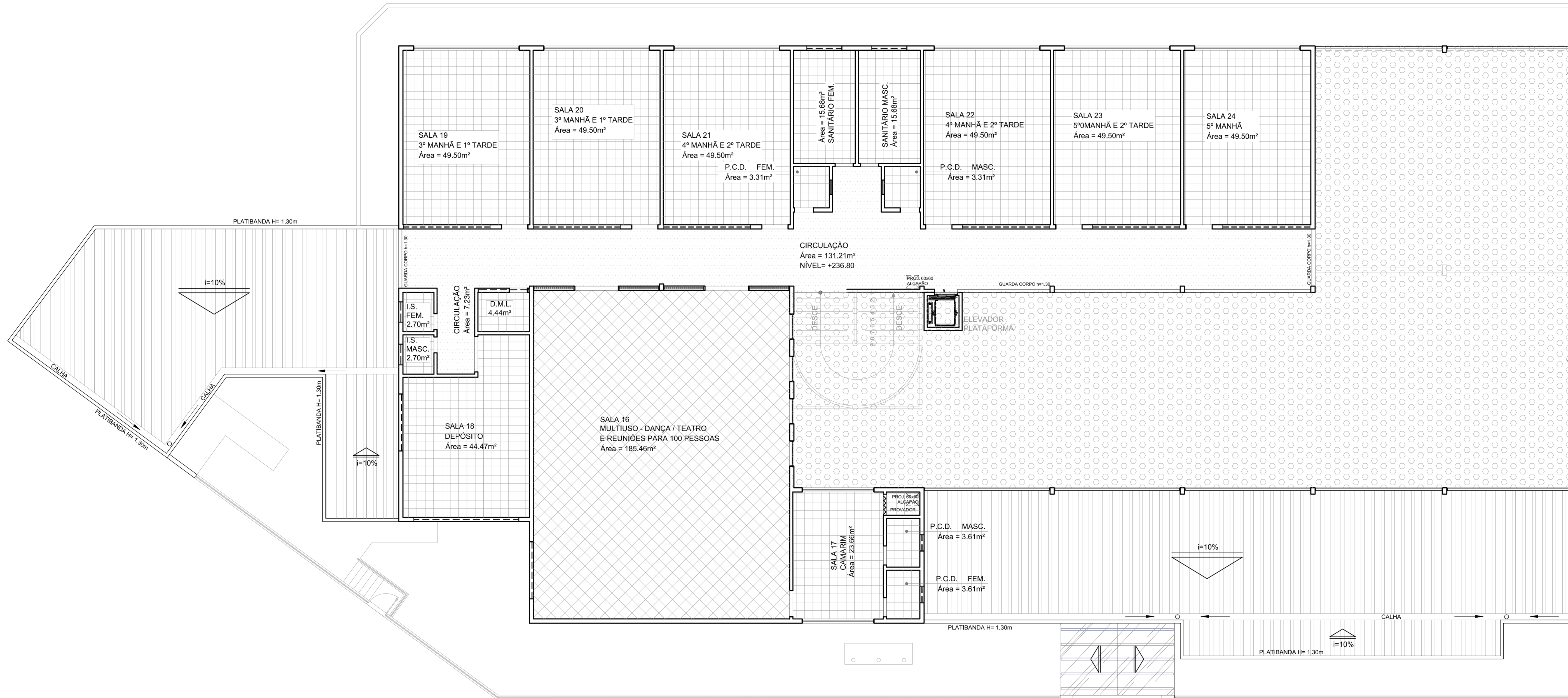
PLANTA TETO 2º PAVIMENTO ESCALA - 1/100
