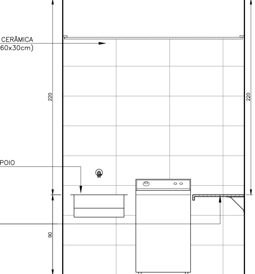
VISTA 02 DML 1º PAVIMENTO ESCALA 1:25
