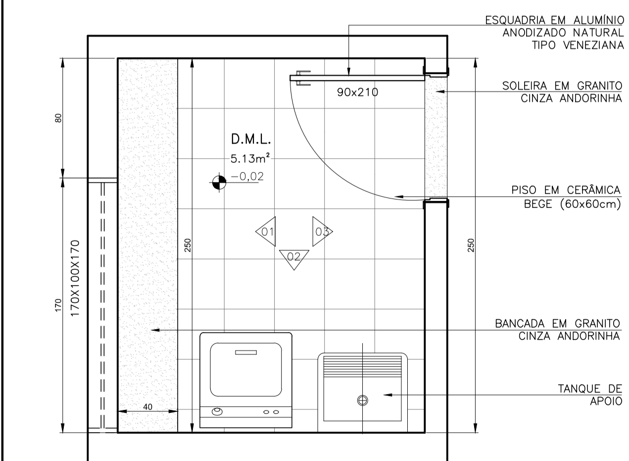
PLANTA LAYOUT DML 1º PAVIMENTO ESCALA 1:25
