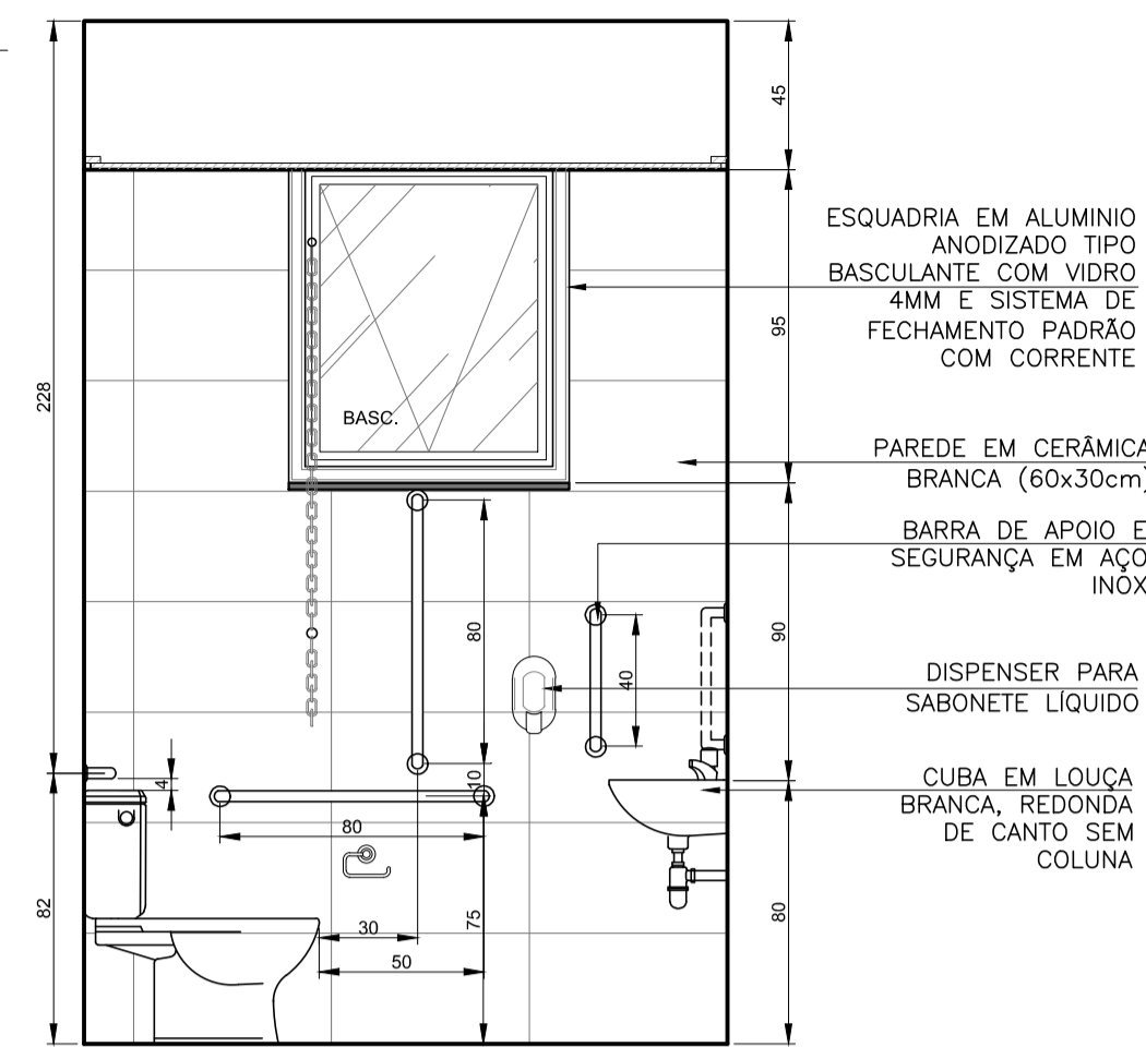
VISTA 02 SANIT. P.C.D. S/BANHO ESCALA 1:25
