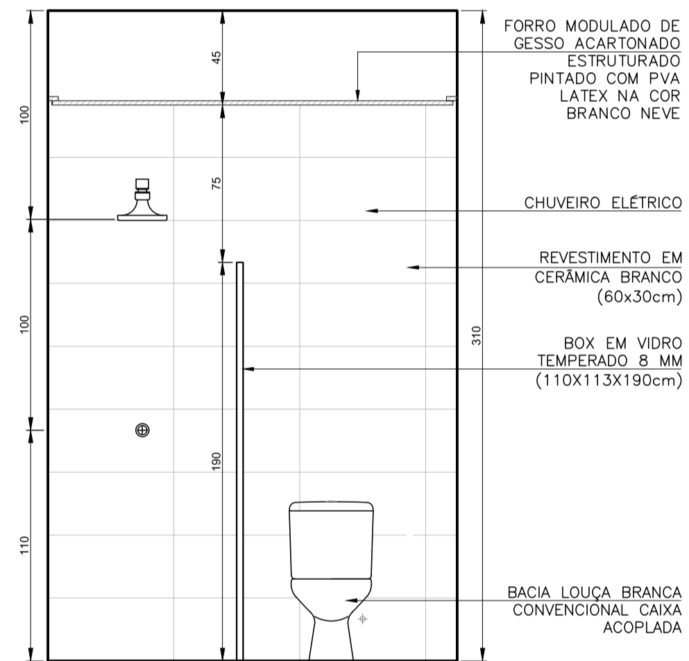
VISTA 01 I.S. FUNC.FEM/I.S. FUNC. MASC. ESCALA 1:25
