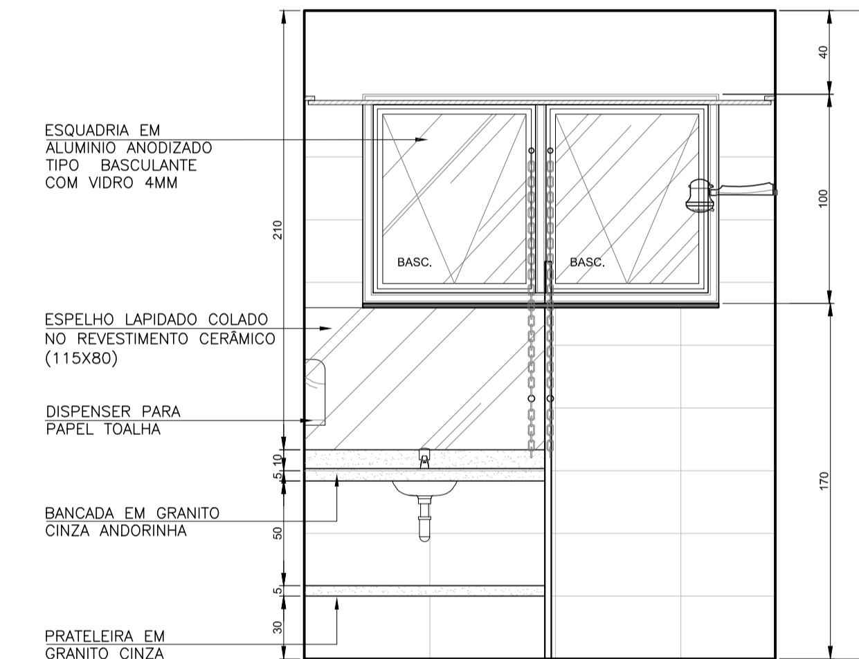
VISTA 02 I.S. FUNC.FEM/I.S. FUNC. MASC. ESCALA 1:25
