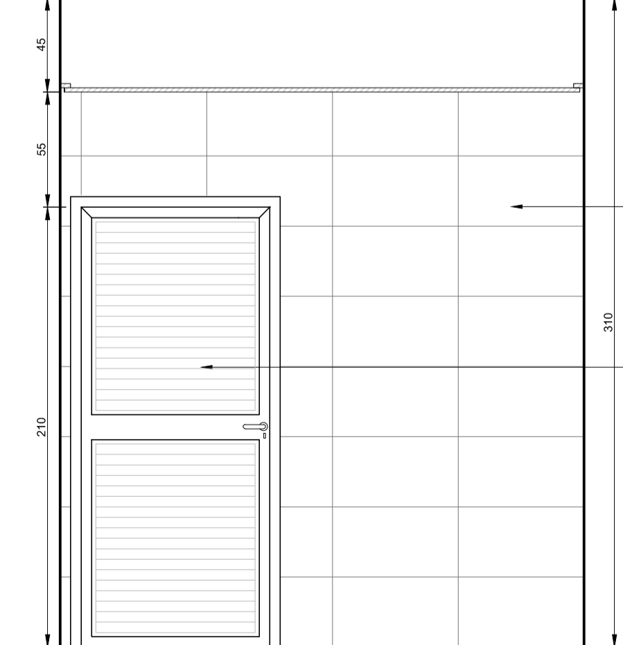
VISTA 03 DML 1º PAVIMENTO ESCALA 1:25
