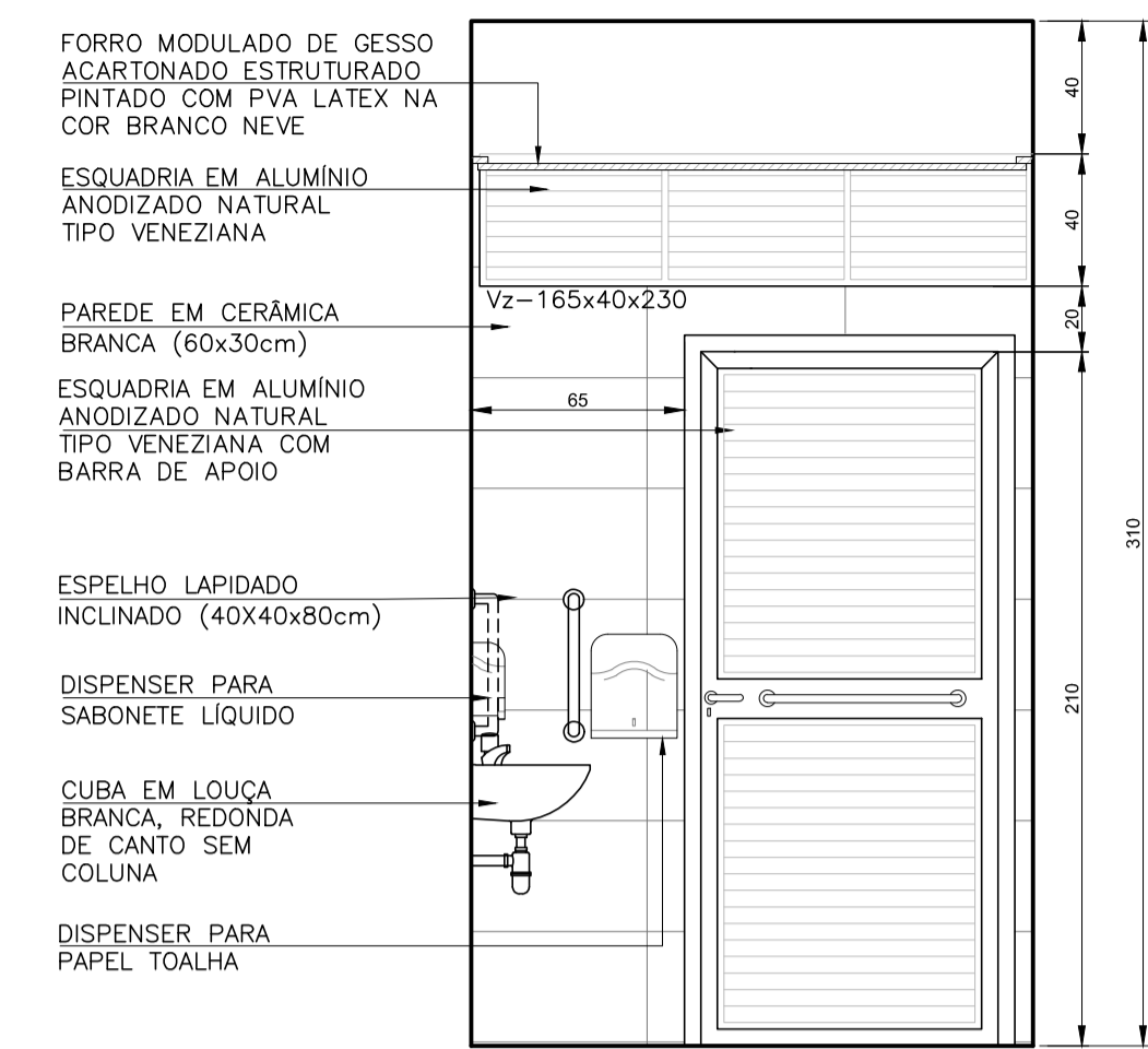
VISTA 03 SANIT. P.C.D. S/BANHO ESCALA 1:25
