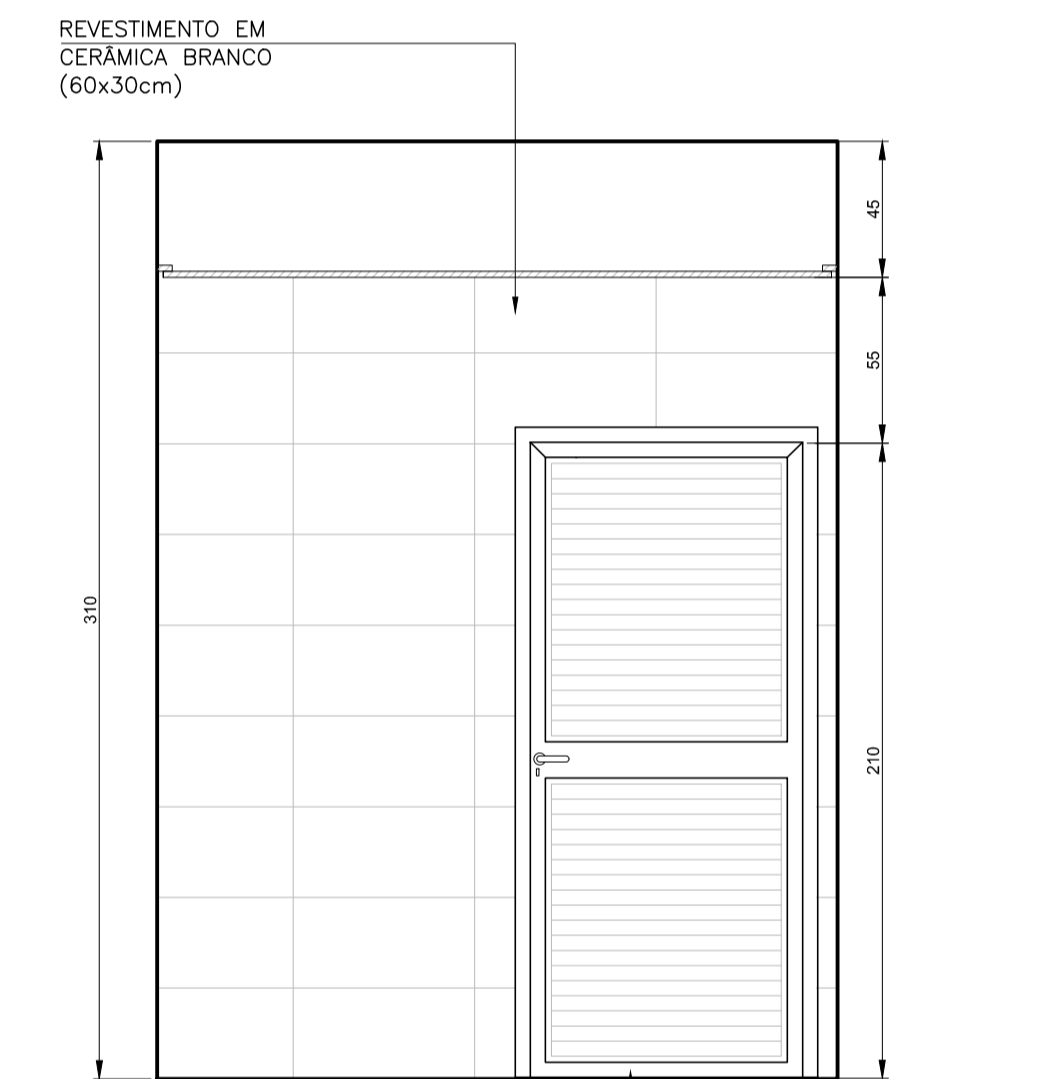
VISTA 03 I.S. FUNC.FEM/I.S. FUNC. MASC. ESCALA 1:25
