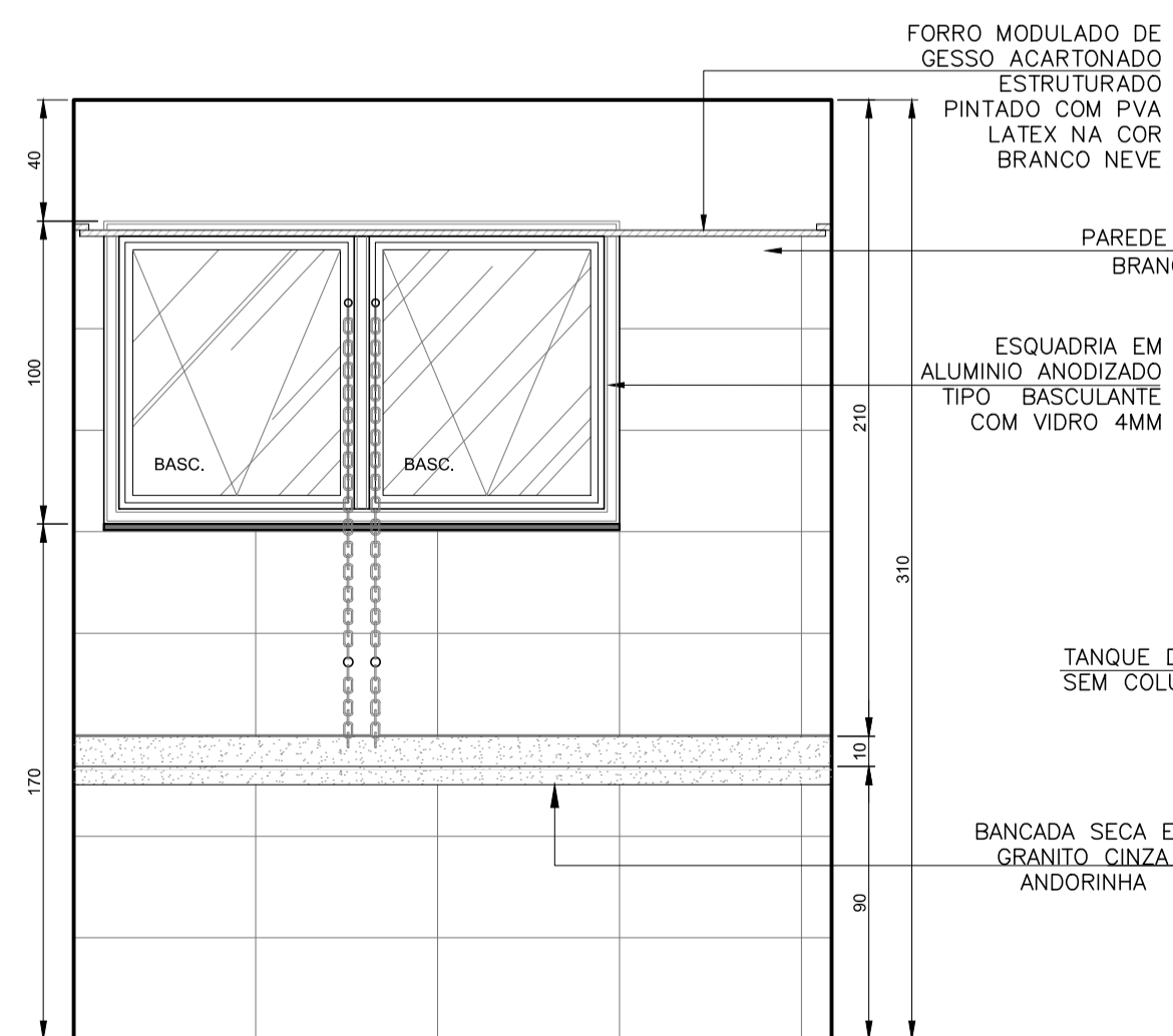
VISTA 01 DML 1º PAVIMENTO ESCALA 1:25
