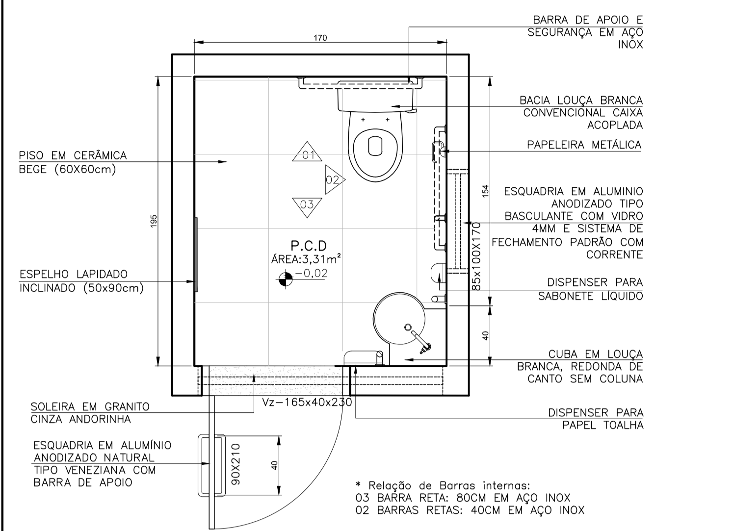
PLANTA LAYOUT SANIT. P.C.D. S/BANHO ESCALA 1:25
