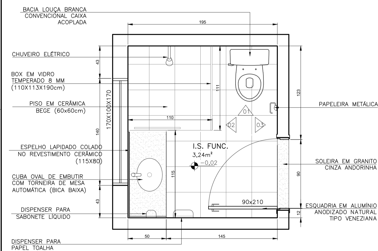
PLANTA LAYOUT I.S. FUNC.FEM/I.S. FUNC. MASC. ESCALA 1:25
