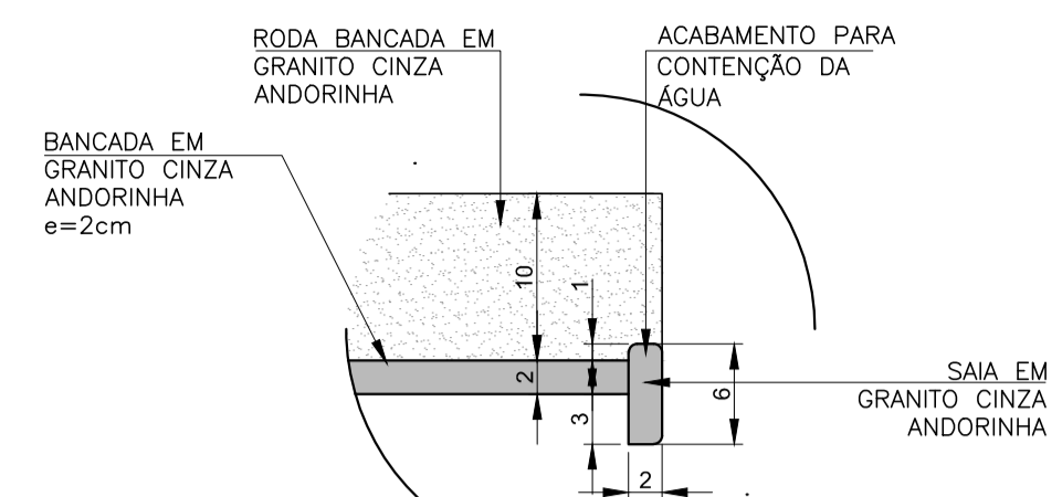
BANCADA DE GRANITO ÁREA MOLHADA esc.: 1/5
