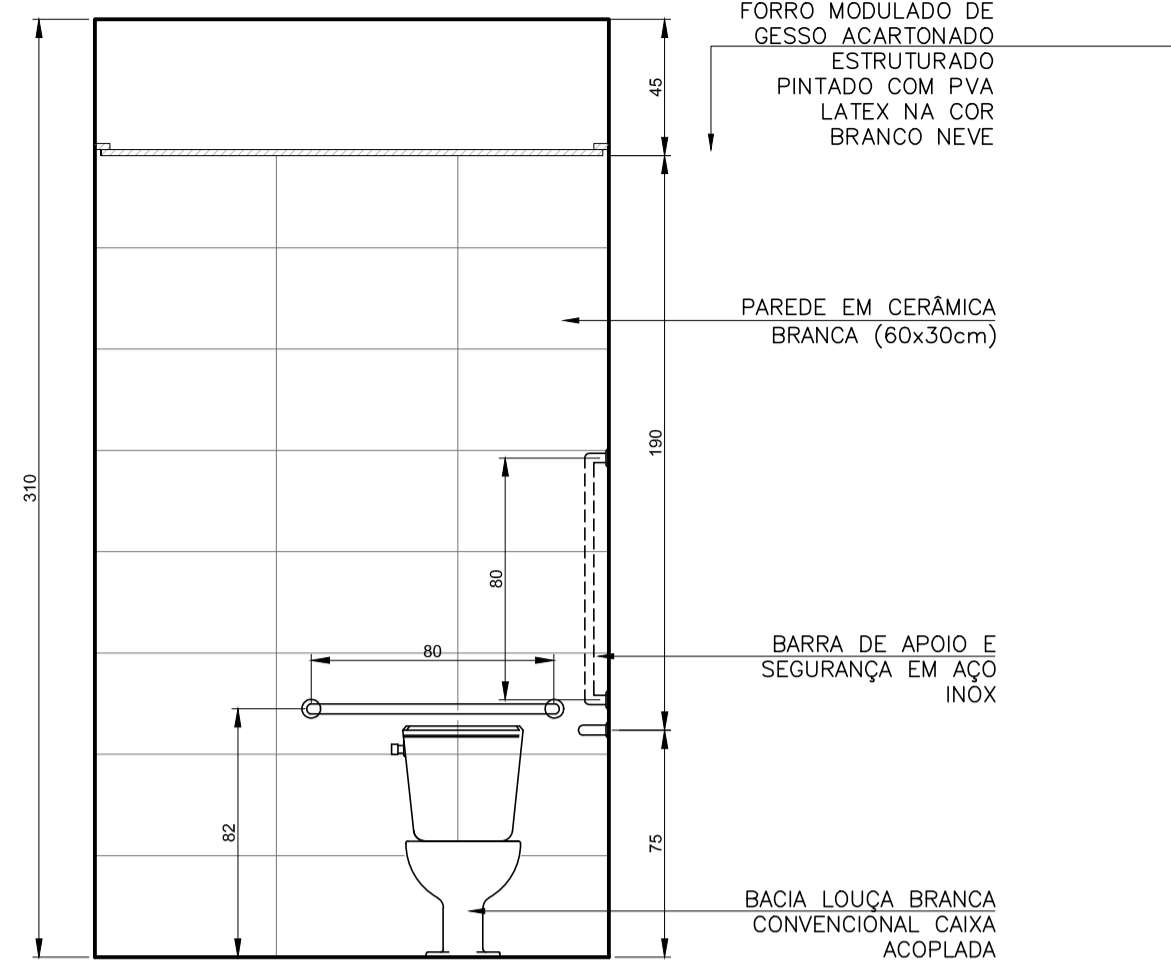
VISTA 01 SANIT. P.C.D. S/BANHO ESCALA 1:25
