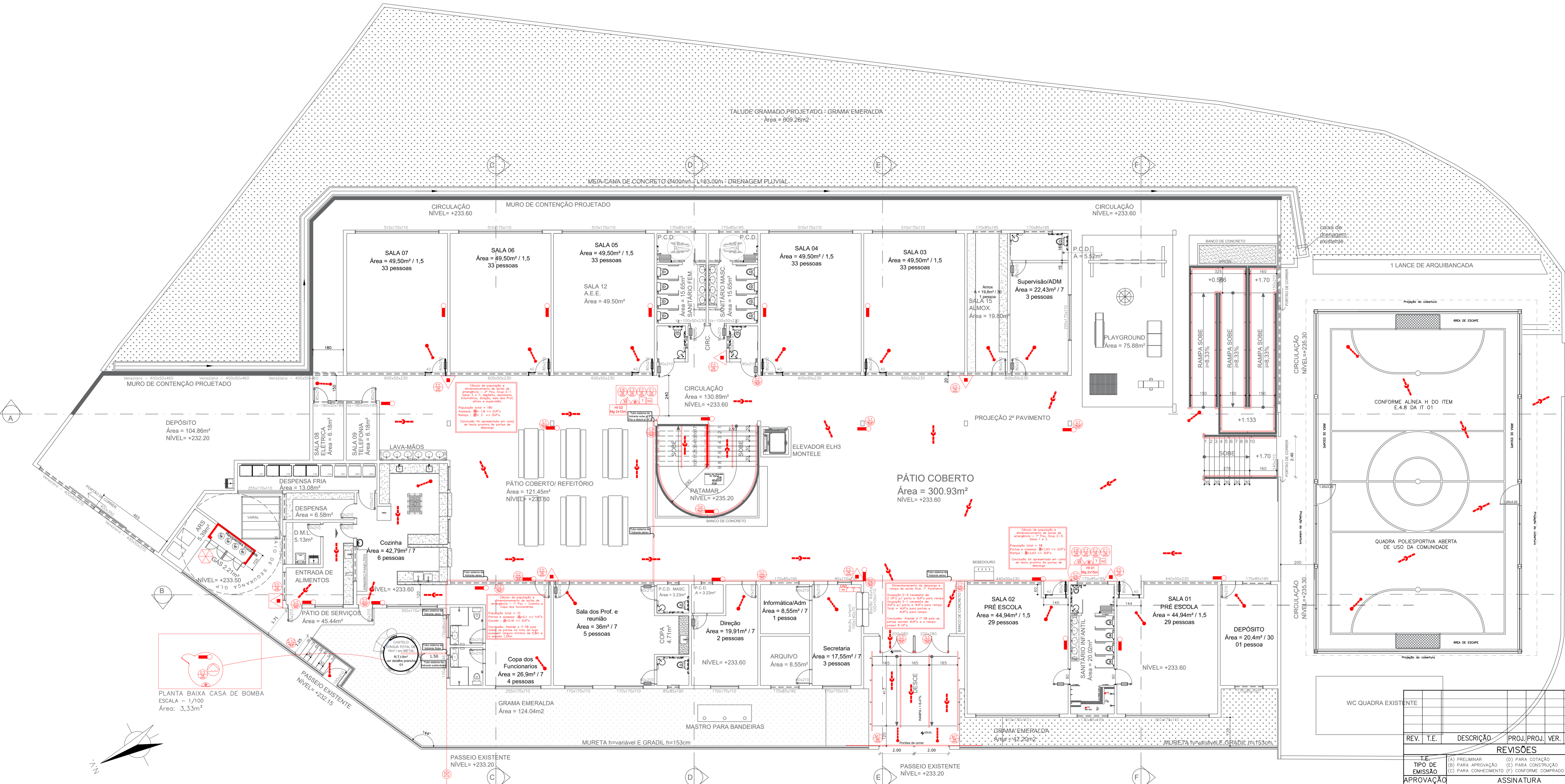
PLANTA BAIXA DO 1º PAVIMENTO ESCALA - 1/100 Área: 1535,43m 2 (1509,24 + 26,19)
